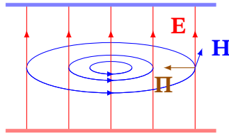
Рис. 13.8. Поля E , H і вектор Пойнтінга \Pi при зарядці плоского конденсатора
