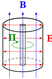
Рис. 14.9. Циліндричний конденсатор в аксіальному магнітному полі: поля \mathbf{E} , \mathbf{B} і вектор Пойнтінга \mathbf{\Pi} , що циркулює навколо осі
