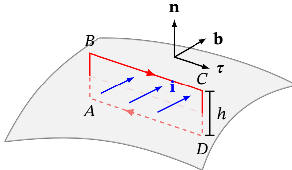
Рис. 11.8. Контур циркуляції на межі розділу двох магнетиків
