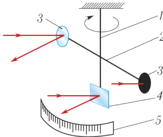
Рис. 14.6. Схема досліду П. М. Лебедева (1899) з вимірювання тиску світла
