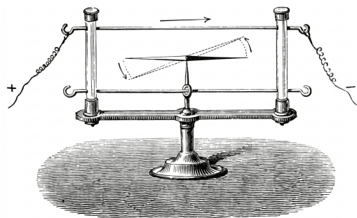
Рис. 10.1. Установка Ерстеда
