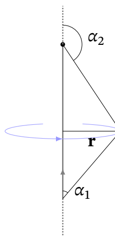
Рис. 10.7. Геометрія задачі про поле скінченного відрізка провідника
