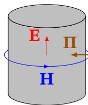
Рис. 13.9. Поля E , H і вектор Пойнтінга \Pi на поверхні довгого провідника зі струмом
