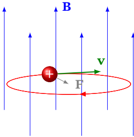
Рис. 10.5. Кругова траєкторія зарядженої частинки в однорідному магнітному полі: сила завжди перпендикулярна до швидкості
