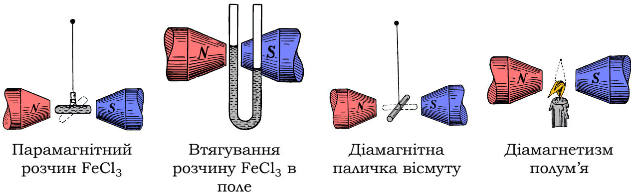
Рис. 12.21. Поведінка пара- й діамагнітних речовин у неоднорідному магнітному полі
