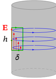
Рис. 13.12. Контур для оцінки циркуляції E поблизу поверхні провідника
