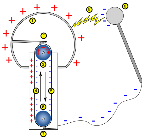
Рис. 4.7. Генератор Ван-де-Граафа
