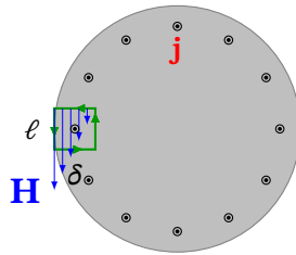
Рис. 13.13. Контур для оцінки циркуляції H на перерізі провідника
