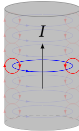
Рис. 13.11. Якісний механізм скін-ефекту: вихрові струми Фуко підсилюють струм на поверхні й послаблюють у центрі провідника
