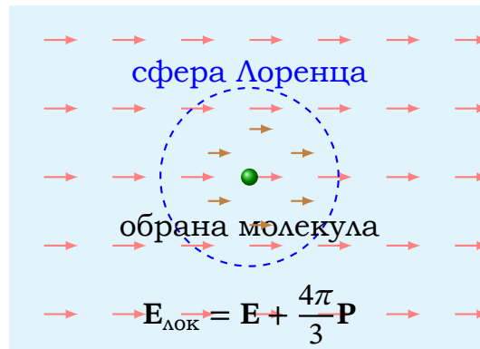
Рис. 6.2. Сфера Лоренца: локальне поле в центрі складається з середнього поля E , поправки +\frac{4\pi}{3}P (за вирізаний об'єм) і поля дискретних сусідів (для кубічної симетрії — нуль)
