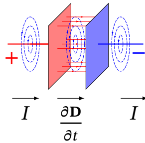
Рис. 13.5. Магнітне поле, створене струмом зміщення всередині конденсатора під час його зарядки
