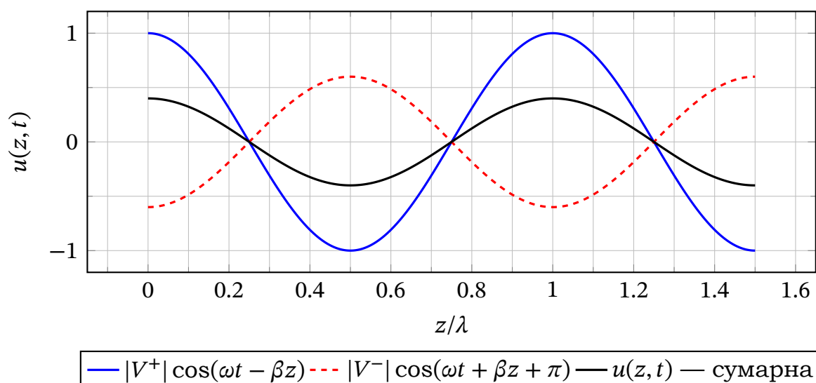
Рис. 19.2. Інтерференція падаючої та відбитої хвиль у лінії без втрат при |V^-|/|V^+| = 0.6 . Амплітуда сумарної напруги має максимуми й мінімуми (стояча хвиля). Коефіцієнт стоячої хвилі КСХ = (1 + 0.6)/(1 - 0.6) = 4 .
