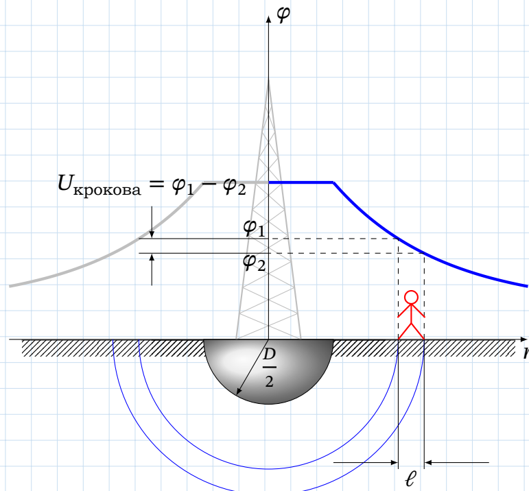
Рис. 7.13. Розтікання струму від напівсферичного заземлювача та крокова напруга
