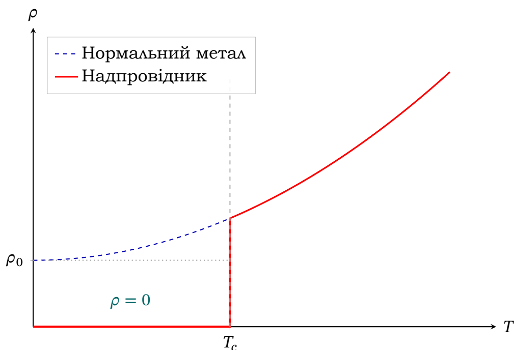
Рис. 8.3. Характерна залежність питомого опору від температури металу, який переходить в надпровідний: при високих T — майже лінійне зростання, T < T_c опір стрибкоподібно падає до нуля
