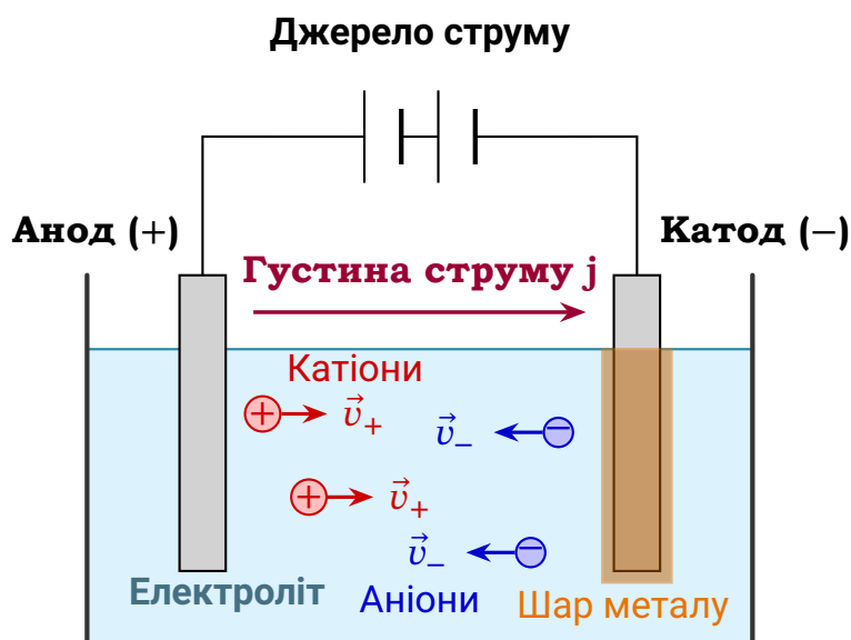
Рис. 8.5. Електроліз: рух йонів у розчині й осадження речовини на катоді
