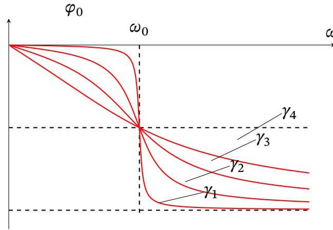
Рис. 18.6. Фазово-частотна характеристика контуру. Залежність фазового зсуву \varphi_0 від частоти \omega зовнішньої ЕРС.
