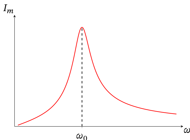
Рис. 18.9. Залежність амплітуди коливань струму від частоти коливань ЕРС — резонанс напруги на конденсаторі і ЕРС в послідовному LCR-контурі (рис. 18.1).
