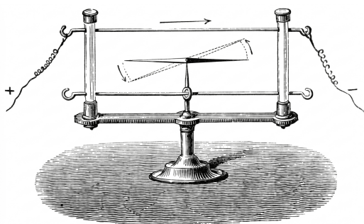
Рис. 9.1. Установка Ерстеда
