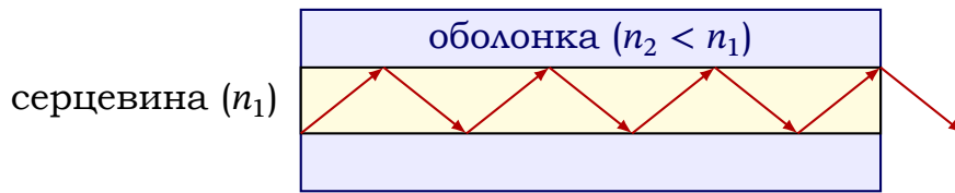
Рис. 20.3. Поширення світла в оптичному волокні завдяки повному внутрішньому відбиттю на межі серцевина-оболонка: промінь «замкнений» усередині серцевини й рухається вздовж волокна майже без втрат.
