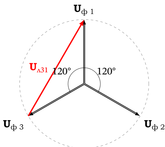
Рис. 18.22. Векторна діаграма співвідношення фазних та лінійних напруг
