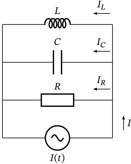
Рис. 18.10. Паралельний LCR -контур, що включає джерело заданого змінного струму I(t) = I_m \cos \omega t .
