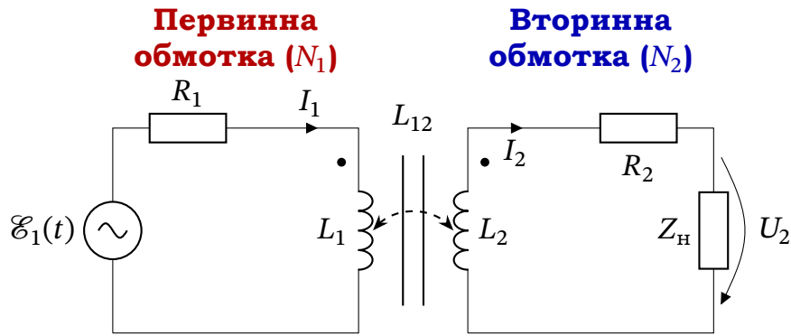
Рис. 18.13. Еквівалентна схема реального трансформатора з котушками L_1, L_2 , крапками фазування (вказують на однакову полярність виводів), активними опорами R_1, R_2 , взаємною індуктивністю L_{12} та навантаженням Z_H .
