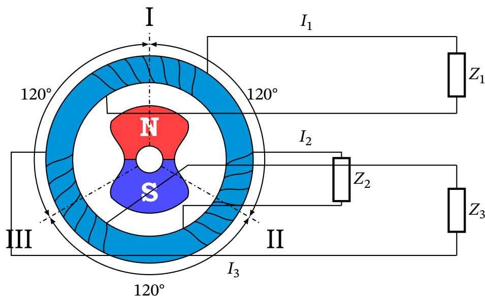
Рис. 18.19. Схематичне зображення трифазного синхронного генератора
