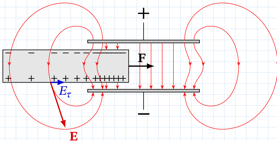
Рис. 6.7. Модель конденсатора з частково всунутою пластиною діелектрика: паралельне з'єднання вакуумного та заповненого діелектриком конденсаторів
