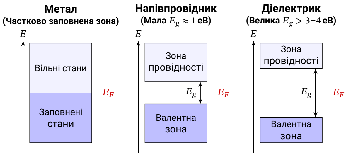
Рис. 8.13. Зонна структура металу, напівпровідника й діелектрика
