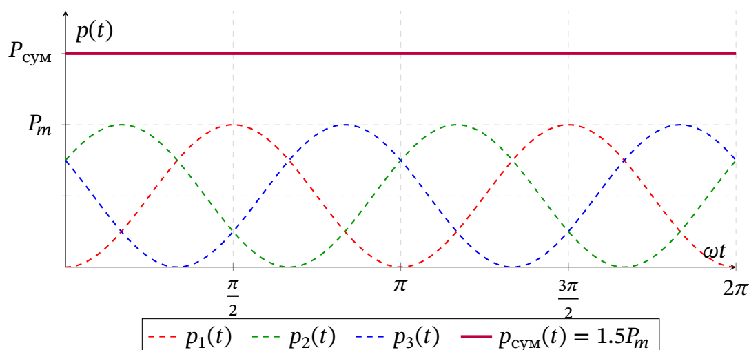
Рис. 18.24. Миттєва потужність окремих фаз та сумарна потужність трифазної системи
