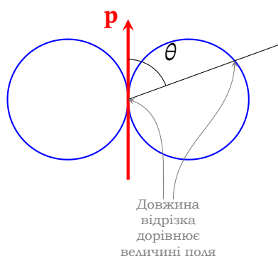
Рис. 17.8. Полярна діаграма спрямованості дипольного випромінювача: характерна форма «бублика»
