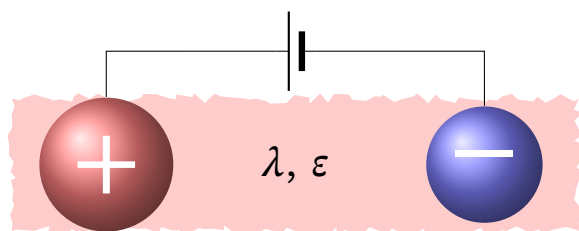
Рис. 7.12. Два електроди в необмеженому провідному середовищі з провідністю \lambda і проникністю \varepsilon
