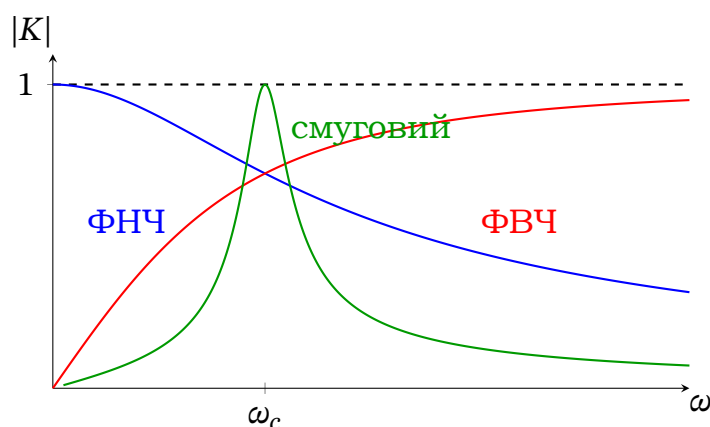
Рис. 18.18. Амплітудно-частотні характеристики трьох фільтрів: ФНЧ (синій), ФВЧ (червоний) і смугового (зелений). Для смугового прийнято Q = 5 .
