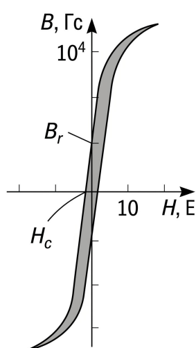
(а) Вузька петля гістерезису магнітом'якого матеріалу
