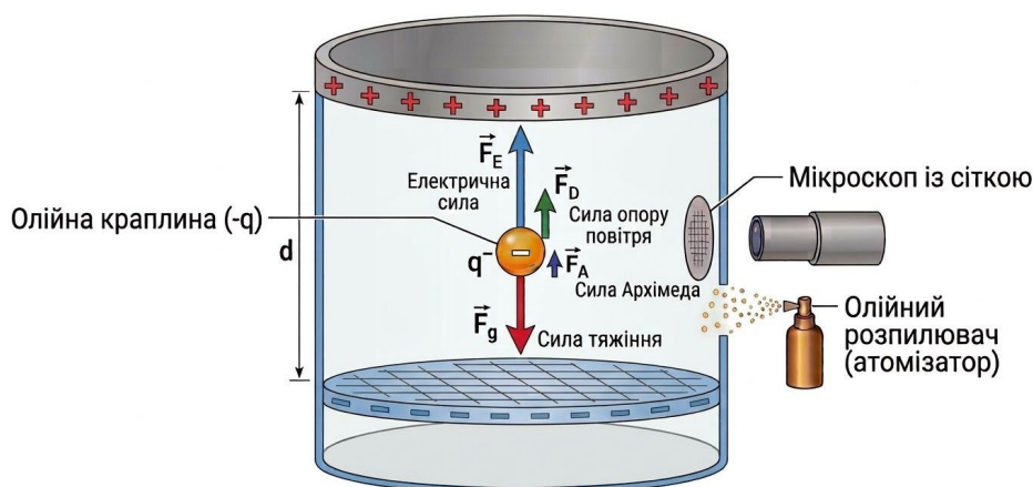
Рис. 11.9. Схема установки Міллікена для вимірювання заряду електрона (сила qE вказана для випадку q < 0 ).
