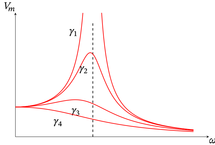
Рис. 18.5. Амплітудно-частотна характеристика контуру. Залежність амплітуди вимушених коливань V_m від частоти \omega зовнішньої ЕРС.
