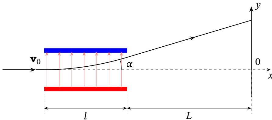
Рис. 11.7. Відхилення зарядженої частинки електричним полем конденсатора.
