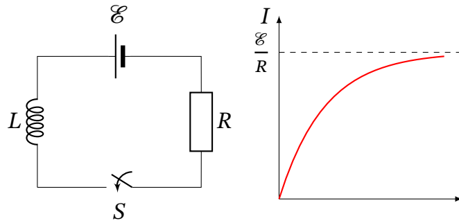
Рис. 12.10. Встановлення струму в колі з індуктивністю після замикання ключа
