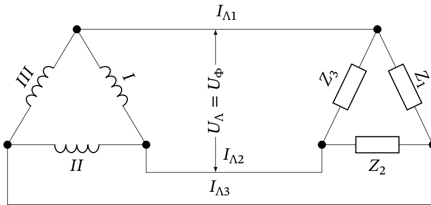
Рис. 18.23. Схема з'єднання генератора та приймача трикутником
