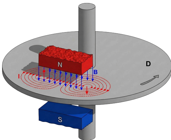
Рис. 12.7. Індукування вихрових струмів Фуко в провідному диску, що обертається в полі магніту
