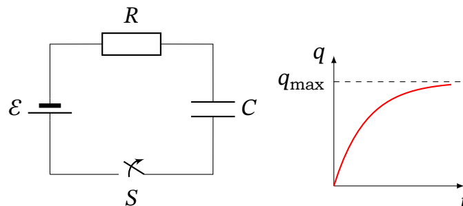
Рис. 7.15. Зарядка конденсатора від джерела ЕРС через резистор: коло та графік q(t)
