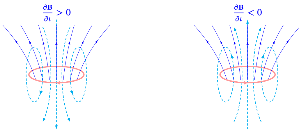
Рис. 12.6. Правило Ленца: напрям індукційного струму залежить від знака \partial \mathbf{B} / \partial t
