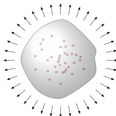
Рис. 14.6. Заряджені частинки в області, обмеженій замкнутою поверхнею: енергія електромагнітного поля може втікати й витікати крізь цю поверхню
