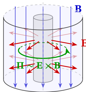
Рис. 16.8. Циліндричний конденсатор в аксіальному магнітному полі: зображено поля \mathbf{E} , \mathbf{B} і вектор Пойнтінга \mathbf{\Pi} , що циркулює навколо осі
