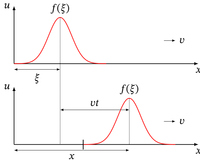
Рис. 16.2. Збурення, що поширюється без зміни форми зі швидкістю v : профіль у момент t — це профіль у момент 0, зсунутий на vt
