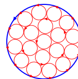
Рис. 10.3. Вигляд торця циліндра: кільцеві струми компенсуються всюди, крім бічної поверхні
