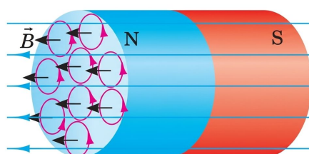
(б) Намагнічена речовина (впорядкований розподіл молекулярних струмів).
