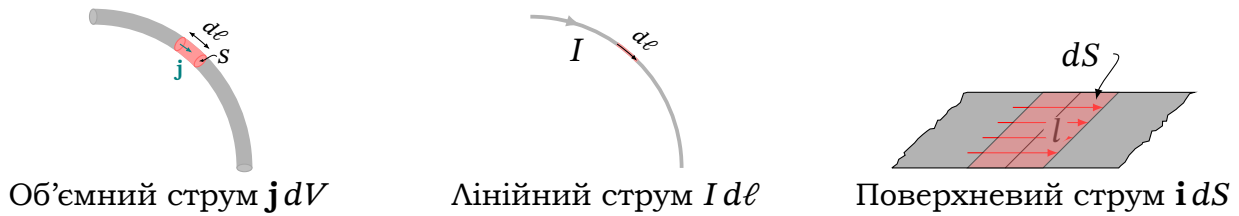
Рис. 9.4. Три еквівалентні форми запису елемента струму
