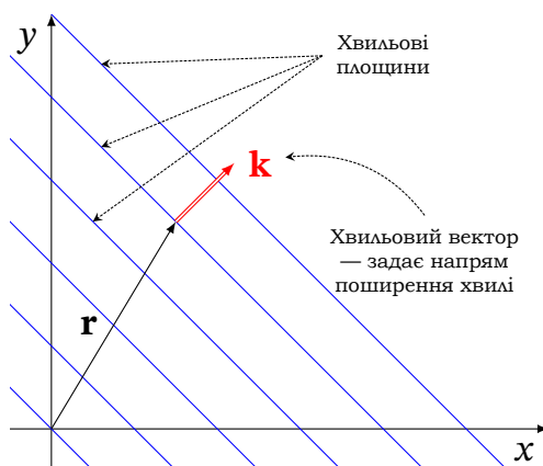
Рис. 16.3. Хвильовий вектор \mathbf{k} вказує напрям поширення плоскої хвилі й перпендикулярний до хвильових площин
