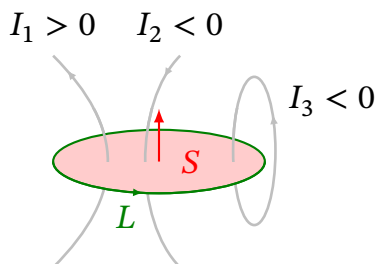
Рис. 9.10. Струм враховують зі знаком «плюс», якщо його напрям узгоджений із напрямом обходу контуру L за правилом правого гвинта, і зі знаком «мінус» — у протилежному випадку
