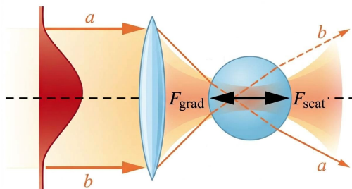
Рис. 16.7. Оптичний пінцет. Промені a і b показують заломлення світла на частинці, яке й породжує градієнтну силу
