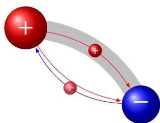
Рис. 7.8. У замкненому колі частина носіїв мусить рухатися проти сил електростатичного поля — це можливо лише завдяки стороннім силам
