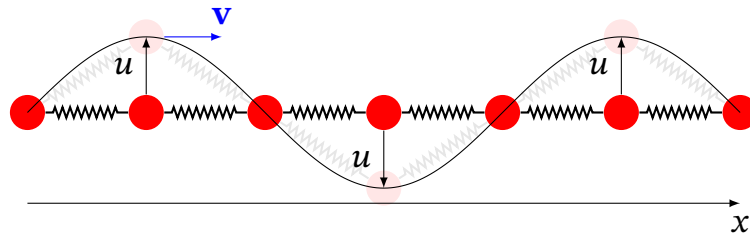
Рис. 16.1. Механічна хвиля в ланцюжку зв'язаних пружинками тягарців — наочна модель для розуміння хвильового процесу
