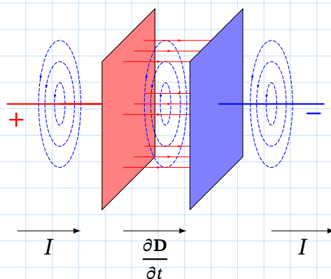
Рис. 14.3. Магнітне поле, створене струмом зміщення всередині конденсатора під час його зарядки
