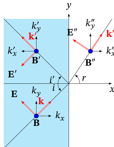
Рис. 16.10. Падаюча, відбита й заломлена p -поляризовані хвилі на межі розділу двох діелектриків
