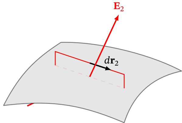
Рис. 5.9. Контур циркуляції на межі розділу двох середовищ для виведення граничної умови на тангенціальну складову \mathbf{E}
