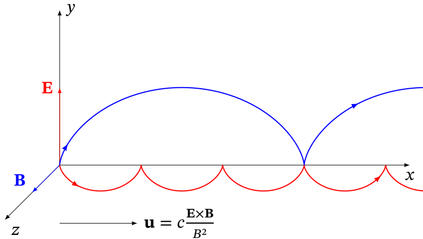
Рис. 11.4. Траєкторія частинки у взаємно перпендикулярних полях \mathbf{B} і \mathbf{E} за умови, що початкова швидкість дорівнює нулю.
