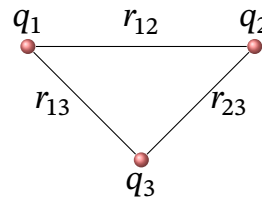
Рис. 6.4. Система трьох точкових зарядів: взаємна енергія набирається із внесків усіх пар
