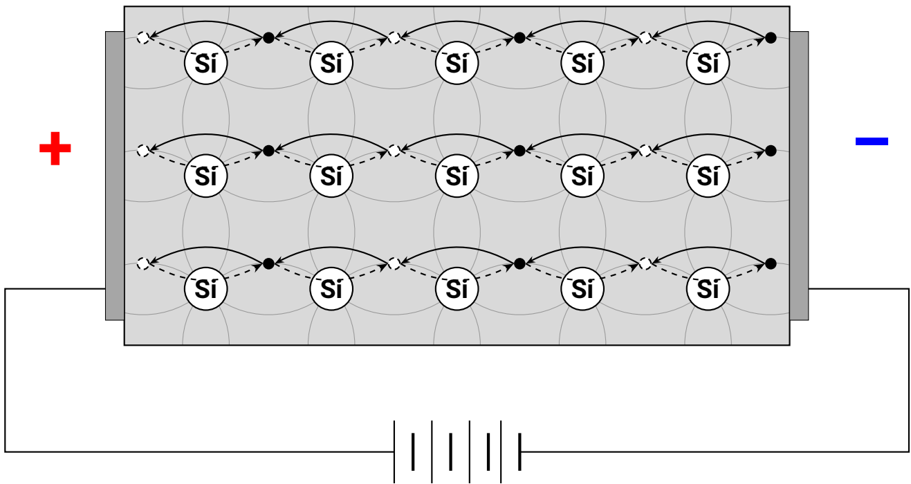
Рис. 8.14. Рух дірки як естафета електронів на сусідні вакансії. Електрони позначені чорними кружками, дірки — білими. Дірки рухаються праворуч, електрони — ліворуч.
