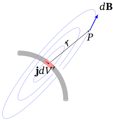
Рис. 9.6. Поле d\mathbf{B} , створюване елементом струму \mathbf{j} dV' , за законом Біо-Савара-Лапласа
