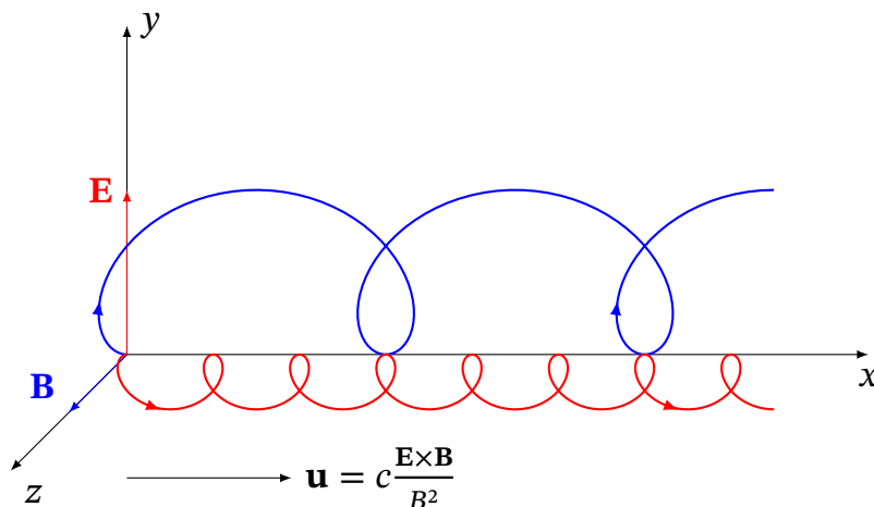
Рис. 11.3. Електричний дрейф додатно (синя крива) та від'ємно (червона крива) заряджених частинок.
