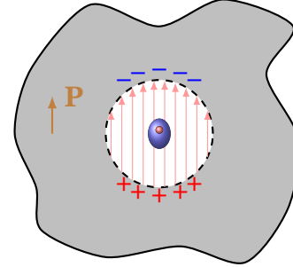
Рис. 5.11. Сферична порожнина Лоренца в поляризованому діелектрику
