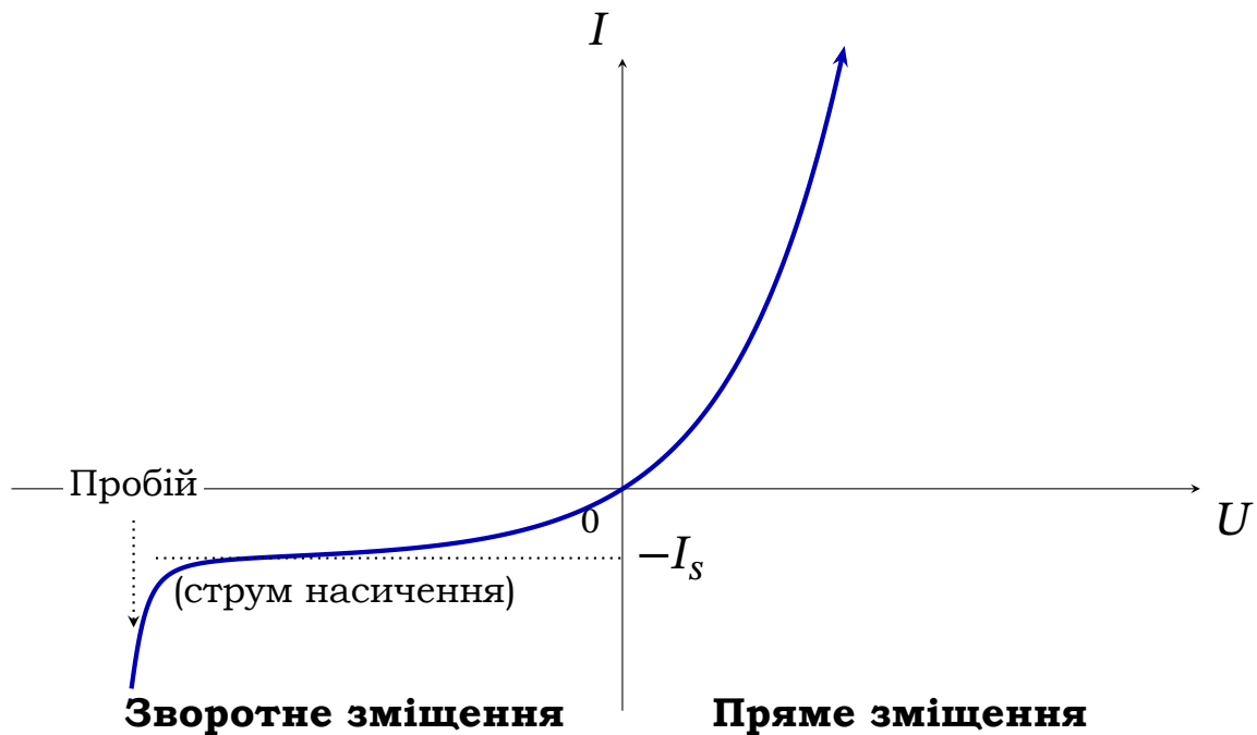
Рис. 8.16. Вольт-амперна характеристика p - n -переходу
