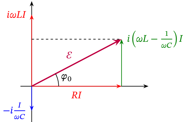
Рис. 18.8. Векторна діаграма для LCR -контур, показаного на рис. 18.1, для випадку \omega L > 1/\omega C .
