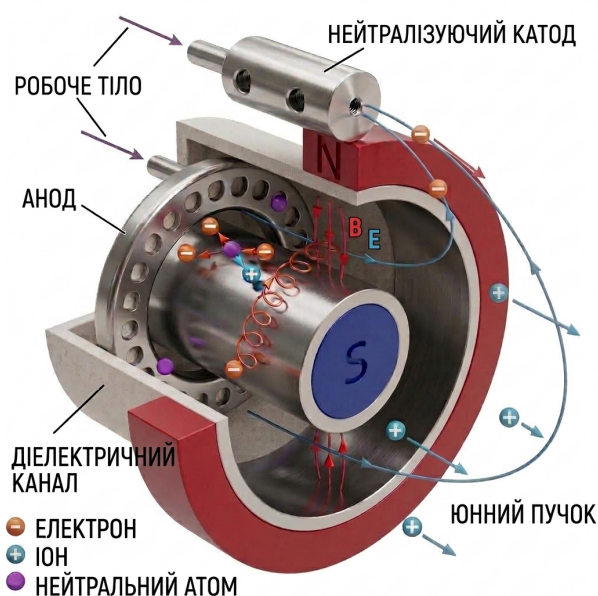
Рис. 11.6. Схема холлівського двигуна.
