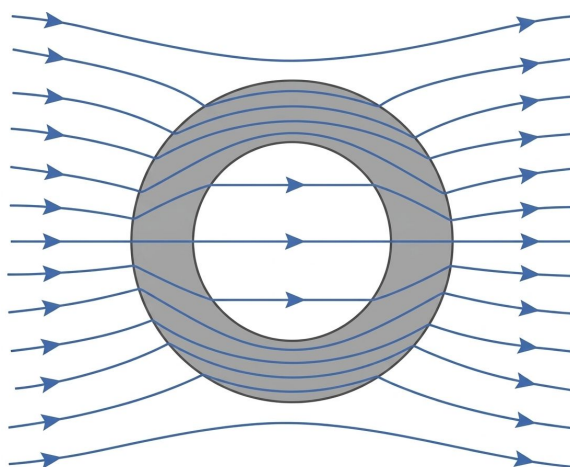
Рис. 10.8. Магнітне екранування: силові лінії концентруються в товщі. феромагнітної оболонки
