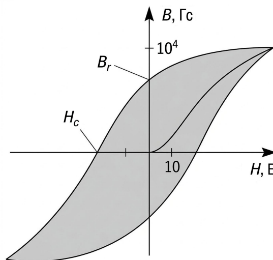
(б) Широка петля гістерезису магнітотвердого матеріалу
