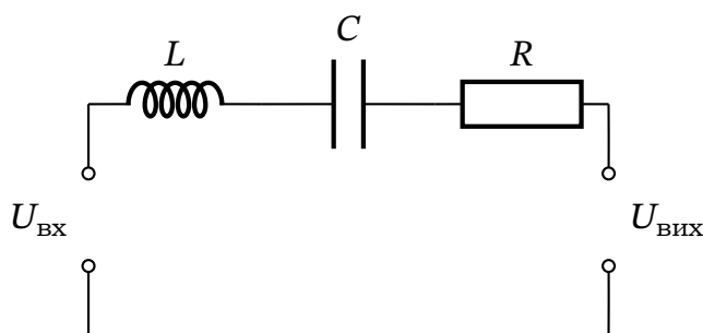
Рис. 18.17. Смуговий фільтр на основі послідовного LCR -контуру: вихідна напруга знімається з резистора R .
