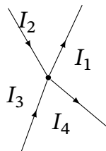
Рис. 7.10. Вузол розгалуженого кола: I_1 + I_4 = I_2 + I_3
