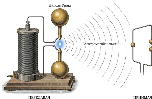
Рис. 17.1. Вібратор Герца.
