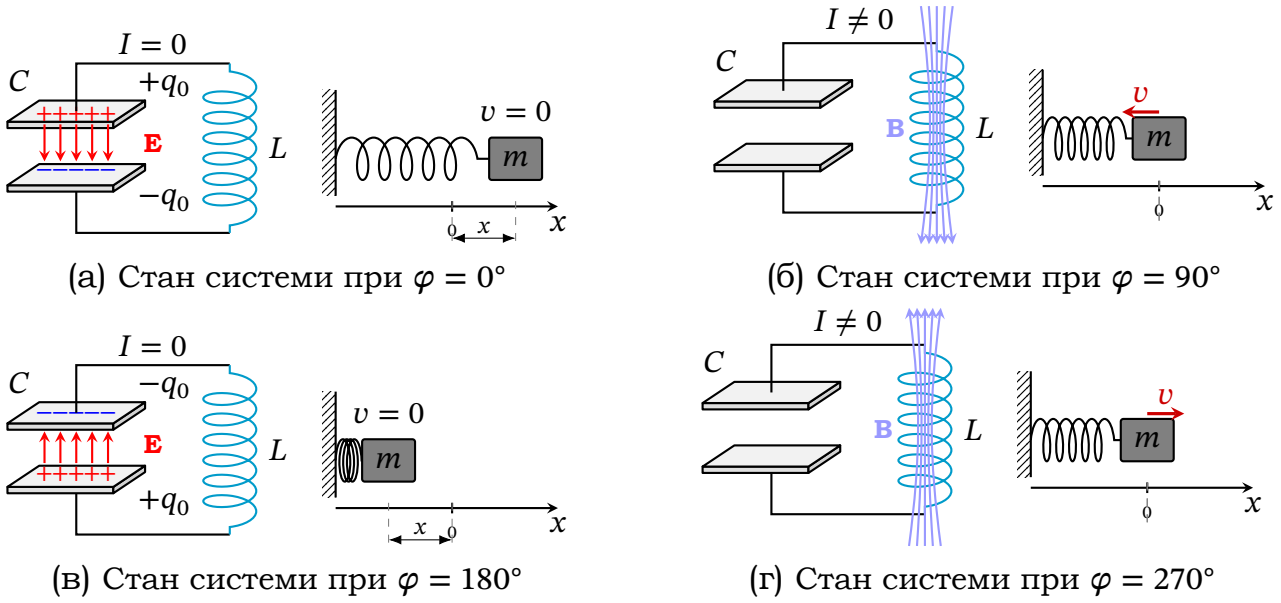
Рис. 18.2. Фази коливань електричного та магнітного полів у коливальному контурі та координати пружинного маятника
