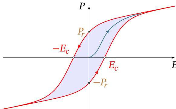
Рис. 5.14. Петля гістерезису сегнетоелектрика: P_r — залишкова поляризація, E_c — коерцитивна сила
