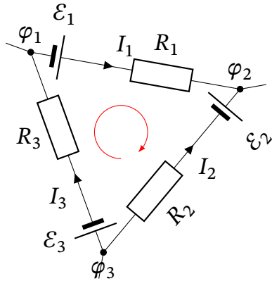
Рис. 7.11. Контур розгалуженого кола з трьома ЕРС і трьома резисторами
