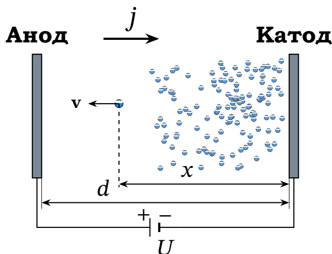
Рис. 8.11. Розподіл просторового заряду та електронів у плоскому вакуумному діоді.
