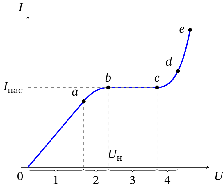
Рис. 8.6. Схематична вольт-амперна характеристика розряду в газі: омична ділянка (1), перехідна ділянка (2), струм насичення (3), лавинне зростання й пробій (4); точки a–e — характерні режими
