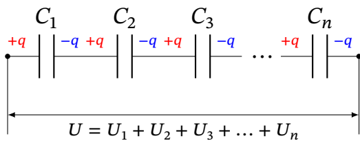
(а) Послідовне з'єднання
