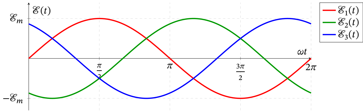
Рис. 18.20. Часові діаграми симетричної трифазної системи ЕРС
