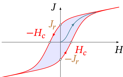
Рис. 10.11. Петля гістерезису феромагнетика: J_r — залишкова намагніченість, H_c — коерцитивна сила
