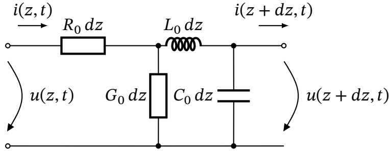
Рис. 19.1. Схема заміщення елементарного відрізка довгої лінії як чотириполосника. Паралельні елементи G_0 dz і C_0 dz рознесені для наочності.
