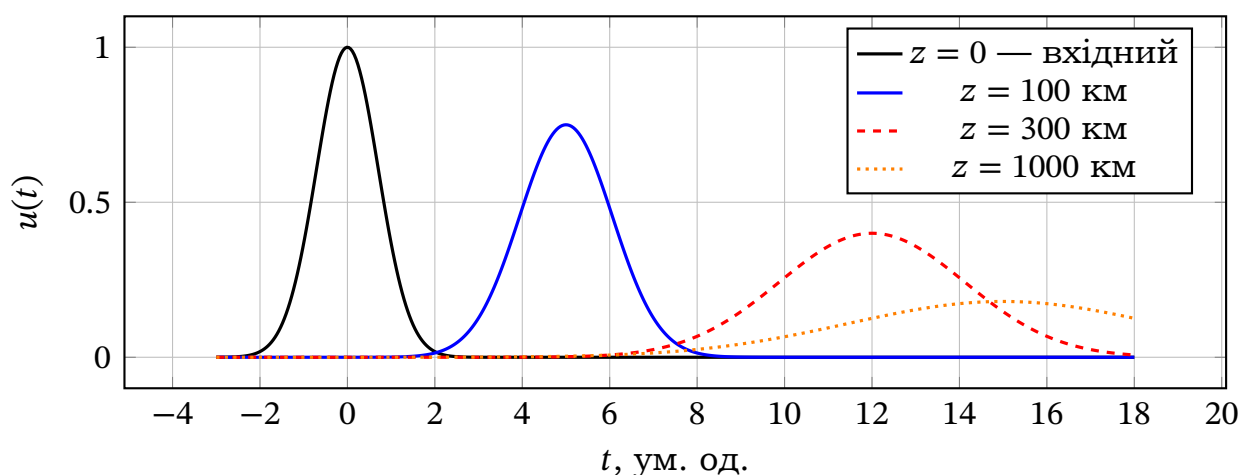
Рис. 19.3. Дисперсійне спотворення гаусового імпульсу при поширенні в лінії з втратами. З відстанню імпульс розширюється і зменшується за амплітудою — саме ця проблема мучила перші трансатлантичні кабелі.
