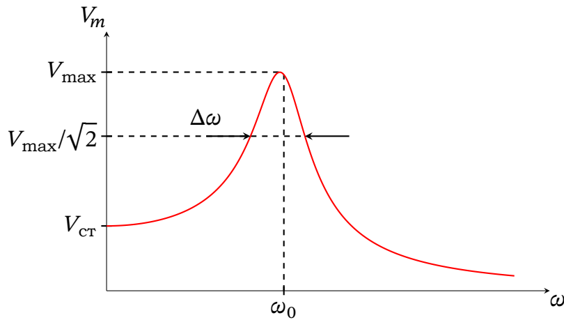
Рис. 18.7. Характеристики резонансної кривої: V_{\max} — максимум амплітуди, V_{\text{ст}} — статична амплітуда, \Delta\omega — ширина резонансу.
