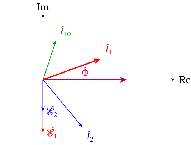
Рис. 18.14. Векторна діаграма трансформатора в режимі навантаження. Потік \hat{\Phi} напрямлений уздовж дійсної осі; ЕРС відстають від нього на \pi/2 ; струм \hat{I}_1 є сумою струму холостого ходу та скомпенсованого вторинного струму.
