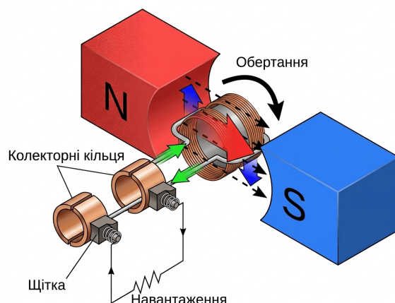
Рис. 12.4. Схема найпростішого генератора змінного струму
