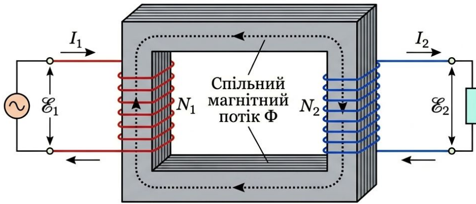
Рис. 13.6. Принципова схема трансформатора
