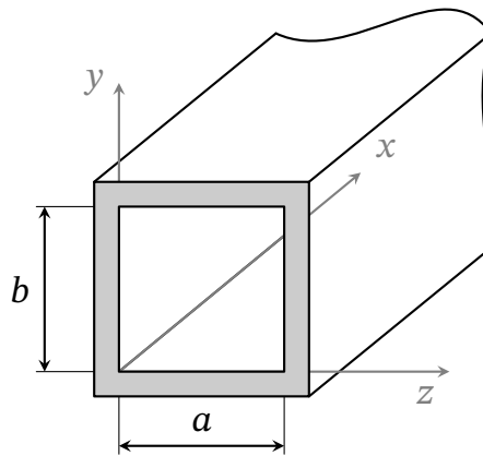
Рис. 20.1. Прямокутний хвильовід
