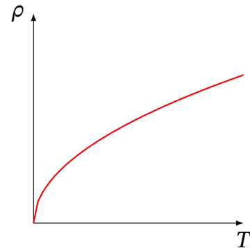
Рис. 8.1. Передбачення найпростішої теорії Друде: \rho \propto \sqrt{T}
