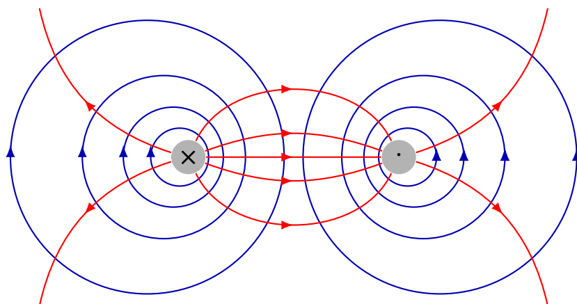
Рис. 19.4. Лінії електричного (червоні) та магнітного (сині) полів для біжучої хвилі в перерізі двопровідної лінії
