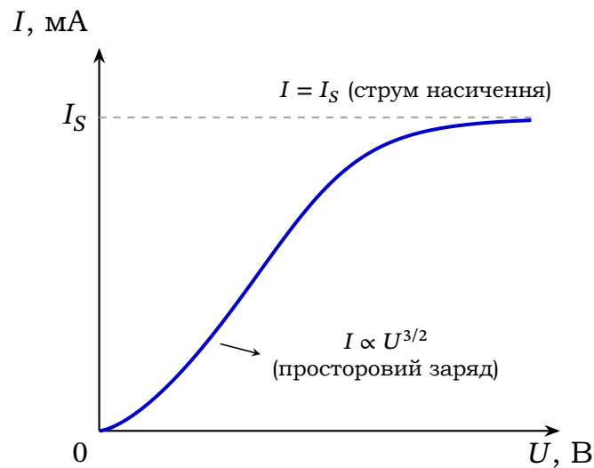
Рис. 8.12. Вольт-амперна характеристика вакуумного діода
