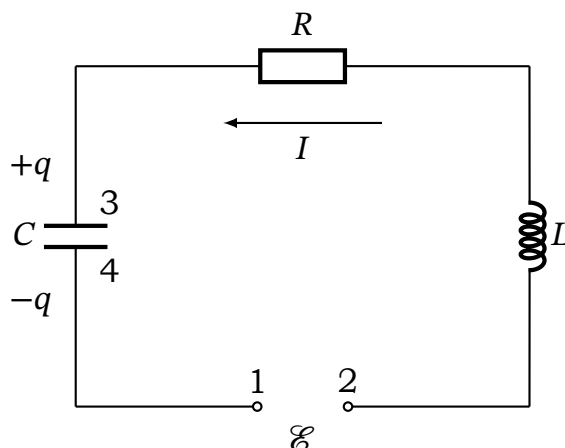
Рис. 18.1. Контур, що включає конденсатор, індуктивність, опір R і стороннє джерело ЕРС \mathcal{E} .
