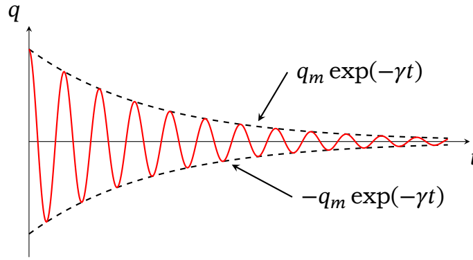
Рис. 18.3. Графік затухаючих коливань. Штриховою лінією показано часову залежність амплітуди A(t) = q_m e^{-\gamma t} .
