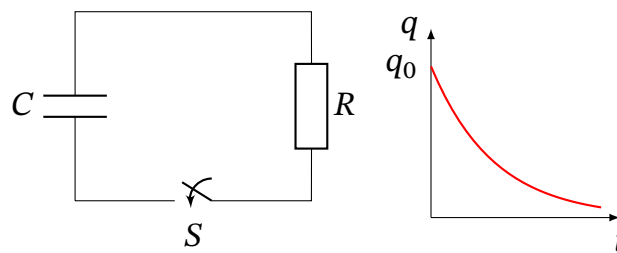
Рис. 7.14. Розрядка конденсатора через резистор: коло та графік q(t)
