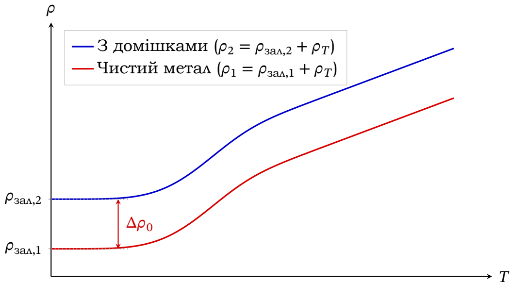
Рис. 8.2. Правило Маттіссена: домішки додають до опору сталу \rho_{\text{зал}} , не змінюючи температурної частини
