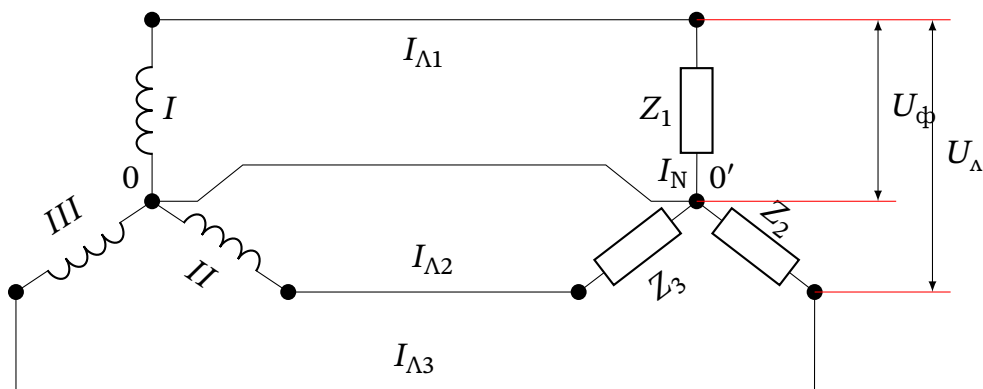
Рис. 18.21. З'єднання трифазної системи зіркою з нейтральним проводом
