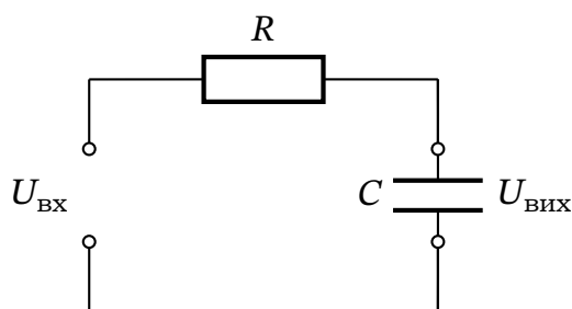
Рис. 18.15. Фільтр низьких частот: вихідна напруга знімається з конденсатора C.
