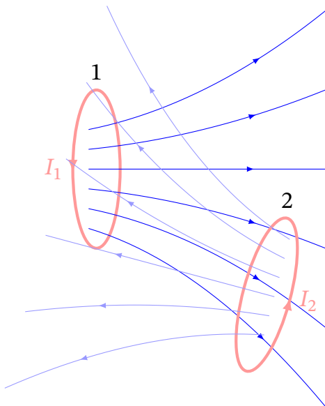
Рис. 13.2. Два нерухомі контури, магнітно пов'язані один з одним
