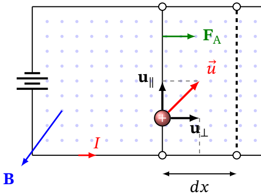
Рис. 12.2. Рамка з рухомою перемичкою в магнітному полі: показано силу Ампера F_A , що діє на перемичку зі струмом I , зміщення dx та розклад повної швидкості \mathbf{u} носія заряду на складові \mathbf{u}_\perp (рух разом із перемичкою) і \mathbf{u}_\parallel (рух уздовж провідника)
