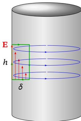
Рис. 14.9. Контур для оцінки циркуляції E поблизу поверхні циліндричного провідника (вигляд збоку)
