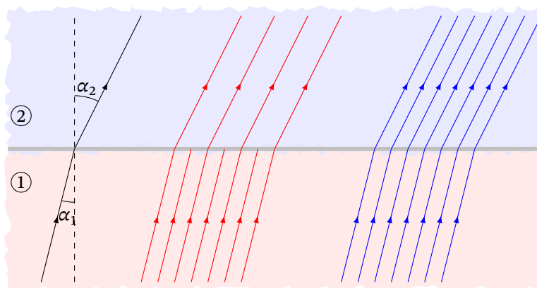
Поле вектора \mathbf{E} Поле вектора \mathbf{D}
