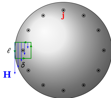
Рис. 14.10. Контур для оцінки циркуляції H поблизу циліндричного поверхні провідника (вигляд зверху)
