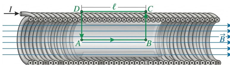
Рис. 9.11. До розрахунку магнітного поля нескінченно довгого соленоїда.
