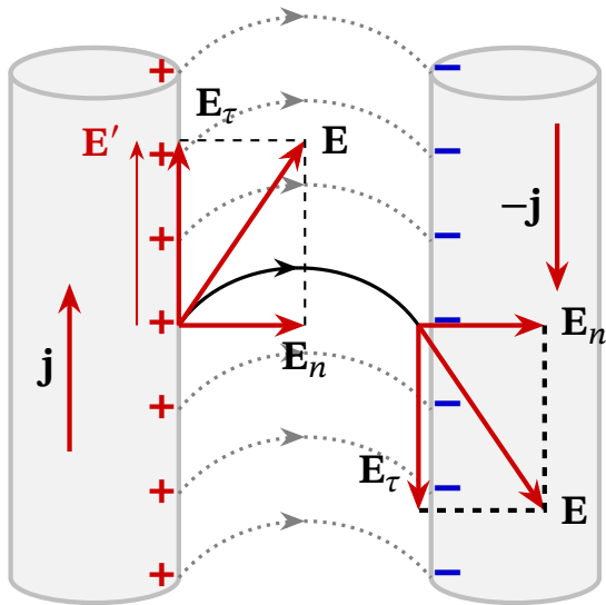
Рис. 7.6. Поверхневі заряди на провіднику зі струмом створюють як тангенціальну, так і нормальну складову поля
