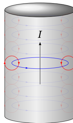
Рис. 14.8. Якісний механізм скін-ефекту: вихрові струми Фуко підсилюють струм на поверхні й послаблюють у центрі провідника
