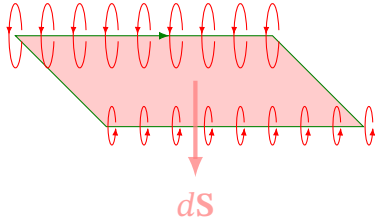
Рис. 10.4. Довільний замкнений контур L у намагніченій речовині
