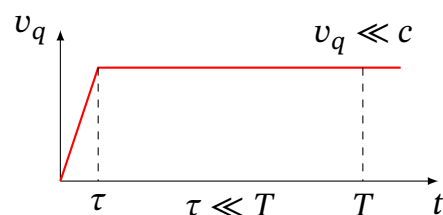
Рис. 17.2. Швидкість заряду: короткий імпульс прискорення тривалістю \tau , після якого заряд рухається рівномірно
