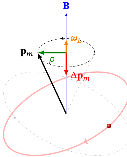
Рис. 10.9. Прецесія орбіти електрона в зовнішньому полі B : магнітний момент \mathbf{p}_m (а разом з ним і площина орбіти) обертається навколо B з ларморовою частотою \omega_L . Ця прецесія еквівалентна додатковому коловому струму I = -e\omega_L/(2\pi) , який створює індукований магнітний момент \Delta\mathbf{p} , направлений проти B .
