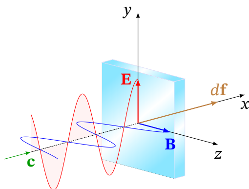
Рис. 16.5. Механізм виникнення тиску електромагнітної хвилі: сила Ампера df , що діє на струм, збуджений полем E , у полі B
