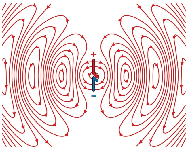
Рис. 17.7. Електричне поле осцилюючого диполя: у ближній зоні поле ніби «причеплене» до диполя, у хвильовій — випромінюється
