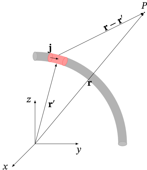
Рис. 9.8. Позначення для точки спостереження \mathbf{r} і точки джерела \mathbf{r}'
