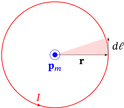
Рис. 9.13. До обчислення магнітного моменту колового витка зі струмом
