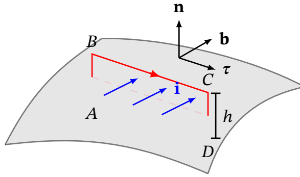
Рис. 10.6. Контур циркуляції на межі розділу двох магнетиків
