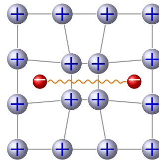
Рис. 8.4. Утворення куперівської пари через обмін фононами
