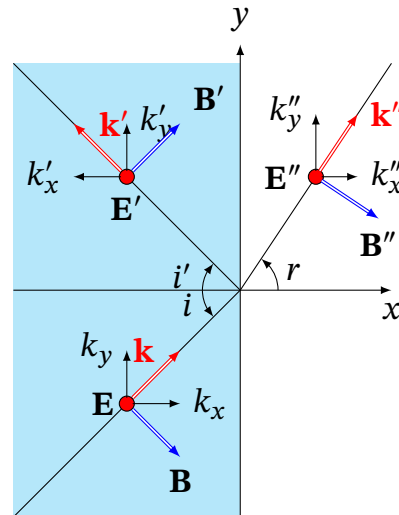
Рис. 16.9. Падаюча, відбита й заломлена s -поляризовані хвилі на межі розділу двох діелектриків
