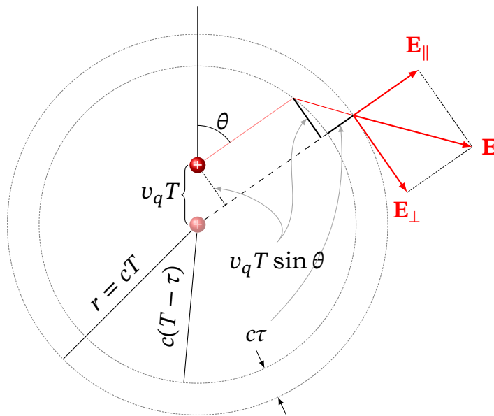
Рис. 17.4. Геометрія зламу силової лінії: розкладання поля на поздовжню E_{\parallel} і поперечну E_{\perp} складові
