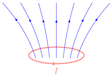
Рис. 12.9. Контур зі струмом I і створюване ним власне магнітне поле
