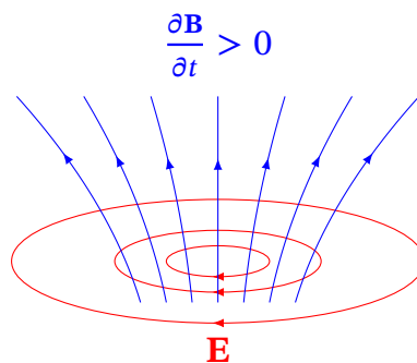
Рис. 12.8. Вихрове електричне поле, породжене зростаючим у часі магнітним полем
