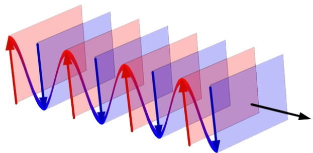
Рис. 16.3. Хвильовий вектор \mathbf{k} вказує напрям поширення плоскої хвилі й перпендикулярний до хвильових площин
