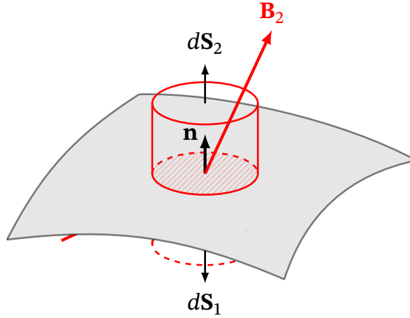
Рис. 10.5. Циліндр Гаусса на межі розділу двох магнетиків
