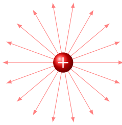
Електростатика: поле точкового заряду
