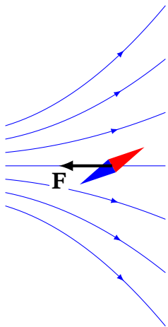
Рис. 9.16. Магнітний диполь у неоднорідному полі втягується в область сильнішого поля
