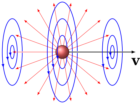
Рис. 9.2. Заряд, що рухається зі швидкістю v , є джерелом як електричного, так і магнітного поля
