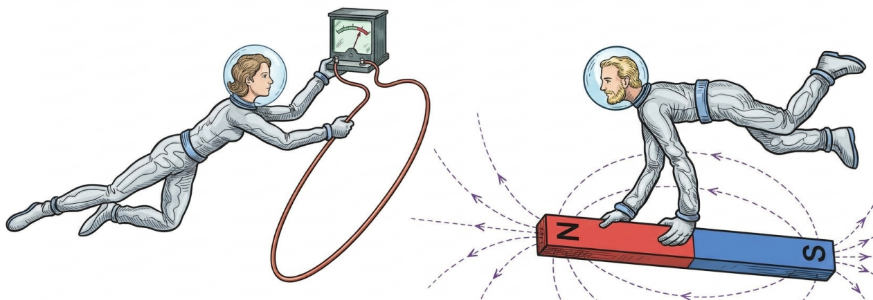
Рис. 15.1. Аліса та Боб, кожен з яких вважає нерухомим себе, по-різному пояснюють причину виникнення того самого струму в провіднику: для Аліси це електричне поле рухомого магніту, для Боба — сила Лоренца з боку магнітного поля нерухомого магніту
