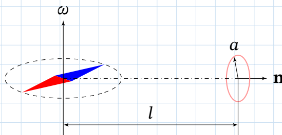
Рис. 13.5. Магнітний диполь, що обертається, і нерухоме кільце на відстані \ell
