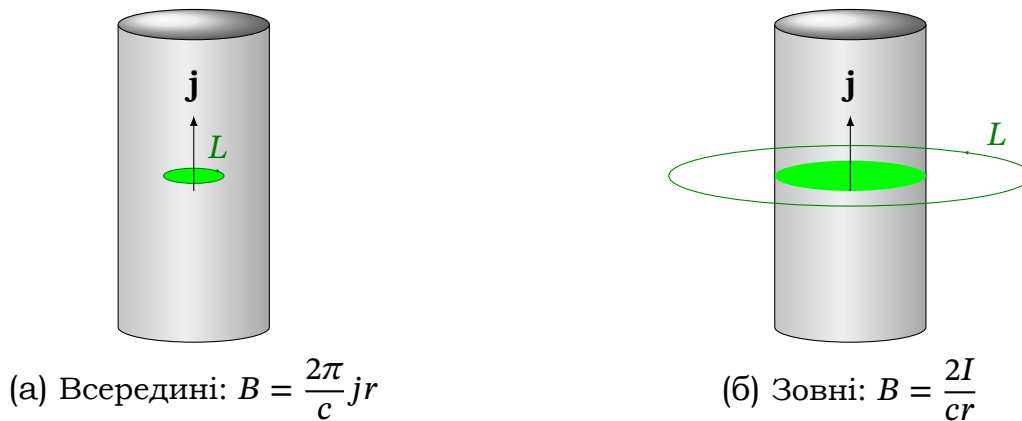
Рис. 9.12. Поле нескінченного циліндричного провідника зі струмом: усередині й поза провідником
