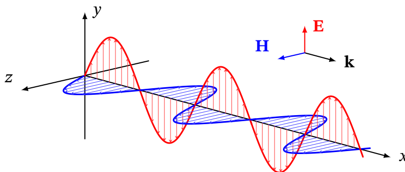
Рис. 16.4. Плоска монохроматична електромагнітна хвиля: взаємно перпендикулярні коливання \mathbf{E} і \mathbf{H} , що поширюються вздовж \mathbf{k}
