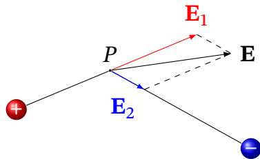
Рис. 2.3. Ілюстрація принципу суперпозиції для випадку двох різнойменних зарядів
