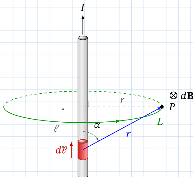
Рис. 9.7. До обчислення магнітного поля нескінченного провідника зі струмом.
