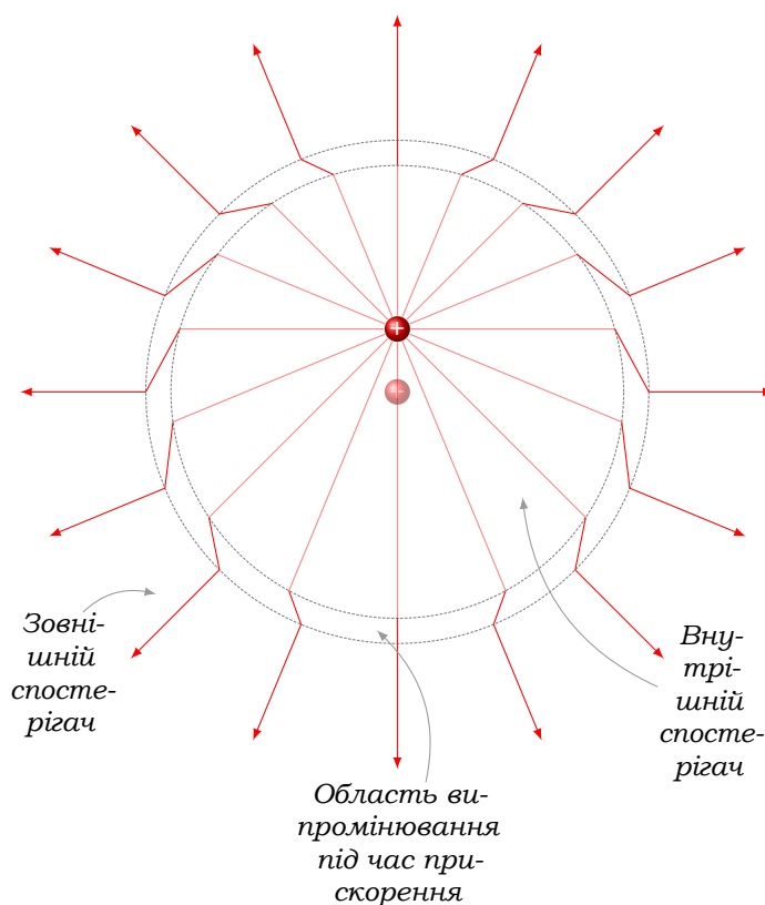
Рис. 17.3. Заломлені («злами») силові лінії поля короткочасно прискореного заряду: межа між «старим» і «новим» полем
