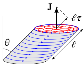
Рис. 10.2. Косокутний циліндр у намагніченій речовині
