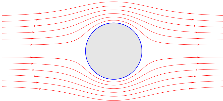
Рис. 12.13. Надпровідна куля в зовнішньому магнітному полі: силові лінії обтікають кулю, не проникаючи всередину — поле виштовхується поверхневими екрануючими струмами
