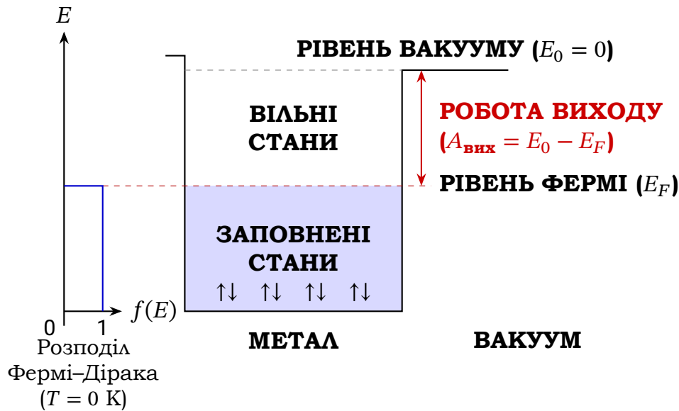
Рис. 8.9. Потенціальна яма електрона в металі: рівень Фермі, рівень вакууму, робота виходу A_{\text{вих}} ; заповнені стани електронів
