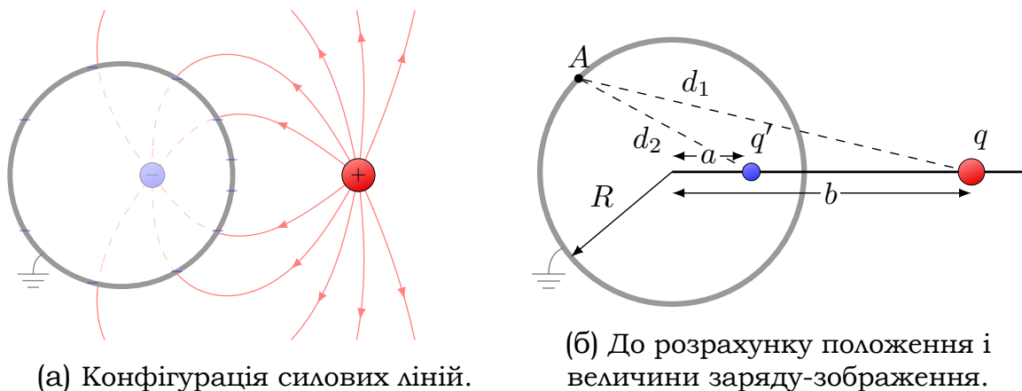
Рис. 4.15. Заряд поблизу заземленої сфери.
