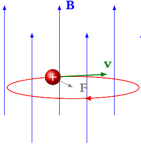
Рис. 11.1. Обертальний рух частинки із зарядом q > 0 навколо напрямку магнітного поля.
