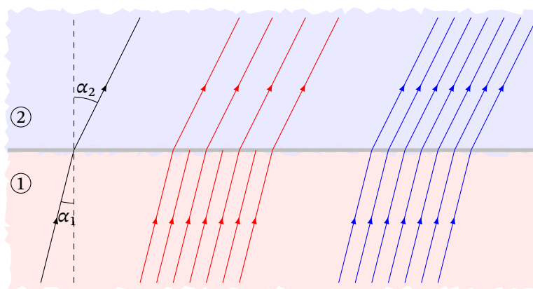
Поле вектора \mathbf{H} Поле вектора \mathbf{B}
