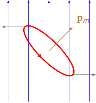
Рис. 9.15. Виток зі струмом, довільно орієнтований в однорідному полі
