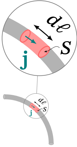
Рис. 9.3. Елемент лінійного струму I d\ell : збільшений фрагмент показує напрям \mathbf{j} уздовж осі провідника перерізу S
