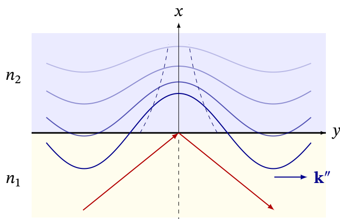
Рис. 16.12. Згасаюча хвиля в другому середовищі при i > i_b ( s -поляризація:
