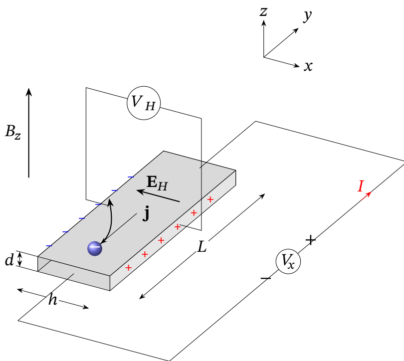
Рис. 11.5. Ефект Холла: струм \mathbf{j} уздовж пластинки, магнітне поле \mathbf{B} перпендикулярно їй; сила Лоренца відхиляє носії заряду до одного з країв, у результаті чого встановлюється поперечне холлівське поле E_H .
