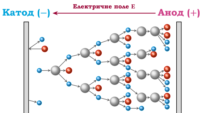
Рис. 8.7. Електронна лавина та вторинна емісія з катода
