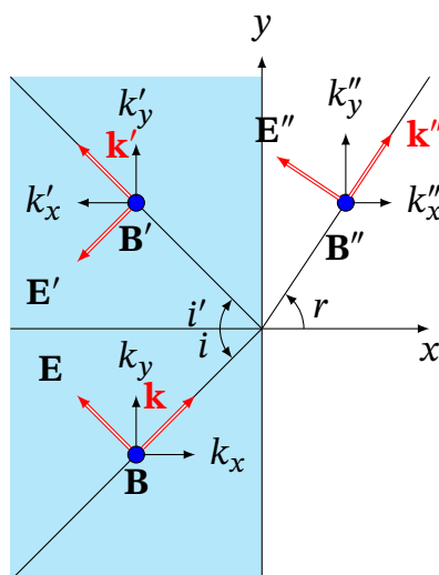
Рис. 14.11. Падаюча, відбита й заломлена r-поляризовані хвилі на межі розділу двох діелектриків
