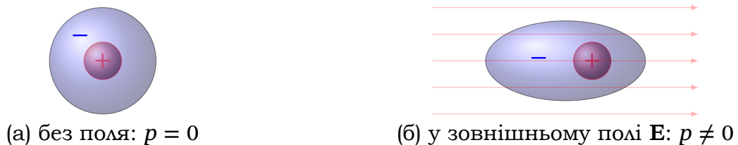
Рис. 5.2. Неполярна молекула без зовнішнього поля та в зовнішньому полі
