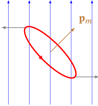
Рис. 9.15. Виток зі струмом, довільно орієнтований в однорідному полі
