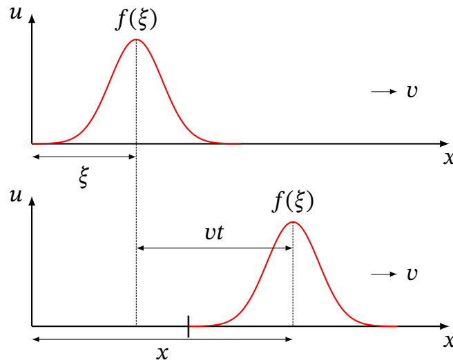
Рис. 16.2. Збурення, що поширюється без зміни форми зі швидкістю v : профіль у момент t — це профіль у момент 0, зсунутий на vt
