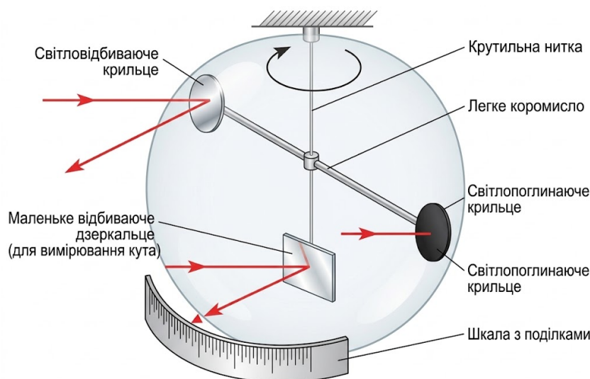
Рис. 12.6. Схема дослідів П. М. Лебедева (1899 р.) з вимірювання тиску світла
