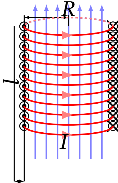
Рис. 10.18. Поздовжній переріз довгого соленоїда: однорідне поле всередині, струм у витках обмотки
