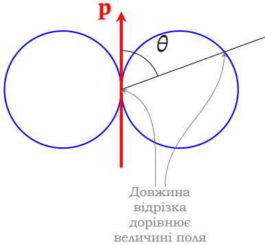
Рис. 13.8. Полярна діаграма спрямованості дипольного випромінювача: характерна форма «бублика»
