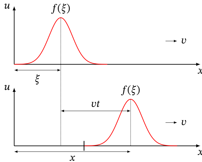
Рис. 12.2. Збурення, що поширюється без зміни форми зі швидкістю v : профіль у момент t — це профіль у момент 0, зсунутий на vt
