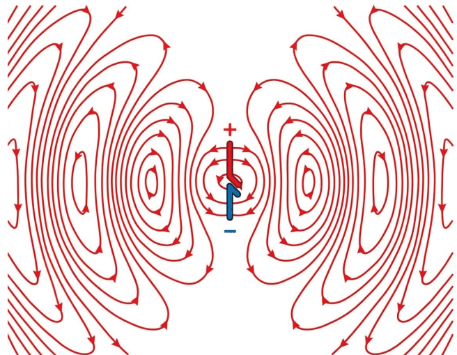
Рис. 13.7. Електричне поле осцилюючого диполя: у ближній зоні поле ніби «причеплене» до диполя, у хвильовій — випромінюється
