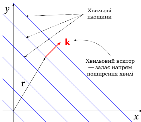
Рис. 12.3. Хвильовий вектор \mathbf{k} вказує напрям поширення плоскої хвилі й перпендикулярний до хвильових площин
