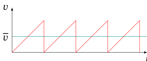
Рис. 7.6. Пилоподібна залежність швидкості електрона від часу в моделі Друде
