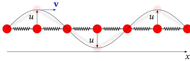
Рис. 12.1. Механічна хвиля в ланцюжку зв'язаних пружинками тягарців — наочна модель для розуміння хвильового процесу
