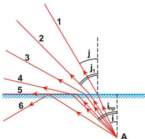
Рис. 12.10. Заломлений промінь наближається до поверхні розділу при зростанні кута падіння
