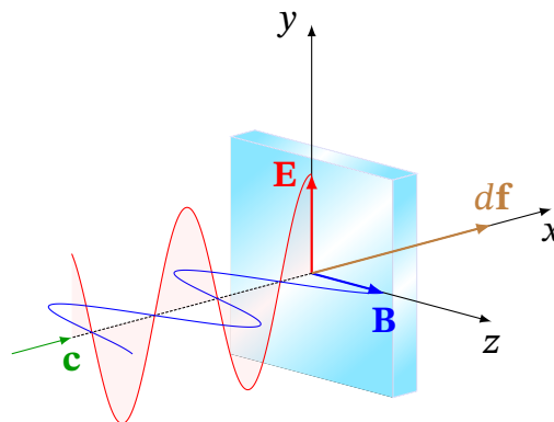
Рис. 12.5. Механізм виникнення тиску електромагнітної хвилі: сила Ампера d\mathbf{f} , що діє на струм, збуджений полем \mathbf{E} , у полі \mathbf{B}
