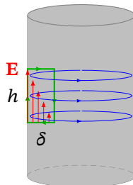
Рис. 11.12. Контур для оцінки циркуляції \mathbf{E} поблизу поверхні провідника
