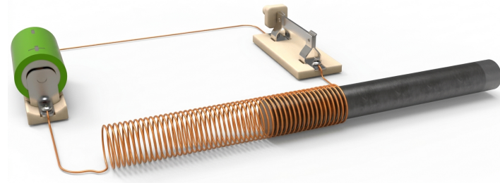
Рис. 10.19. Осердя втягується в котушку зі струмом — приклад пондеромоторної сили в магнітному полі
