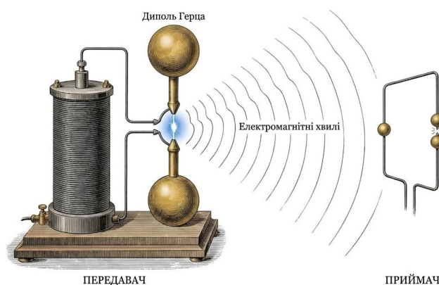
Рис. 13.1. Вібратор Герца.
