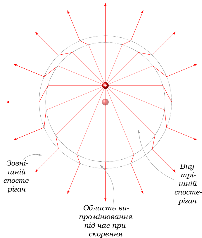
Рис. 13.3. Заломлені («злами») силові лінії поля короткочасно прискореного заряду: межа між «старим» і «новим» полем
