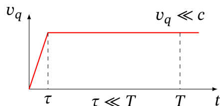
Рис. 13.2. Швидкість заряду: короткий імпульс прискорення тривалістю \tau , після якого заряд рухається рівномірно
