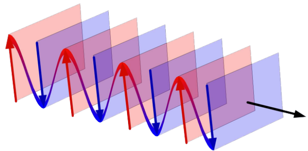
Рис. 12.3. Хвильовий вектор \mathbf{k} вказує напрям поширення плоскої хвилі й перпендикулярний до хвильових площин
