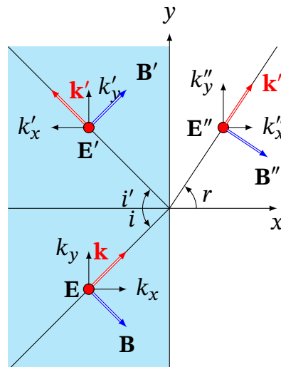
Рис. 12.8. Падаюча, відбита й заломлена s-поляризовані хвилі на межі розділу двох діелектриків
