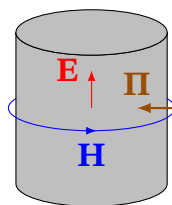
Рис. 11.9. Поля \mathbf{E} , \mathbf{H} і вектор Пойнтінга \mathbf{\Pi} на поверхні довгого провідника зі струмом
