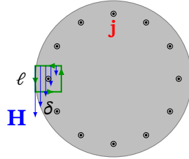
Рис. 11.13. Контур для оцінки циркуляції \mathbf{H} на перерізі провідника
