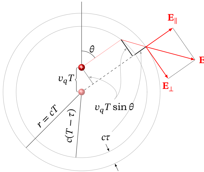
Рис. 13.4. Геометрія зламу силової лінії: розкладання поля на поздовжню E_{\parallel} і поперечну E_{\perp} складові
