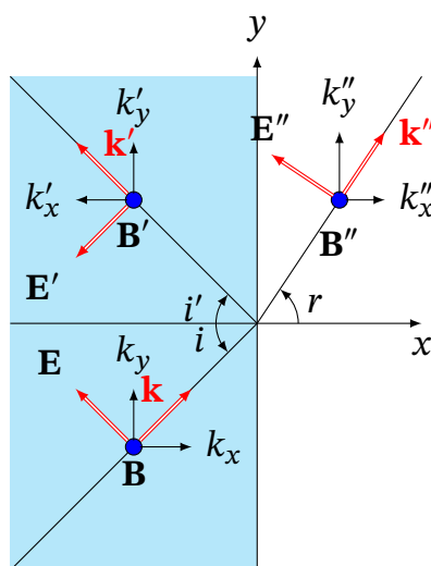
Рис. 12.9. Падаюча, відбита й заломлена p -поляризовані хвилі на межі розділу двох діелектриків
