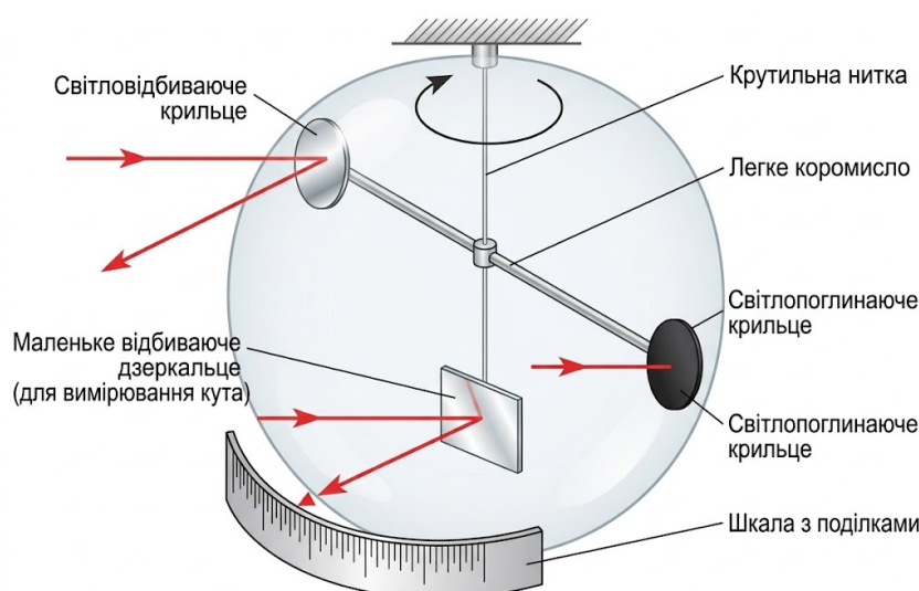
Рис. 12.6. Схема досліду П. М. Лебедева (1899 р.) з вимірювання тиску світла
