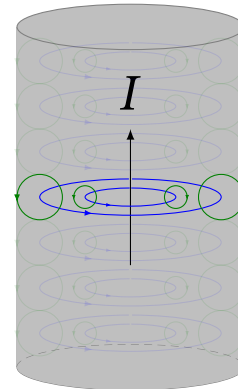
Рис. 9.6. Циліндричний провідник з парамагнетика зі струмом I : молекулярні струми (умовно показані малими витками) течуть навколо кожного елемента об'єму
