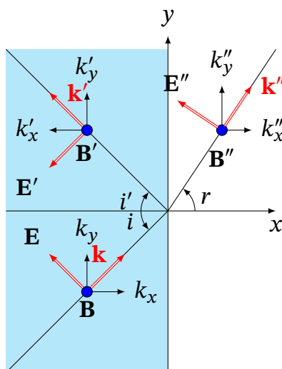
Рис. 12.11. Падаюча, відбита й заломлена p -поляризовані хвилі на межі розділу двох діелектриків
