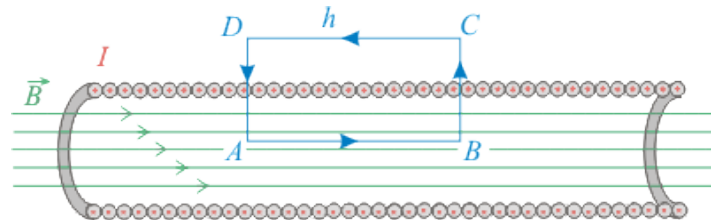
Рис. 9.5. Соленоїд, заповнений магнетиком
