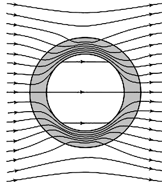
Рис. 9.10. Магнітне екранування: силові лінії концентруються в товщі феромагнітної оболонки
