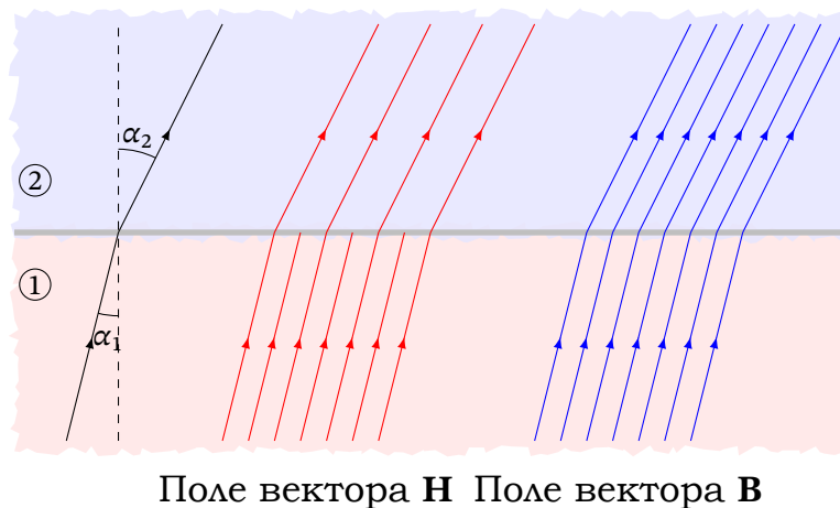
Рис. 9.9. Заломлення силових ліній \mathbf{H} і \mathbf{B} на межі розділу двох магнетиків
