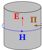
Рис. 11.9. Поля E , H і вектор Пойнтінга \Pi на поверхні довгого провідника зі струмом
