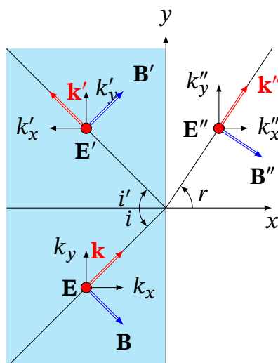
Рис. 12.10. Падаюча, відбита й заломлена s -поляризовані хвилі на межі розділу двох діелектриків
