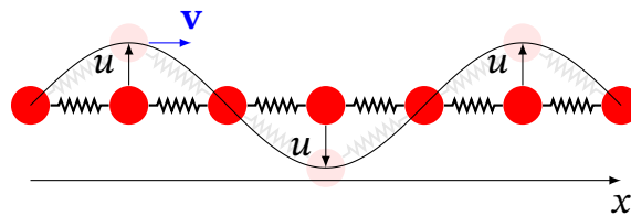
Рис. 12.1. Механічна хвиля в ланцюжку зв'язаних пружинками тягарців — наочна модель для розуміння хвильового процесу
