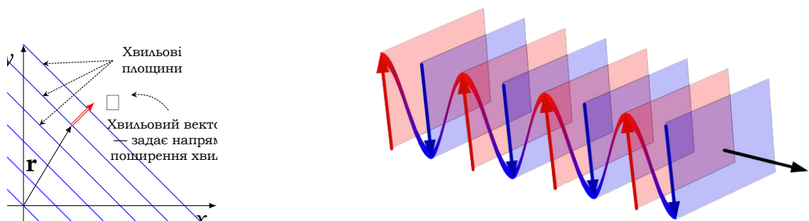
Рис. 12.3. Хвильовий вектор \mathbf{k} вказує напрям поширення плоскої хвилі й перпендикулярний до хвильових площин
