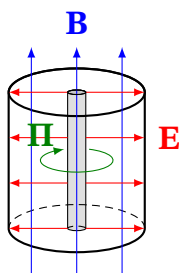
Рис. 12.9. Циліндричний конденсатор в аксіальному магнітному полі: поля \mathbf{E} , \mathbf{B} і вектор Пойнтінга \mathbf{\Pi} , що циркулює навколо осі конденсатора та кутову швидкість, з якою конденсатор почне обертатися після вимкнення поля \mathbf{B} .
