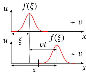
Рис. 12.2. Збурення, що поширюється без зміни форми зі швидкістю v : профіль у момент t — це профіль у момент 0, зсунутий на vt
