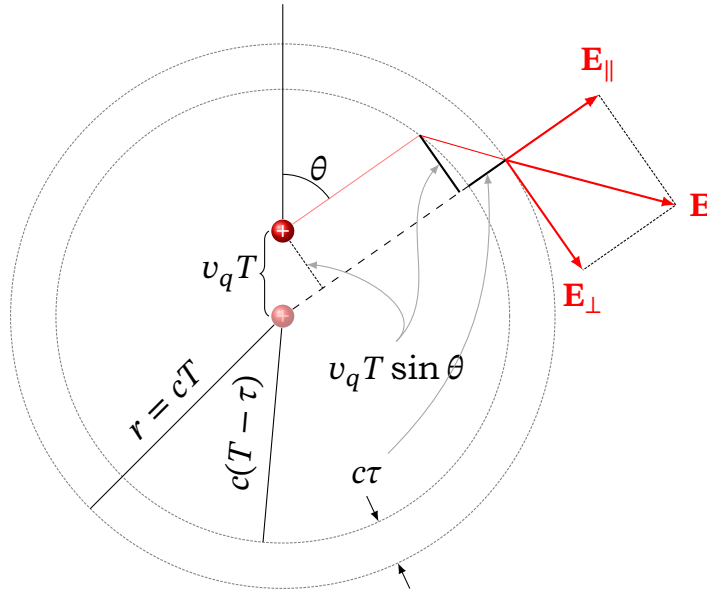
Рис. 13.4. Геометрія зламу силової лінії: розкладання поля на поздовжню E_{\parallel} і поперечну E_{\perp} складові
