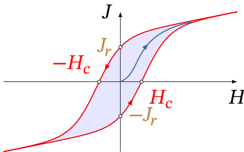
Рис. 9.12. Петля гістерезису ферромагнетика: J_r — залишкова намагніченість, H_c — коерцитивна сила
