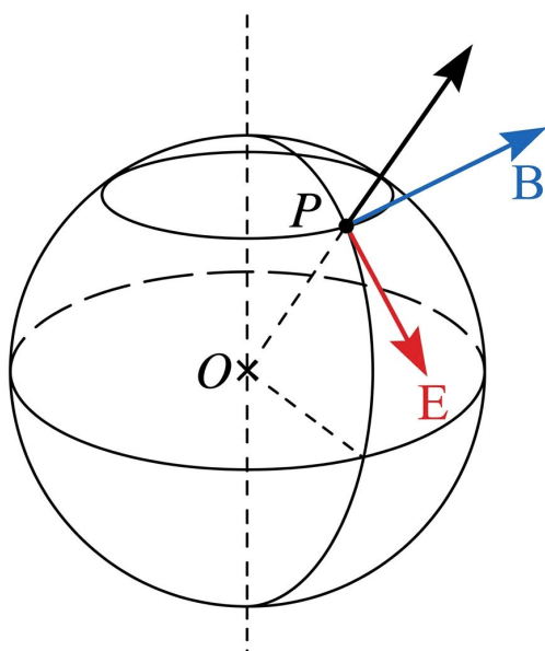
Рис. 13.6. Поля E_\theta і B_\varphi у хвильовій зоні диполя
