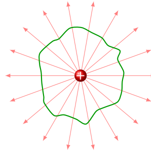
Рис. 1.21. До поняття циркуляції вектора \mathbf{E}
