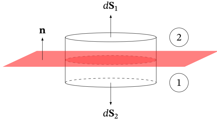
Рис. 1.30. До виведення першої граничної умови
