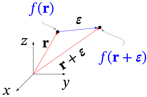
Рис. 1.27. Ілюстрація до формул. Функція-поле f(\mathbf{r}) і різних точках простору.
