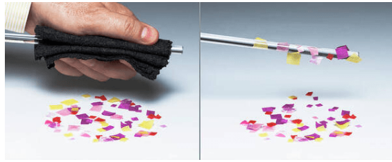
Рис. 1.3. Електризація тертям
