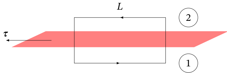
Рис. 1.31. До виведення другої граничної умови
