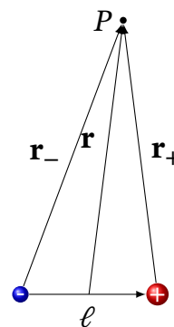
Рис. 1.13. До виведення напруженості поля диполя
