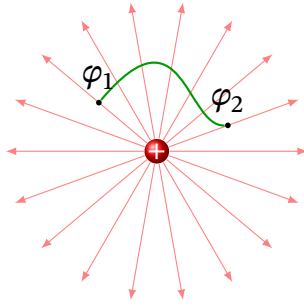
Рис. 1.20. До задачі виведення різниці потенціалів
