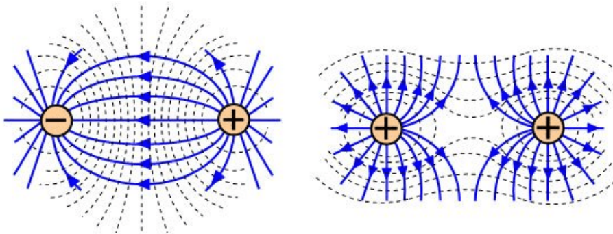
Рис. 1.8. Вигляд силових ліній системи двох зарядів
