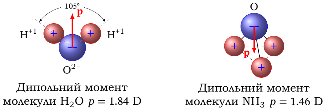
Рис. 1.10. ілюстрація дипольних моментів деяких полярних молекул
