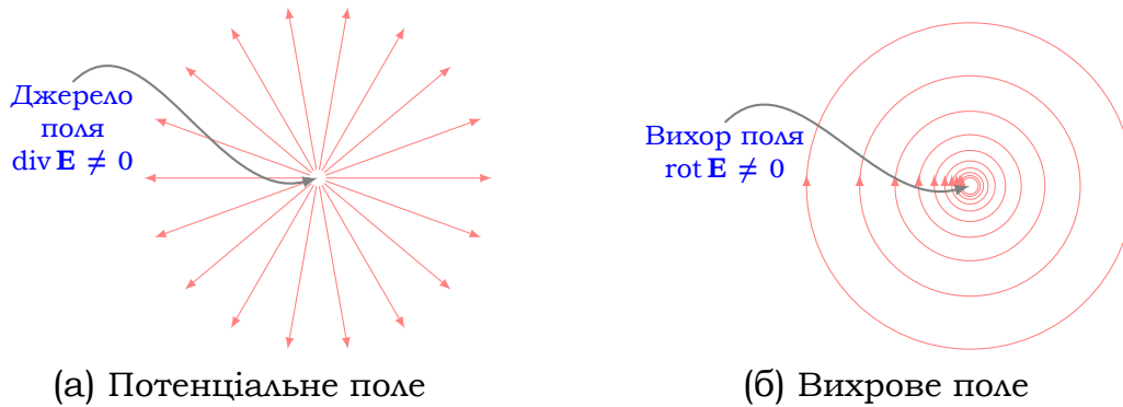
Рис. 1.23. Приклад силових ліній потенціального та вихрового полів
