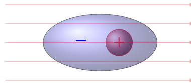
Рис. 1.12. Дипольний момент виник під дією зовнішнього поля p \neq 0 .
