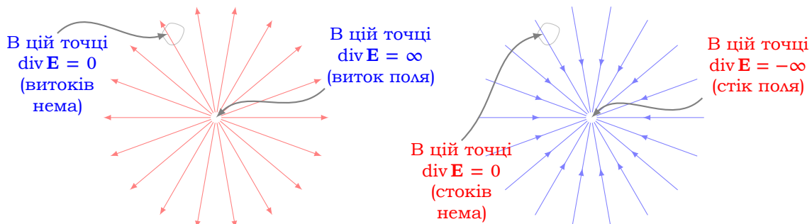
Рис. 1.18. У тих точках поля, де дивергенція поля \mathbf{E} більша нуля , ми маємо джерела поля (позитивні заряди), а в тих точках, де вона менше нуля , — стоки (негативні заряди). Лінії вектора \mathbf{E} виходять із витоків поля, а в місцях стоків вони закінчуються.
