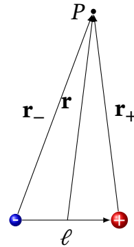
Рис. 1.26. До виведення потенціалу диполя.
