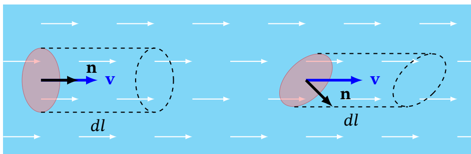
Рис. 1.15. До виведення поняття потоку вектора
