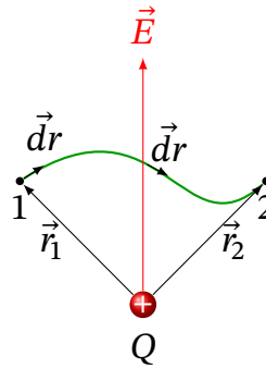
Рис. 1.19. До виведення роботи сил поля по переміщенню пробного заряду.
