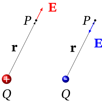
Рис. 1.5. Напруженість поля точкового заряду Q в точці спостереження P . Для додатного і від'ємного зарядів напрямки вектора напруженості E відрізняються.
