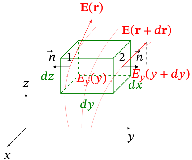
Рис. 1.16. До виведення диференціальної форми теореми Гаусса
