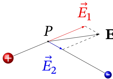
Рис. 1.6. Ілюстрація принципу суперпозиції для випадку двох різноіменних зарядів
