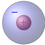
Рис. 1.11. Дипольний момент без зовнішнього поля p = 0 .
