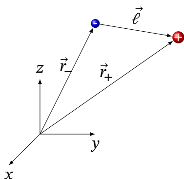
Рис. 1.9. Електричний диполь
