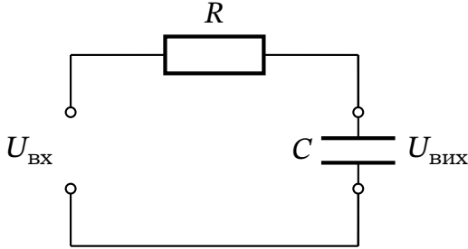
Рис. 17.12. Фільтр низьких частот: вихідна напруга знімається з конденсатора C .
