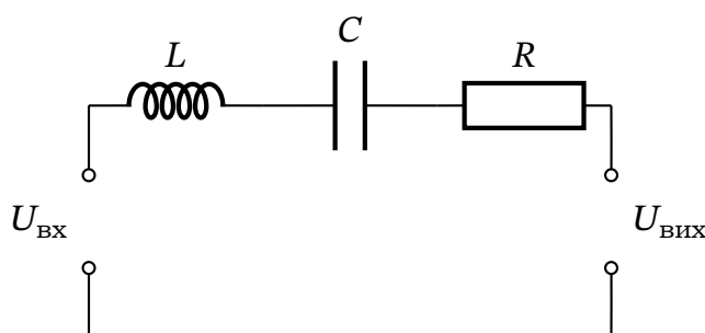
Рис. 17.14. Смуговий фільтр на основі послідовного LCR -контурі: вихідна напруга знімається з резистора R .
