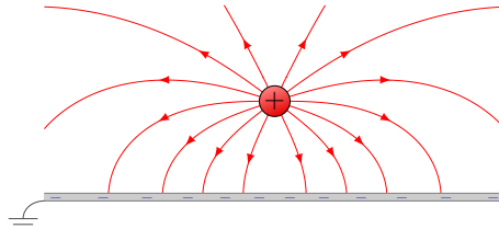
Рис. 4.13. Точковий заряд q поблизу нескінченної заземленої провідної площини.
