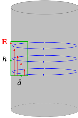
Рис. 13.9. Контур для оцінки циркуляції \mathbf{E} поблизу поверхні провідника
