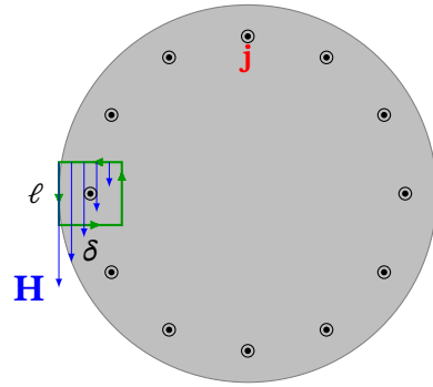
Рис. 13.10. Контур для оцінки циркуляції \mathbf{H} поблизу поверхні провідника
