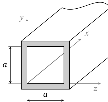
Рис. 19.1. Прямокутний хвильовід
