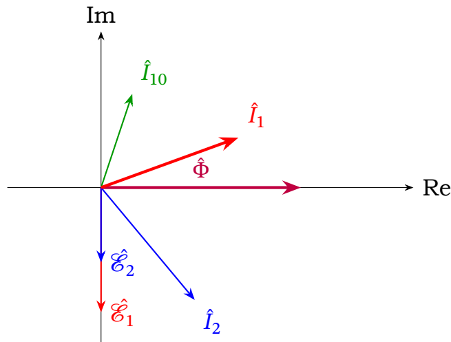
Рис. 17.14. Векторна діаграма трансформатора в режимі навантаження. Потік \Phi напрямлений уздовж дійсної осі; ЕРС відстають від нього на \pi/2 ; струм \hat{I}_1 є сумою струму холостого ходу та скомпенсованого вторинного струму.
