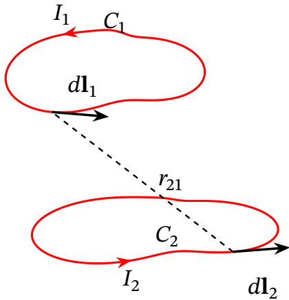
Рис. 12.3. До доведення теореми взаємності. Зображено контури C_1 і C_2 , елементи d\mathbf{l}_1 , d\mathbf{l}_2 та радіус-вектор r_{21} між ними, які використовуються при обчисленні потоку \Phi_{12} .
