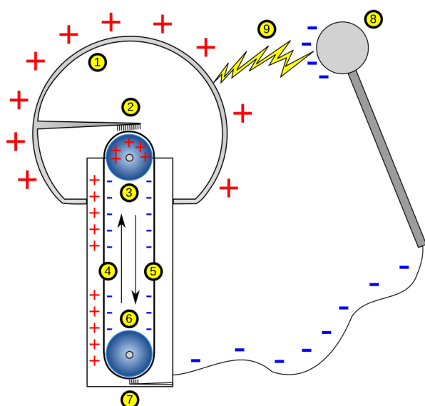
Рис. 4.8. Генератор Ван-де-Граафа
