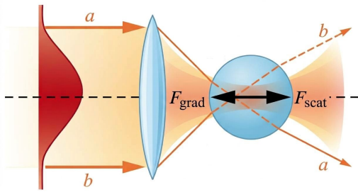
Рис. 15.7. Оптичний пінцет. Промені a і b показують заломлення світла на частинці, яке й породжує градієнтну силу
