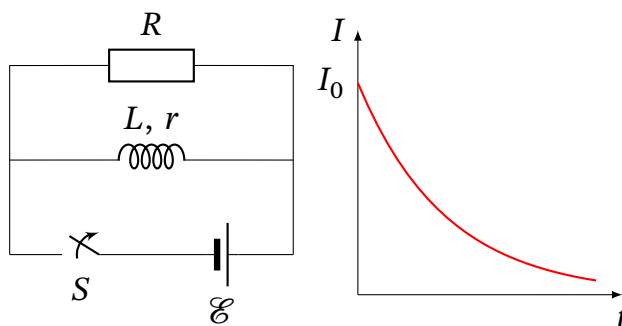
Рис. 11.11. Екстраструм розмикання в колі з індуктивністю
