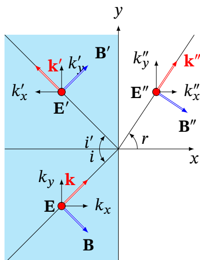
Рис. 15.9. Падаюча, відбита й заломлена s-поляризовані хвилі на межі розділу двох діелектриків
