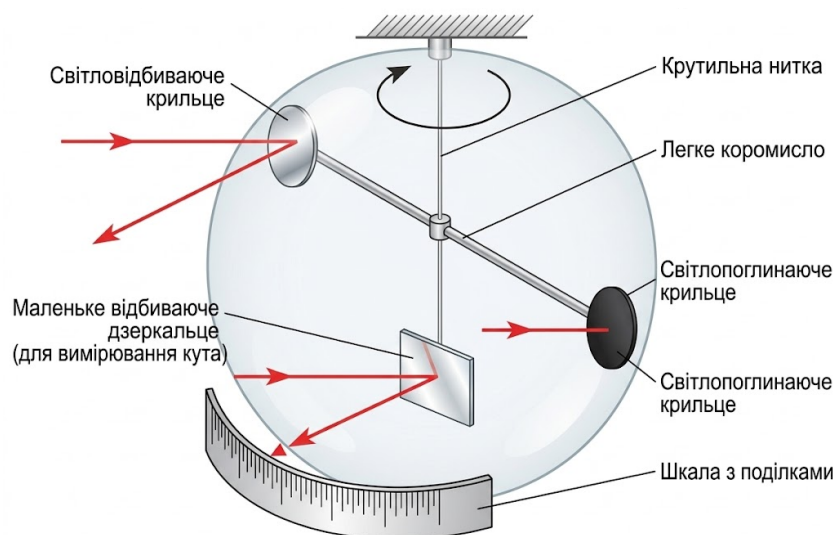
Рис. 15.6. Схема досліду П. М. Лебедева (1899 р.) з вимірювання тиску світла
