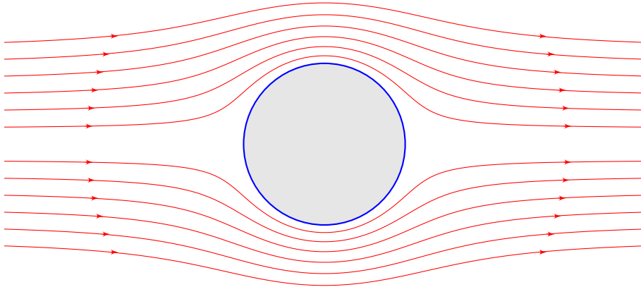
Рис. 11.12. Надпровідна куля в зовнішньому магнітному полі: силові лінії обтікають кулю, не проникаючи всередину — поле виштовхується поверхневими екрануючими струмами
