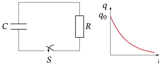
Рис. 7.16. Розрядка конденсатора через резистор: коло та графік q(t)
