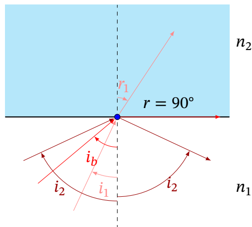
Рис. 15.11. Заломлений промінь наближається до поверхні розділу при зростанні кута падіння
