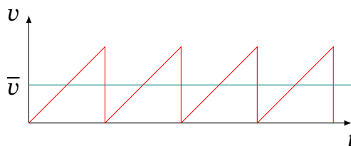
Рис. 7.6. Пілоподібна залежність швидкості електрона від часу в моделі Друде
