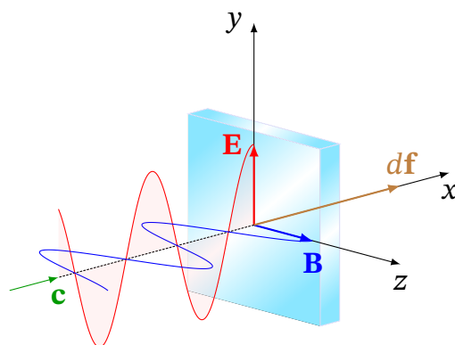
Рис. 15.5. Механізм виникнення тиску електромагнітної хвилі: сила Ампера df , що діє на струм, збуджений полем \mathbf{E} , у полі \mathbf{B}
