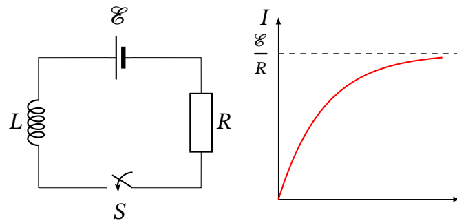
Рис. 11.10. Встановлення струму в колі з індуктивністю після замикання ключа
