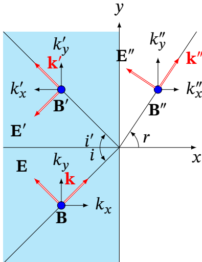
Рис. 15.10. Падаюча, відбита й заломлена p -поляризовані хвилі на межі розділу двох діелектриків
