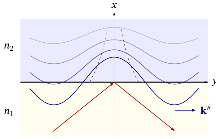
Рис. 15.12. Згасаюча хвиля в другому середовищі при i > i_b (s-поляризація:
