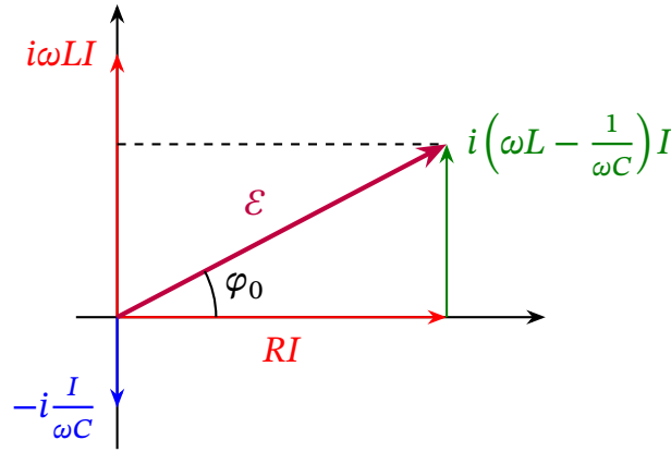
Рис. 17.7. Векторна діаграма для LCR-контуру, показаного на рис. 17.1, для випадку \omega L > 1/\omega C .
