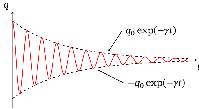
Рис. 17.2. Графік затухаючих коливань. Штриховою лінією показано часову залежність амплітуди A(t) = q_0 e^{-\gamma t} .
