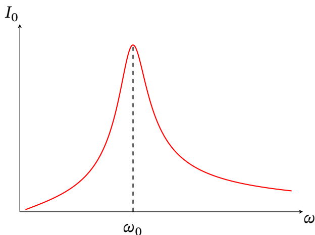
Рис. 17.8. Залежність амплітуди коливань струму від частоти коливань ЕРС — резонанс напруги на конденсаторі і ЕРС в послідовному LCR -контурі (рис. 17.1).
