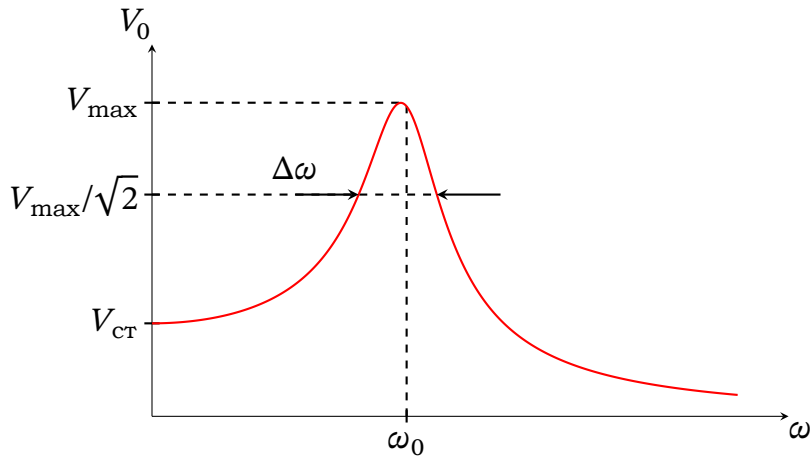
Рис. 17.6. Характеристики резонансної кривої: V_{\text{max}} — максимум амплітуди, V_{\text{ст}} — статична амплітуда, \Delta\omega — ширина резонансу.
