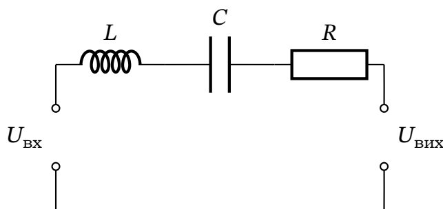
Рис. 17.14. Смуговий фільтр на основі послідовного LCR -контур: вихідна напруга знімається з резистора R .
