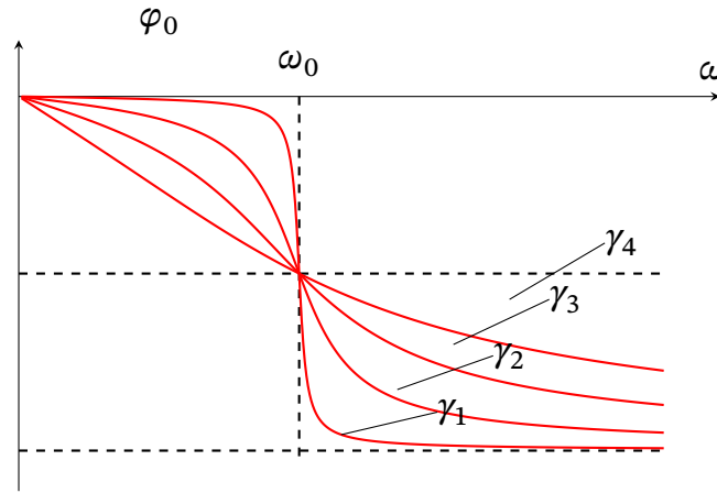
Рис. 17.5. Фазово-частотна характеристика контуру. Залежність фазового зсуву \varphi_0 від частоти \omega зовнішньої ЕРС.
