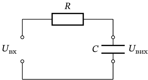
Рис. 17.12. Фільтр низьких частот: вихідна напруга знімається з конденсатора C .
