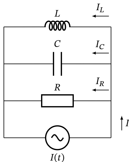
Рис. 17.9. Паралельний LCR -контур, що включає джерело заданого змінного струму I(t) = I_0 \cos \omega t .
