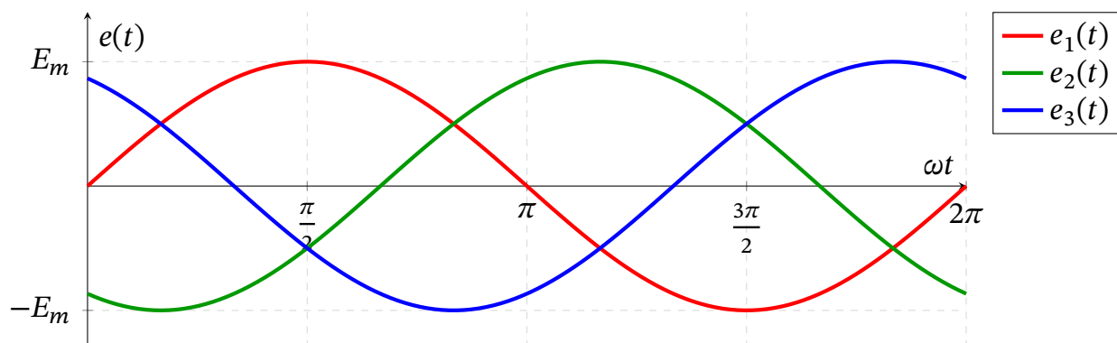
Рис. 17.17. Часові діаграми симетричної трифазної системи ЕРС
