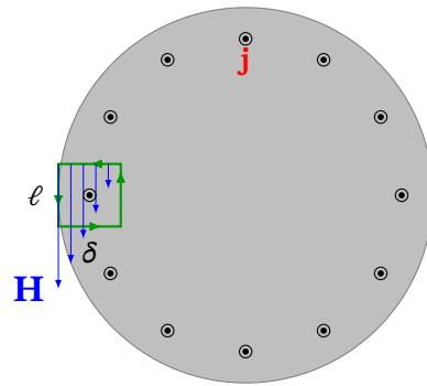
Рис. 13.11. Контур для оцінки циркуляції \mathbf{H} поблизу поверхні провідника
