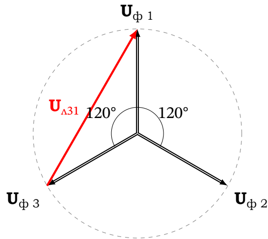
Рис. 17.19. Векторна діаграма співвідношення фазних та лінійних напруг
