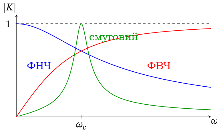
Рис. 17.15. Амплітудно-частотні характеристики трьох фільтрів: ФНЧ (синій), ФВЧ (червоний) і смугового (зелений). Для смугового прийнято Q = 5 .
