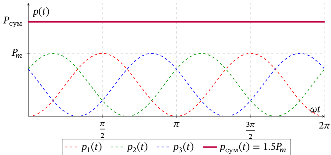
Рис. 17.21. Миттєва потужність окремих фаз та сумарна потужність трифазної системи
