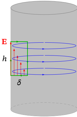
Рис. 13.10. Контур для оцінки циркуляції \mathbf{E} поблизу поверхні провідника
