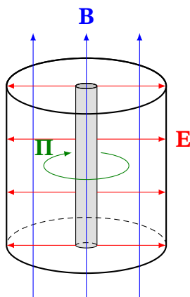
Рис. 15.7. Циліндричний конденсатор в аксіальному магнітному полі: поля \mathbf{E} , \mathbf{B} і вектор Пойнтінга \mathbf{\Pi} , що циркулює навколо осі
