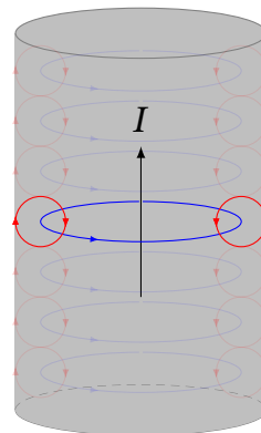
Рис. 13.9. Якісний механізм скін-ефекту: вихрові струми Фуко підсилюють струм на поверхні й послаблюють у центрі провідника
