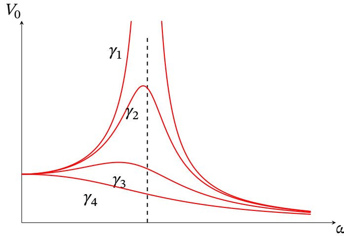
Рис. 17.4. Амплітудно-частотна характеристика контуру. Залежність амплітуди вимушених коливань V_0 від частоти \omega зовнішньої ЕРС.
