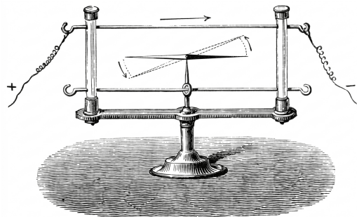
Рис. 8.1. Установка Ерстеда
