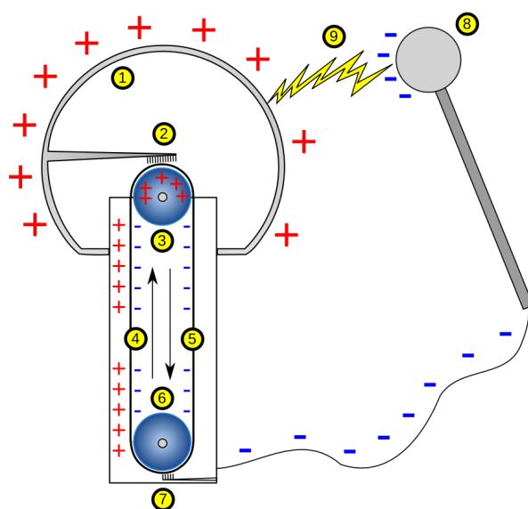
Рис. 4.8. Генератор Ван-де-Граафа
