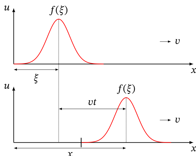
Рис. 13.2. Збурення, що поширюється без зміни форми зі швидкістю v : профіль у момент t — це профіль у момент 0, зсунутий на vt
