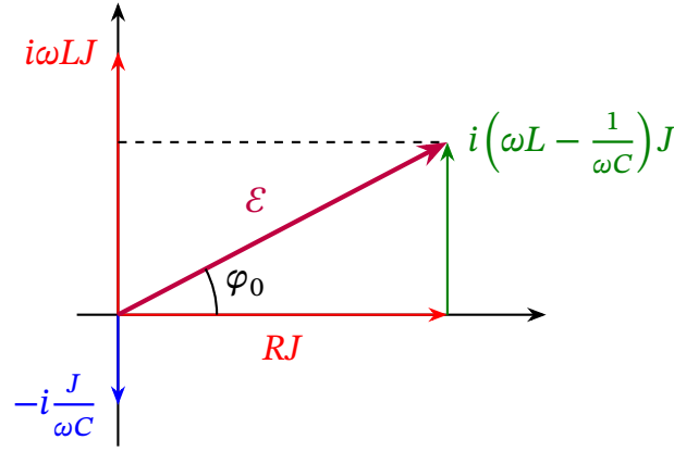
Рис. 15.7. Векторна діаграма для LCR -контурі, показаного на рис. 15.1, для випадку \omega L > 1/\omega C .
