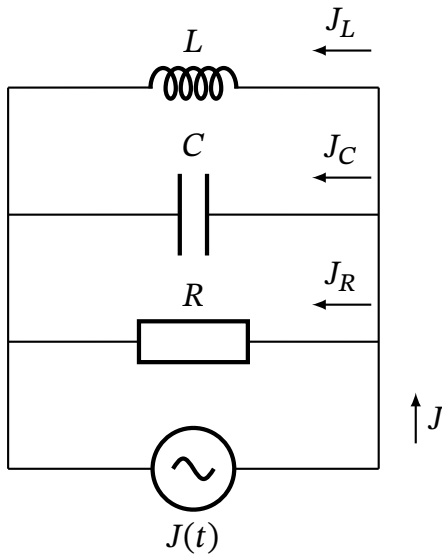
Рис. 15.9. Паралельний LCR -контур, що включає джерело заданого змінного струму J(t) = J_0 \cos \omega t .
