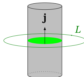
(б) Зовні: B = \frac{2I}{cr}
