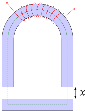
Рис. 10.20. Електромагніт з якорем, відокремленим повітряним зазором x
