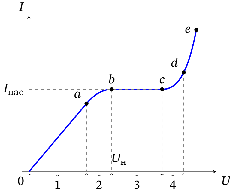
Рис. 8.6. Схематична вольт-амперна характеристика розряду в газі: омічна ділянка (1), перехідна ділянка (2), струм насичення (3), лавинне зростання й пробій (4); точки a–e — характерні режими
