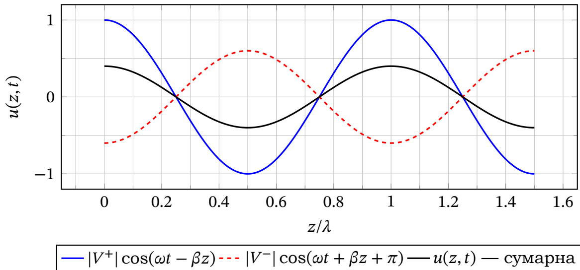
Рис. 19.2. Інтерференція падаючої та відбитої хвиль у лінії без втрат при |V^-|/|V^+| = 0.6 . Сумарна напруга утворює стоячу хвилю з вузлами та пучностями. Коефіцієнт стоячої хвилі КСХ = (1 + 0.6)/(1 - 0.6) = 4 .
