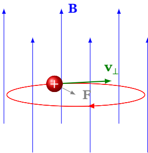
Рис. 9.5. Кругова траєкторія зарядженої частинки в однорідному магнітному полі: сила завжди перпендикулярна до швидкості
