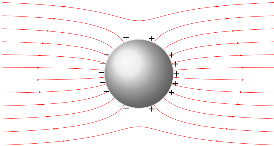
Рис. 4.17. Конфігурація поля навколо металевої кулі, вміщеної в однорідне електричне поле.
