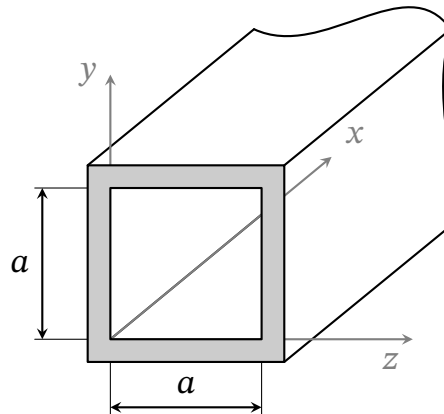
Рис. 20.1. Прямокутний хвилевід
