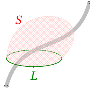
Рис. 9.9. Контур L і натягнута на нього поверхня S , крізь яку протікає струм
