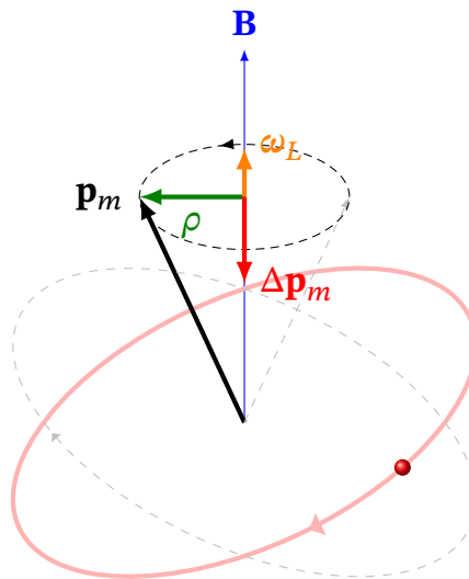
Рис. 10.9. Прецесія орбіти електрона в зовнішньому полі B : магнітний момент p m (а разом з ним і площина орбіти) обертається навколо B з ларморовою частотою \omega_L . Ця прецесія еквівалентна додатковому коловому струму I = -e\omega_L/(2\pi) , який створює індукований магнітний момент Δp , направлений проти B .
