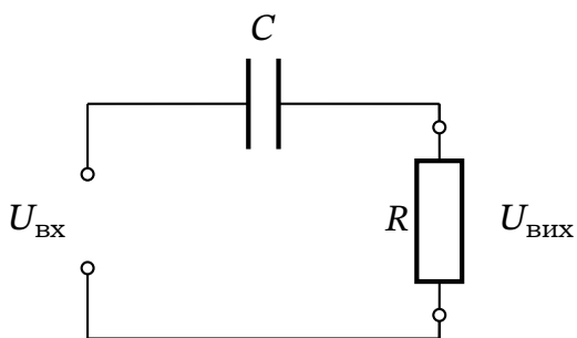
Рис. 18.16. Фільтр високих частот: вихідна напруга знімається з резистора R .
