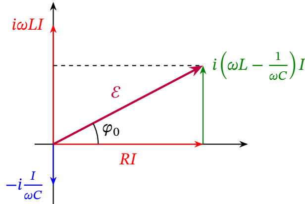
Рис. 18.8. Векторна діаграма для LCR-контуру, показаного на рис. 18.1, для випадку \omega L > 1/\omega C .
