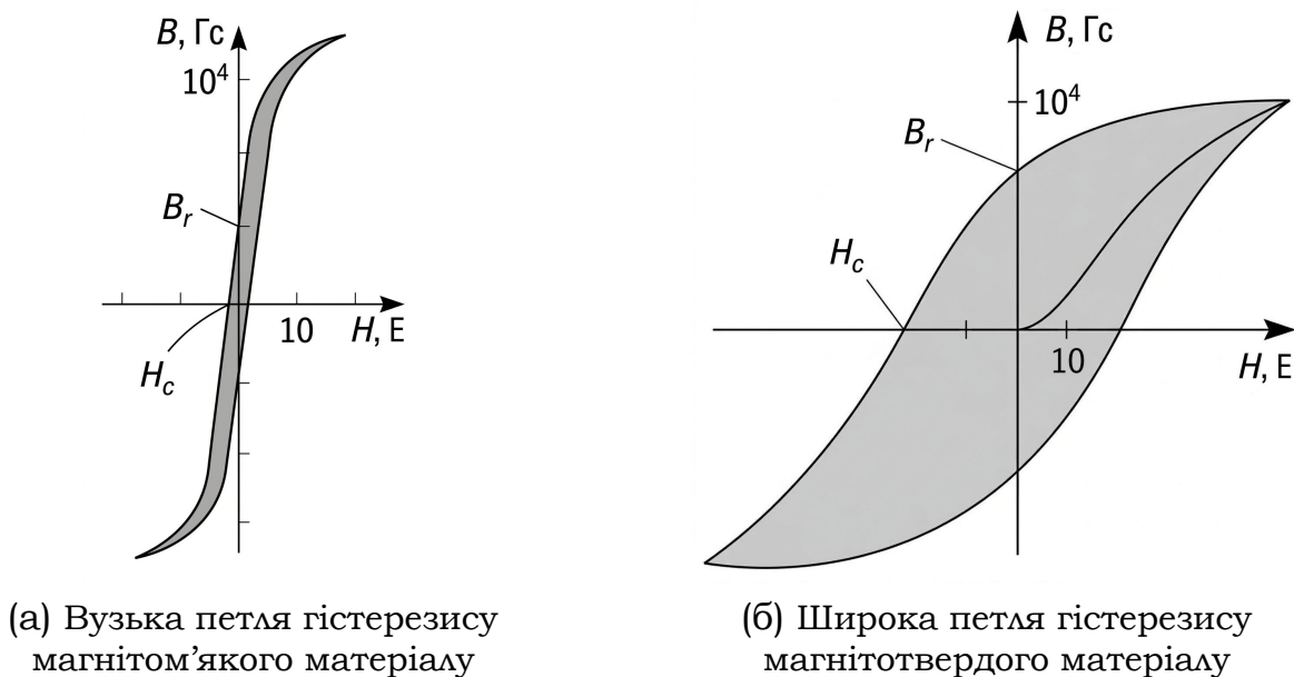
Рис. 10.12. Петлі гістерезису магнітом'якого та магнітотвердого матеріалів
