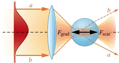
Рис. 16.7. Оптичний пінцет. Промені a і b показують заломлення світла на частинці, яке й породжує градієнтну силу
