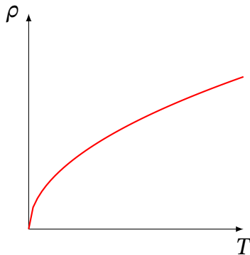
Рис. 8.1. Передбачення найпростішої теорії Друде: \rho \propto \sqrt{T}
