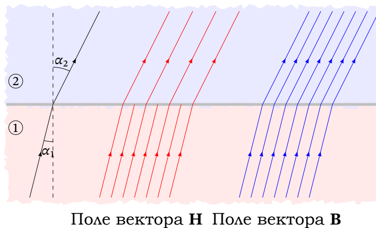
Рис. 10.7. Заломлення силових ліній \mathbf{H} і \mathbf{B} на межі розділу двох магнетиків
