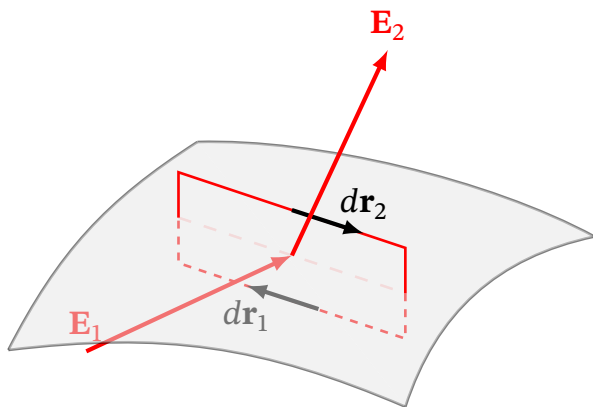
Рис. 5.9. Контур циркуляції на межі розділу двох середовищ для виведення граничної умови на тангенціальну складову E
