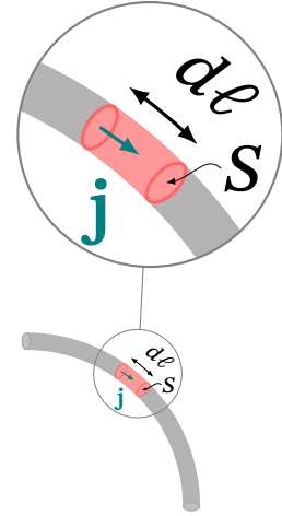
Рис. 9.3. Елемент лінійного струму I d\ell : збільшений фрагмент показує напрям \mathbf{j} уздовж осі провідника перерізу S
