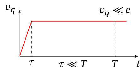
Рис. 17.2. Швидкість заряду: короткий імпульс прискорення тривалістю \tau , після якого заряд рухається рівномірно
