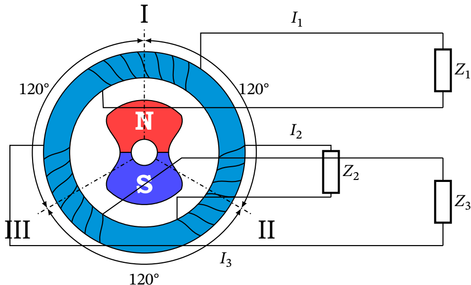
Рис. 18.19. Схематичне зображення трифазного синхронного генератора
