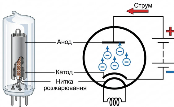
Рис. 8.10. Вигляд вакуумного діода: нагрітий катод емітує електрони, які прискорюються до анода під дією електричного поля. При зміні полярності анода струм не проходить.
