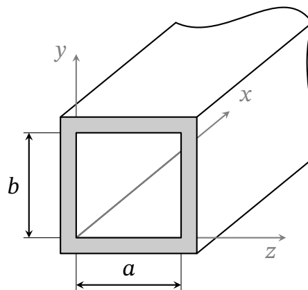
Рис. 20.1. Прямокутний хвиевід
