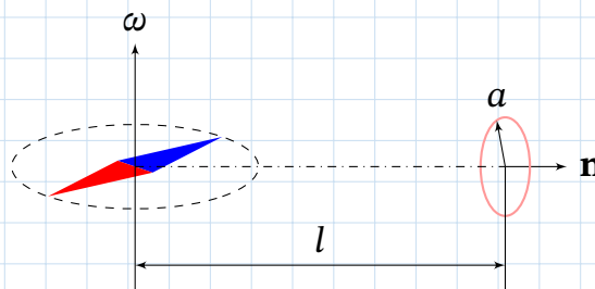
Рис. 13.5. Магнітний диполь, що обертається, і нерухоме кільце на відстані \ell
