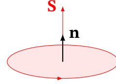
Рис. 2.18. Орієнтована площа
