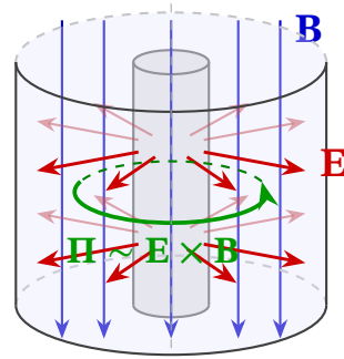
Рис. 16.8. Циліндричний конденсатор в аксіальному магнітному полі: зображено поля \mathbf{E} , \mathbf{B} і вектор Пойнтінга \mathbf{P} , що циркулює навколо осі
