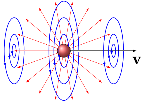
Рис. 9.2. Заряд, що рухається зі швидкістю \mathbf{v} , є джерелом як електричного, так і магнітного поля
