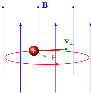
Рис. 9.5. Кругова траєкторія зарядженої частинки в однорідному магнітному полі: сила завжди перпендикулярна до швидкості
