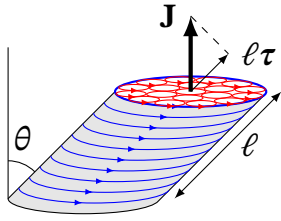
Рис. 10.2. Косокутний циліндр у намагніченій речовині
