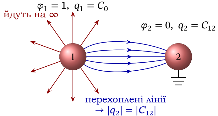
Рис. 6.1. Частина силових ліній провідника 1 замикається на заземленому провіднику 2, решта йде на нескінченність
