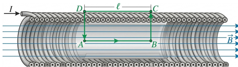
Рис. 9.11. До розрахунку магнітного поля нескінченно довгого соленоїда.
