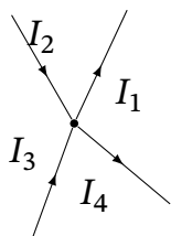
Рис. 7.10. Вузол розгалуженого кола: I_1 + I_4 = I_2 + I_3
