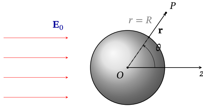
Рис. 4.16. Металева куля радіуса R в однорідному зовнішньому полі E_0 . Початок координат O суміщено з центром кулі, полярну вісь направлено вздовж E_0 . Положення точки P задається радіус-вектором \mathbf{r} та кутом \theta між \mathbf{r} і полярною віссю.
