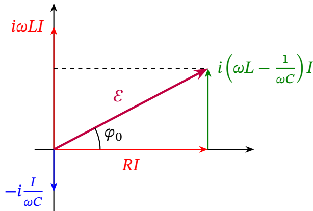
Рис. 17.8. Векторна діаграма для LCR-контурі, показаного на рис. 17.1, для випадку \omega L > 1/\omega C .
