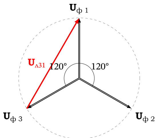
Рис. 17.21. Векторна діаграма співвідношення фазних та лінійних напруг
