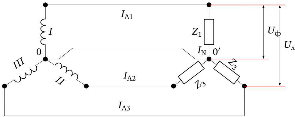
Рис. 17.20. З'єднання трифазної системи зіркою з нейтральним проводом
