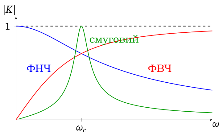
Рис. 17.17. Амплітудно-частотні характеристики трьох фільтрів: ФНЧ (синій), ФВЧ (червоний) і смугового (зелений). Для смугового прийнято Q = 5 .
