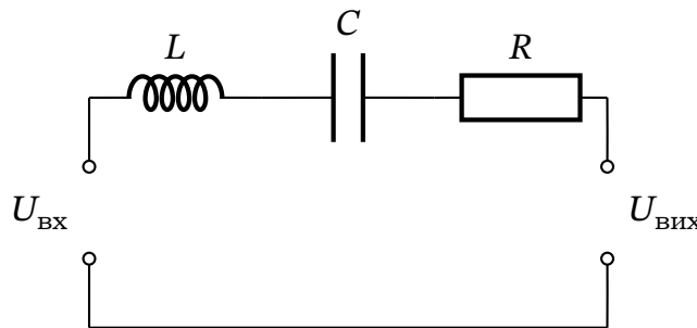
Рис. 17.16. Смуговий фільтр на основі послідовного LCR -контур: вихідна напруга знімається з резистора R .
