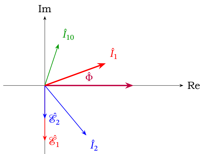
Рис. 17.13. Векторна діаграма трансформатора в режимі навантаження. Потік \hat{\Phi} направлений уздовж дійсної осі; ЕРС відстають від нього на \pi/2 ; струм \hat{I}_1 є сумою струму холостого ходу та скомпенсованого вторинного струму.
