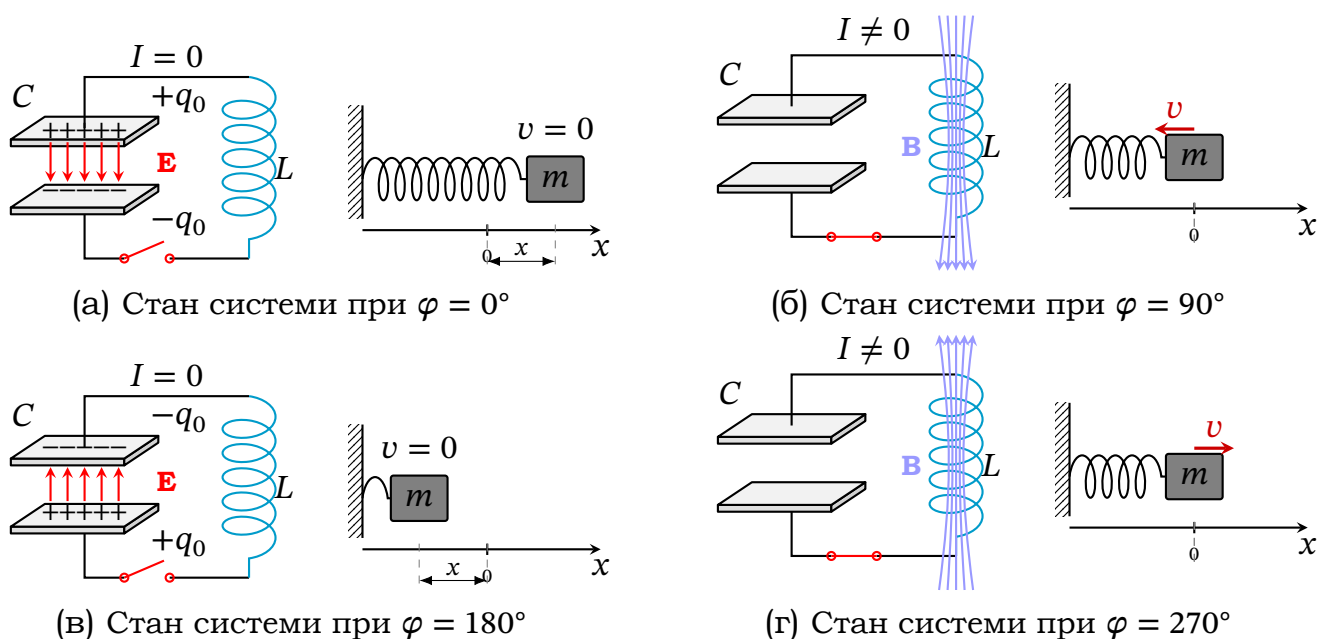
Рис. 17.2. Фази коливань електричного та магнітного полів у коливальному контурі та координати пружинного маятника
