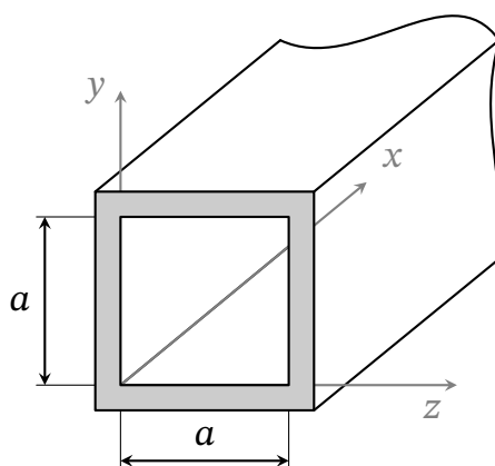
Рис. 19.1. Прямокутний хвильовід
