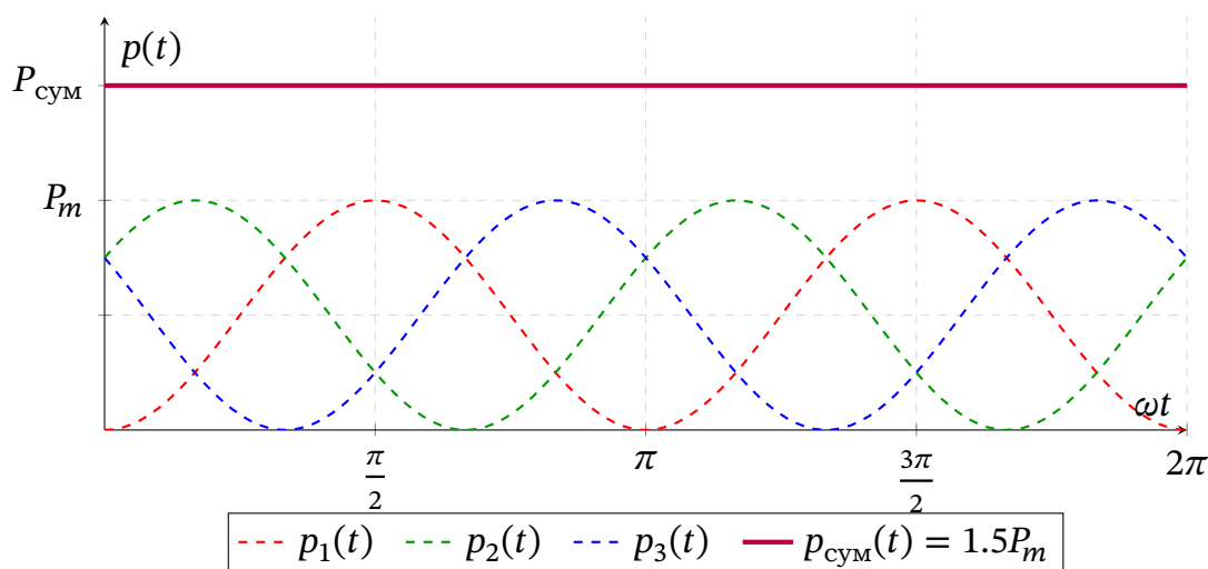
Рис. 17.23. Миттєва потужність окремих фаз та сумарна потужність трифазної системи
