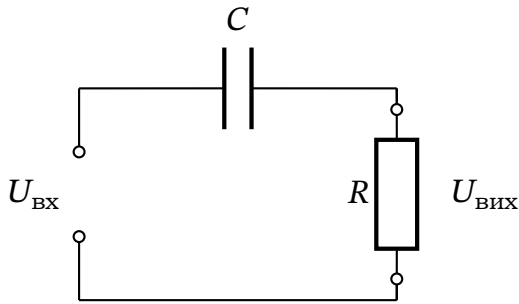
Рис. 17.15. Фільтр високих частот: вихідна напруга знімається з резистора R .
