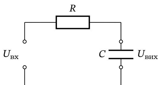
Рис. 17.14. Фільтр низьких частот: вихідна напруга знімається з конденсатора C .
