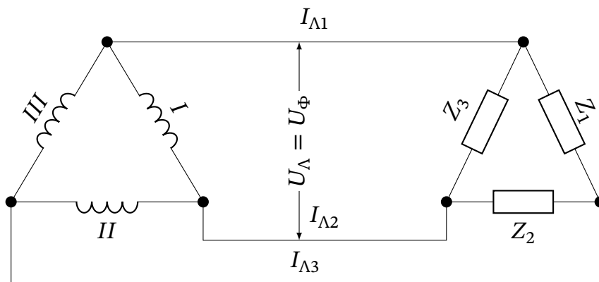
Рис. 17.22. Схема з'єднання генератора та приймача трикутником
