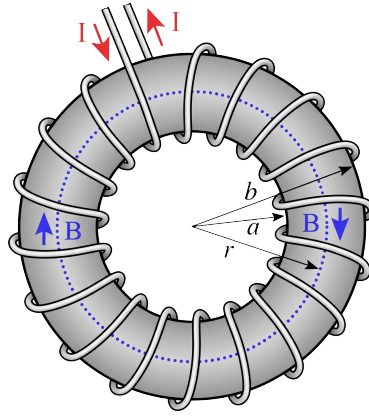
Рис. 11.10. Тороїдальна котушка
