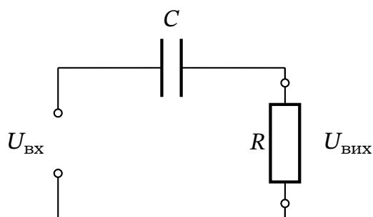
Рис. 17.14. Фільтр високих частот: вихідна напруга знімається з резистора R .
