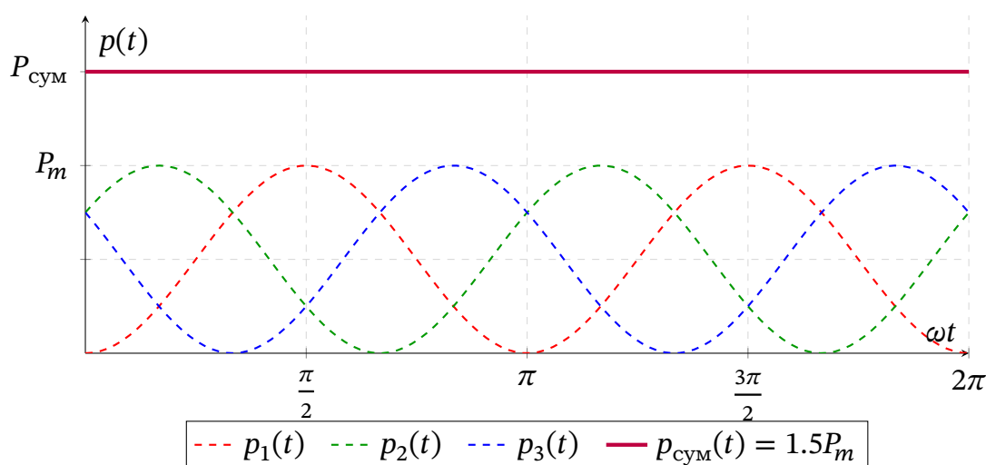
Рис. 17.22. Миттєва потужність окремих фаз та сумарна потужність трифазної системи
