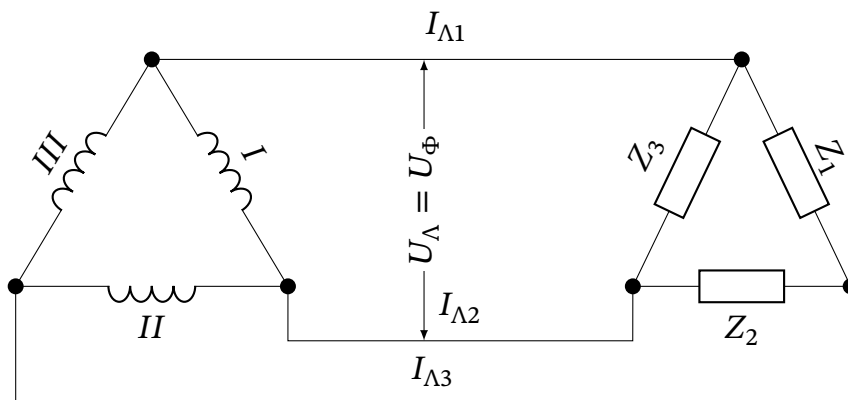
Рис. 17.21. Схема з'єднання генератора та приймача трикутником
