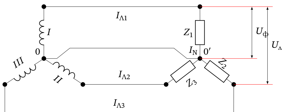
Рис. 17.19. З'єднання трифазної системи зіркою з нейтральним проводом
