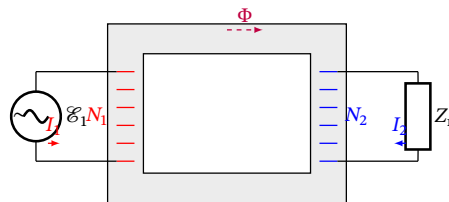
Рис. 1. Схематична будова трансформатора: первинна обмотка N_1 підключена до джерела \mathcal{E}_1 , вторинна N_2 — до навантаження Z_{\text{н}} . Спільне осердя забезпечує магнітний зв'язок між обмотками.
