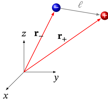
Рис. 3.1. Електричний диполь
