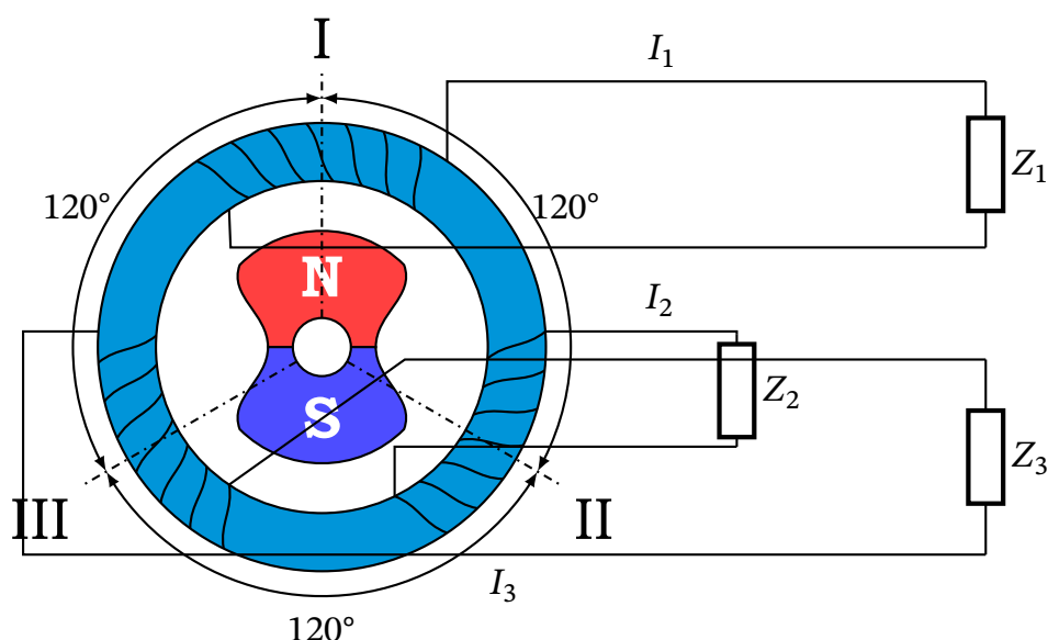
Рис. 17.17. Схематичне зображення трифазного синхронного генератора
