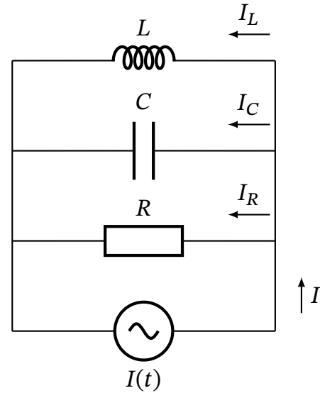
Рис. 17.10. Паралельний LCR -контур, що включає джерело заданого змінного струму I(t) = I_0 \cos \omega t .
