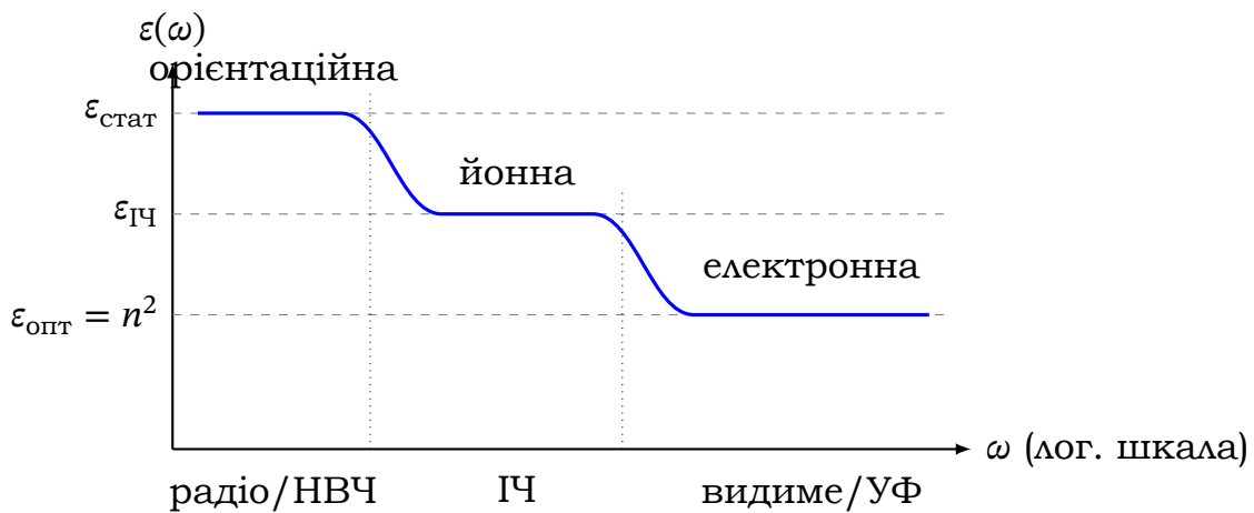
Рис. 6.1. Схематична залежність діелектричної проникності від частоти: три «сходинки» відповідають послідовному «вимиканню» орієнтаційного, йонного та електронного механізмів
