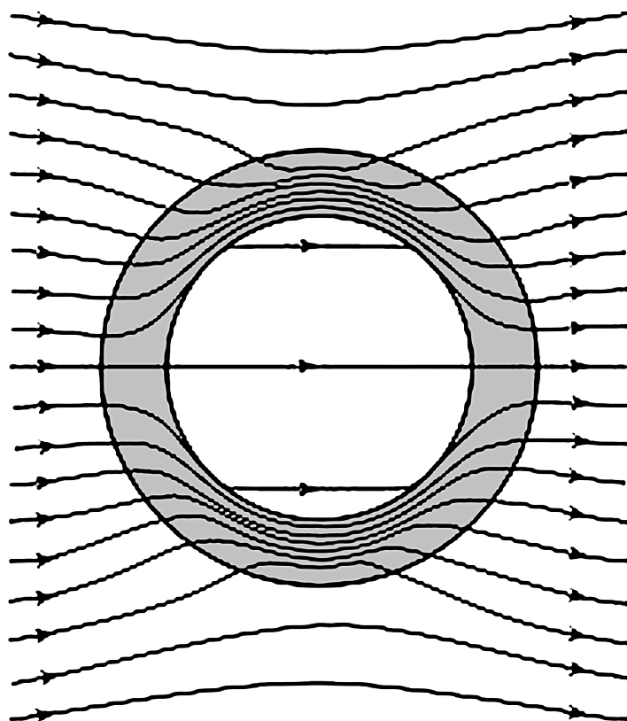
Рис. 11.10. Магнітне екранування: силові лінії концентруються в товщі феромагнітної оболонки
