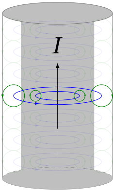
Рис. 11.6. Циліндричний провідник з парамагнетика зі струмом I : молекулярні струми (умовно показані малими витками) течуть навколо кожного елемента об'єму
