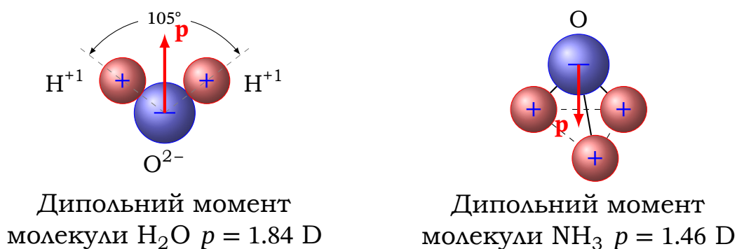
Рис. 3.2. Ілюстрація дипольних моментів деяких полярних молекул
