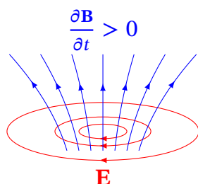
Рис. 12.9. Вихрове електричне поле, породжене зростаючим у часі магнітним полем
