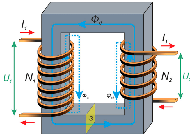
Рис. 12.17. Принципова схема трансформатора
