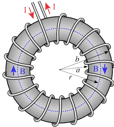
Рис. 11.11. Тороїдальна котушка
