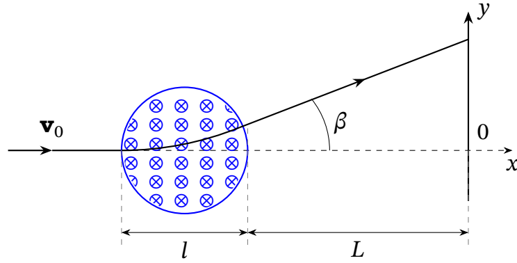
Рис. 10.6. Відхилення зарядженої частинки магнітним полем. М — магніт, Е — екран. Напрямок магнітного поля перпендикулярно площині листа і напрямлено «за лист».
