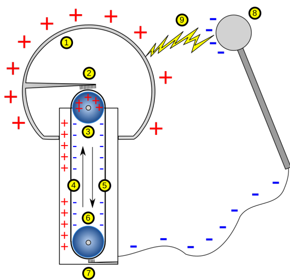
Рис. 4.8. Генератор Ван-де-Граафа
