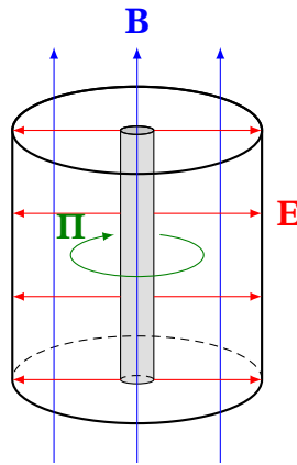
Рис. 14.7. Циліндричний конденсатор в аксіальному магнітному полі: поля \mathbf{E} , \mathbf{B} і вектор Пойнтінга \mathbf{\Pi} , що циркулює навколо осі об'ємом між обкладками:
