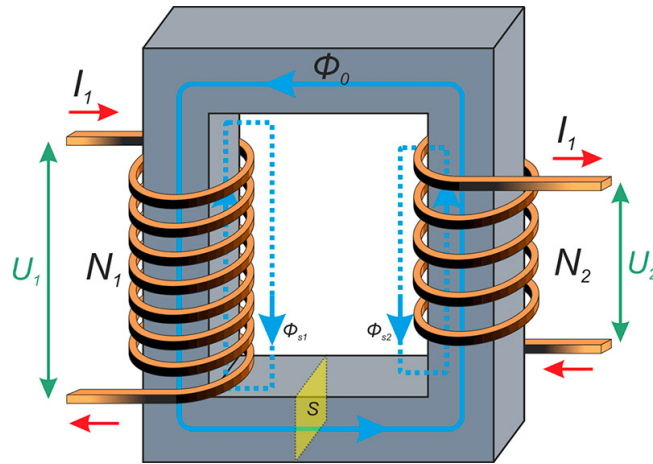
Рис. 11.17. Принципова схема трансформатора (знак «мінус» означає протилежність фаз). Відношення
