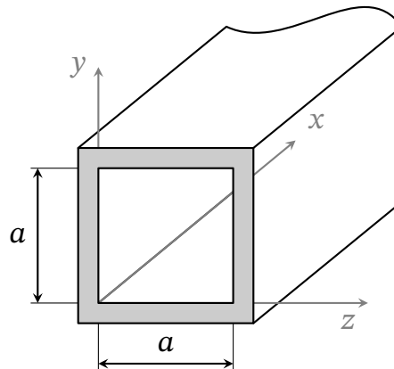
Рис. 18.1. Прямокутний хвильовід
