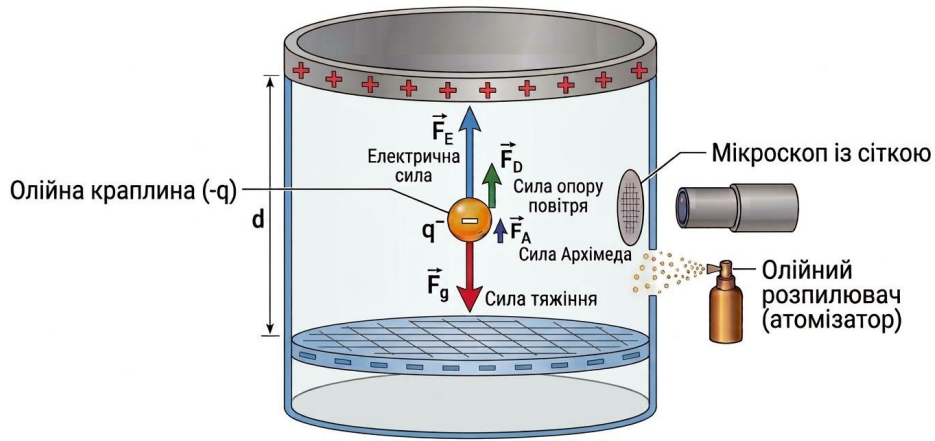
Рис. 10.7. Схема установки Міллікена для вимірювання заряду електрона (сила qE вказана для випадку q < 0 ).
