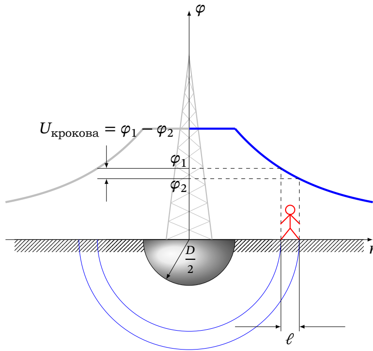
Рис. 7.14. Розтікання струму від напівсферичного заземлювача та крокова напруга нескінченності ( C_2 \rightarrow \infty , тобто 1/C \rightarrow 1/C_1 )
