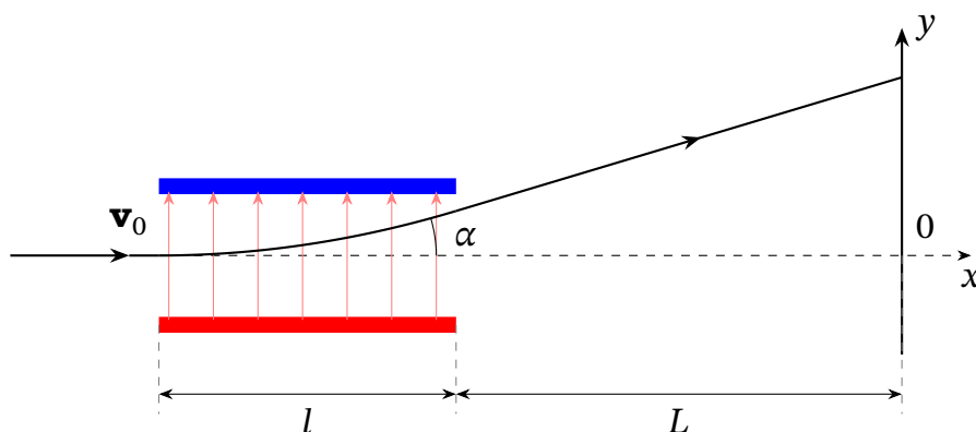
Рис. 10.5. Відхилення зарядженої частинки електричним полем конденсатора. К — конденсатор, Е — екран.
