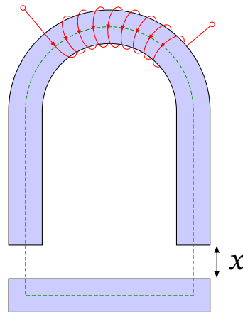
Рис. 11.20. Електромагніт з якорем, відокремленим повітряним зазором x
