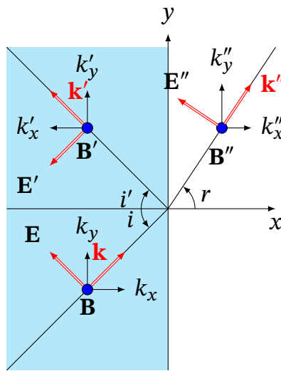
Рис. 14.9. Падаюча, відбита й заломлена p -поляризовані хвилі на межі розділу двох діелектриків
