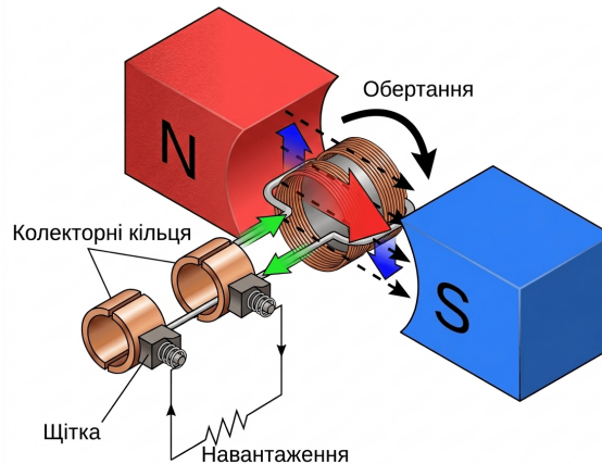
Рис. 11.4. Схема найпростішого генератора змінного струму
