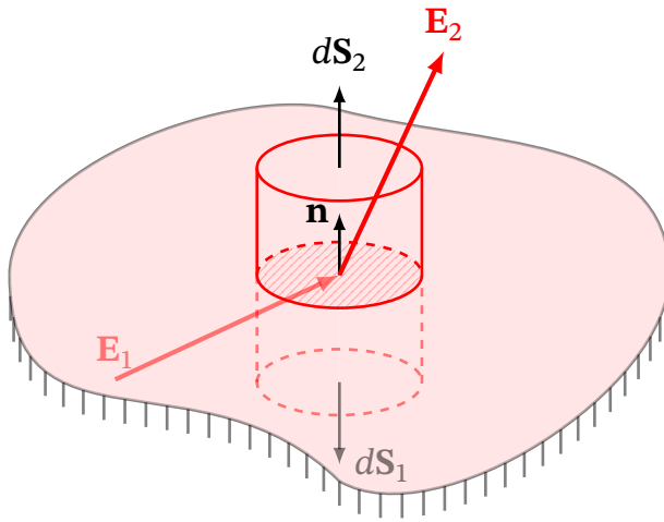
Рис. 1.32. До виведення першої граничної умови
