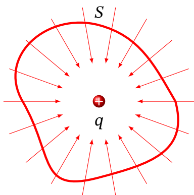
Рис. 1.17. До теореми Ерншоу
