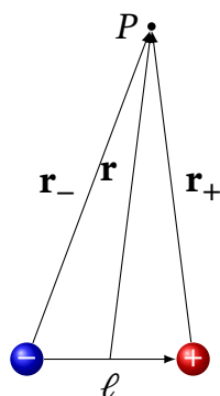
Рис. 1.14. До виведення напруженості поля диполя
