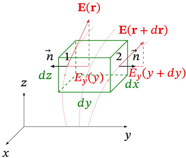
Рис. 1.18. До виведення диференціальної форми теореми Гаусса
