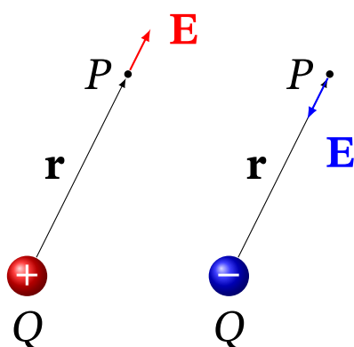
Рис. 1.6. Напруженість поля точкового заряду Q в точці спостереження P . Для додатного і від'ємного зарядів напрямки вектора напруженості \mathbf{E} відрізняються.
