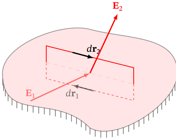
Рис. 1.33. До виведення другої граничної умови
