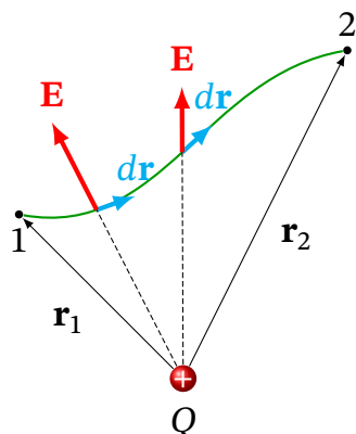
Рис. 1.21. До виведення роботи сил поля по переміщенню пробного заряду.
