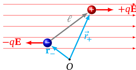
Рис. 1.15. до виведення моменту сил, що діє на диполь в однорідному електричному полі
