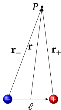
Рис. 1.28. До виведення потенціалу диполя.
