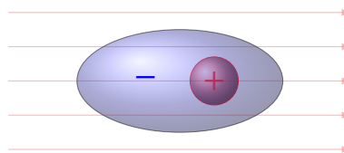
Рис. 1.13. Дипольний момент виник під дією зовнішнього поля p \neq 0 .
