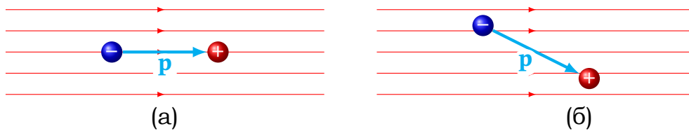
Рис. 1.31. Положення диполя в однорідному електричному полі. Ліворуч (а) — положення стійкої рівноваги з мінімальною енергією. Праворуч (б) — нестійке положення.
