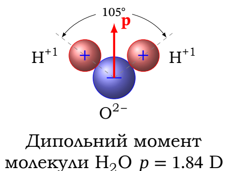
Рис. 1.11. ілюстрація дипольних моментів деяких полярних молекул
