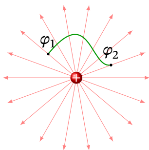
Рис. 1.22. До задачі виведення різниці потенціалів
