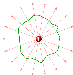
Рис. 1.23. До поняття циркуляції вектора \mathbf{E}
