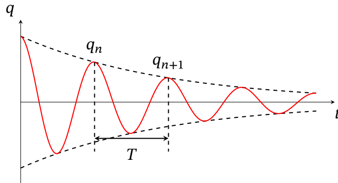
Рис. 15.3. Затухаючі коливання. До означення логарифмічного декременту.
