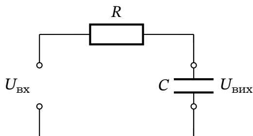
Рис. 15.12. Фільтр низьких частот: вихідна напруга знімається з конденсатора C .
