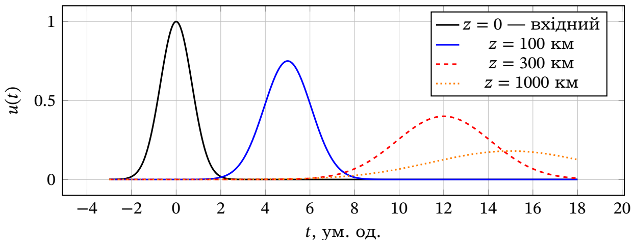
Рис. 16.3. Дисперсійне спотворення гаусового імпульсу при поширенні в лінії з втратами. З відстанню імпульс розширюється і зменшується за амплітудою — саме ця проблема мучила перші трансатлантичні кабелі.
