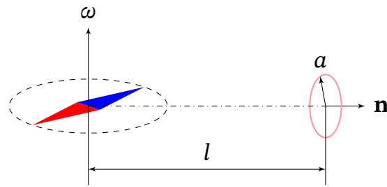
Рис. 10.16. Магнітний диполь, що обертається, і нерухоме кільце на відстані \ell
