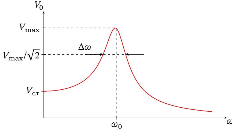
Рис. 15.6. Характеристики резонансної кривої: V_{\text{max}} — максимум амплітуди, V_{\text{ст}} — статична амплітуда, \Delta\omega — ширина резонансу.
