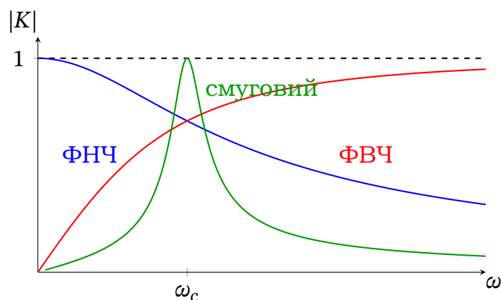
Рис. 15.15. Амплітудно-частотні характеристики трьох фільтрів: ФНЧ (синій), ФВЧ (червоний) і смугового (зелений). Для смугового прийнято Q = 5 .
