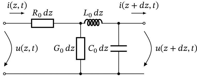
Рис. 16.1. Схема заміщення елементарного відрізка довгої лінії як чотириполюсника. Паралельні елементи G_0 dz і C_0 dz рознесені для наочності.
