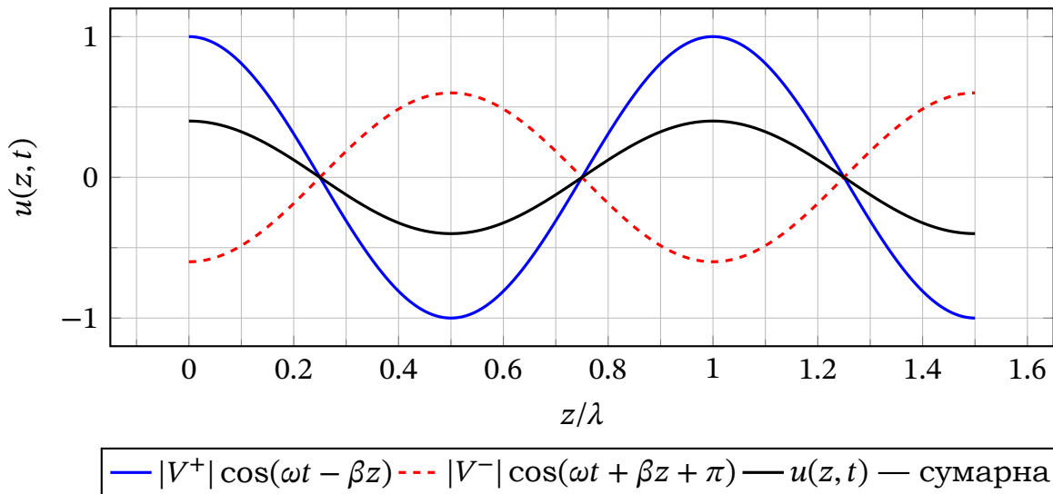
Рис. 16.2. Інтерференція падаючої та відбитої хвиль у лінії без втрат при |V^-|/|V^+| = 0.6 . Сумарна напруга утворює стоячу хвилю з вузлами та пучностями. Коефіцієнт стоячої хвилі КСХ = (1 + 0.6)/(1 - 0.6) = 4 .
