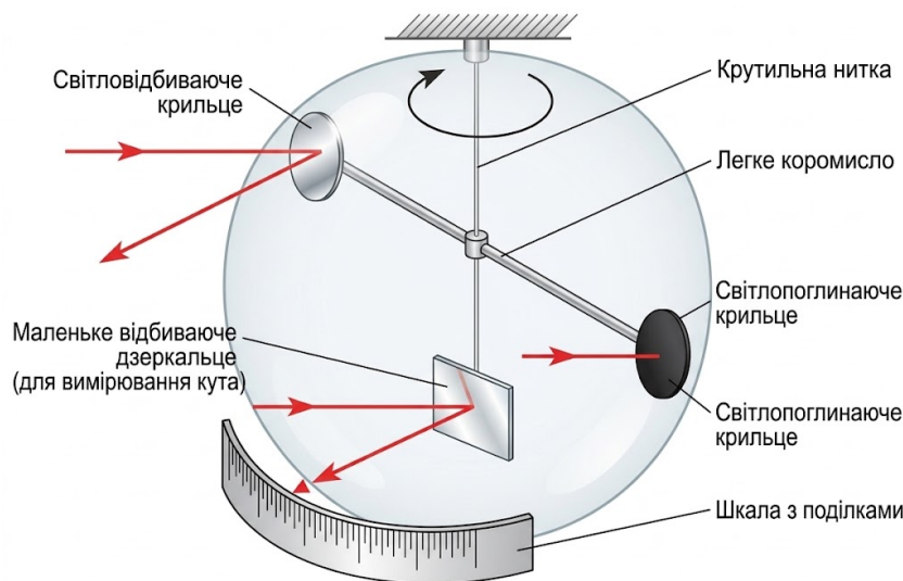
Рис. 13.6. Схема дослідів П. М. Лебедєва (1899 р.) з вимірювання тиску світла
