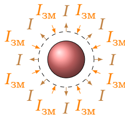
Рис. 11.3. Радіальне стікання заряду з кулі: струм провідності I і струм зміщення I_{\text{зм}}
