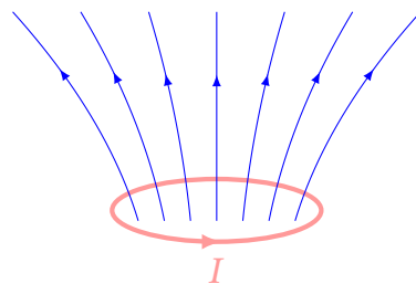
Рис. 10.10. Контур зі струмом I і створюване ним власне магнітне поле
