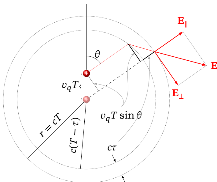
Рис. 14.4. Геометрія зламу силової лінії: розкладання поля на поздовжню E_{\parallel} і поперечну E_{\perp} складові
