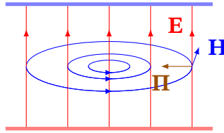
Рис. 11.8. Поля \mathbf{E} , \mathbf{H} і вектор Пойнтінга \mathbf{\Pi} при зарядці плоского конденсатора
