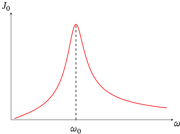
Рис. 15.8. Залежність амплітуди коливань струму від частоти коливань ЕРС — резонанс напруги на конденсаторі і ЕРС в послідовному LCR-контурі (рис. 15.1).
