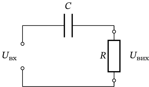
Рис. 15.13. Фільтр високих частот: вихідна напруга знімається з резистора R .
