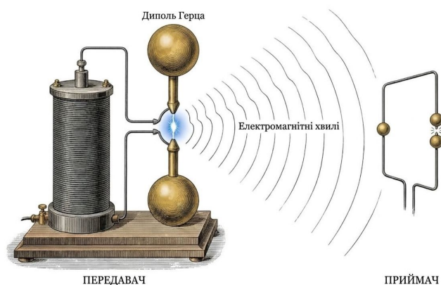
Рис. 14.1. Вібратор Герца.
