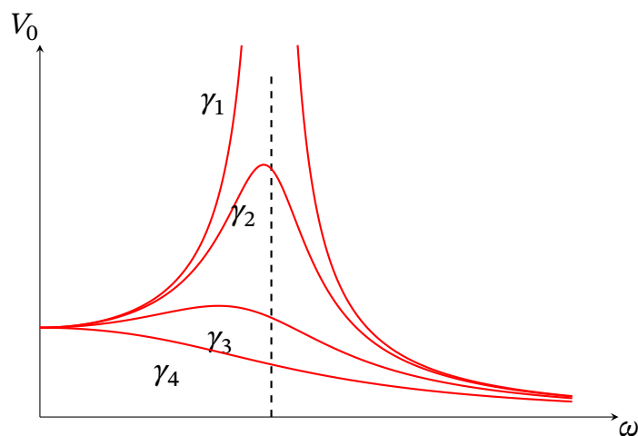
Рис. 15.4. Амплітудно-частотна характеристика контуру. Залежність амплітуди вимушених коливань V_0 від частоти \omega зовнішньої ЕРС.
