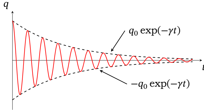
Рис. 15.2. Графік затухаючих коливань. Штриховою лінією показано часову залежність амплітуди A(t) = q_0 e^{-\gamma t} .
