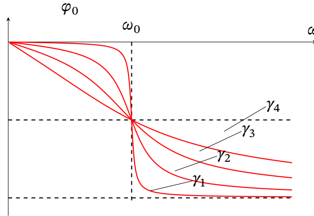
Рис. 15.5. Фазово-частотна характеристика контуру. Залежність фазового зсуву \varphi_0 від частоти \omega зовнішньої ЕРС.
