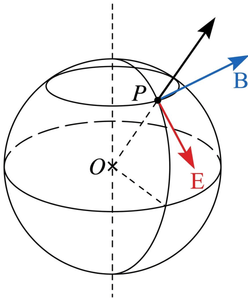
Рис. 14.6. Поля E_\theta і B_\varphi у хвильовій зоні диполя
