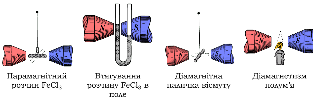
Рис. 10.21. Поведінка пара- й діамагнітних речовин у неоднорідному магнітному полі
