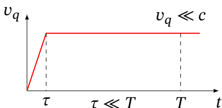
Рис. 14.2. Швидкість заряду: короткий імпульс прискорення тривалістю \tau , після якого заряд рухається рівномірно
