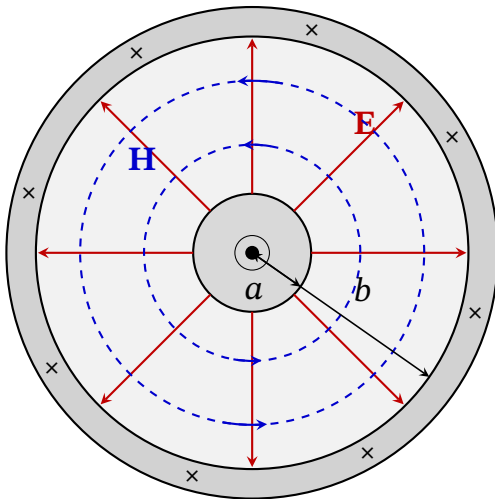
Рис. 16.4. Структура електромагнітного поля в поперечному перерізі довгої лінії (коаксіального кабелю): вектор \mathbf{E} направлений від внутрішньої жили до зовнішнього екрана, а лінії вектора \mathbf{H} охоплюють провідник зі струмом.
