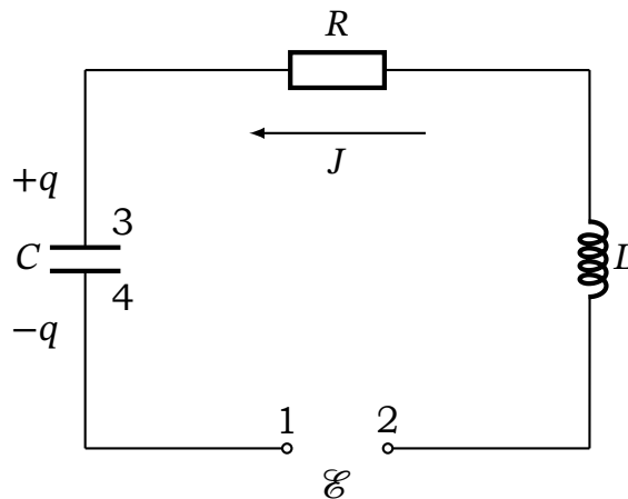
Рис. 15.1. Контур, що включає конденсатор, індуктивність, опір R і стороннє джерело ЕРС \mathcal{E} .
