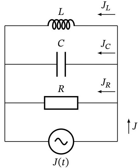
Рис. 15.9. Паралельний LCR -контур, що включає джерело заданого змінного струму J(t) = J_0 \cos \omega t .
