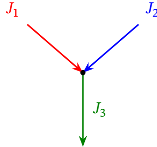
Рис. 15.10. Перше правило Кірхгофа: сума струмів, що входять у вузол, рівна нулю.
