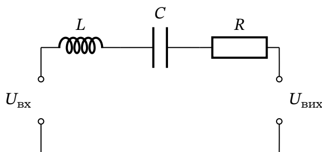
Рис. 15.14. Смуговий фільтр на основі послідовного LCR -контур: вихідна напруга знімається з резистора R .
