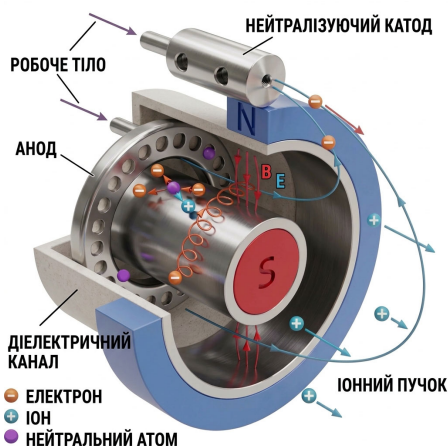
Рис. 10.6. Схема холлівського двигуна.
