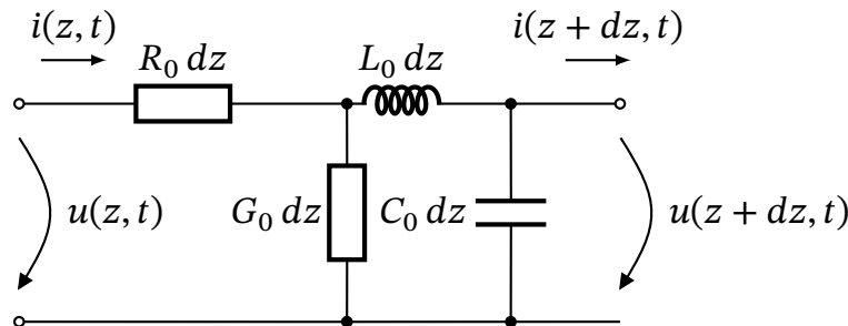
Рис. 17.1. Схема заміщення елементарного відрізка довгої лінії як чотириполосника. Паралельні елементи G_0 dz і C_0 dz рознесені для наочності.
