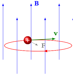
Рис. 10.1. Обертальний рух частинки із зарядом q > 0 навколо напрямку магнітного поля.
