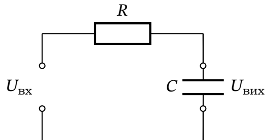
Рис. 16.12. Фільтр низьких частот: вихідна напруга знімається з конденсатора C .
