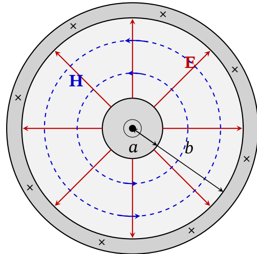
Рис. 17.4. Структура електромагнітного поля в поперечному перерізі довгої лінії (коаксiального кабелю): вектор \mathbf{E} напрямлений від внутрішньої жили до зовнішнього екрана, а лінії вектора \mathbf{H} охоплюють провідник зі струмом.
