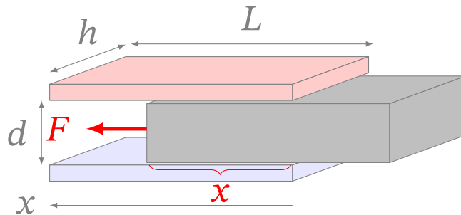
Рис. 6.6. Модель конденсатора з частково всунутою пластиною діелектрика: паралельне з'єднання вакуумного та заповненого діелектриком конденсаторів
