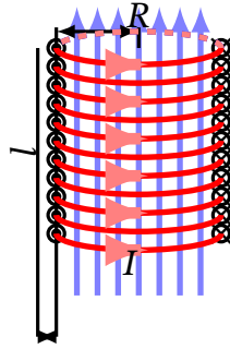
Рис. 10.18. Поздовжній переріз довгого соленоїда: однорідне поле всередині, струм у витках обмотки
