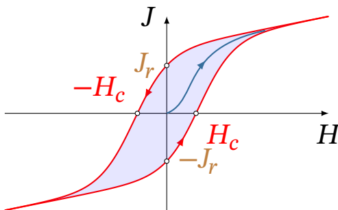
Рис. 9.11. Петля гістерезису ферромагнетика: J_r — залишкова намагніченість, H_c — коерцитивна сила
