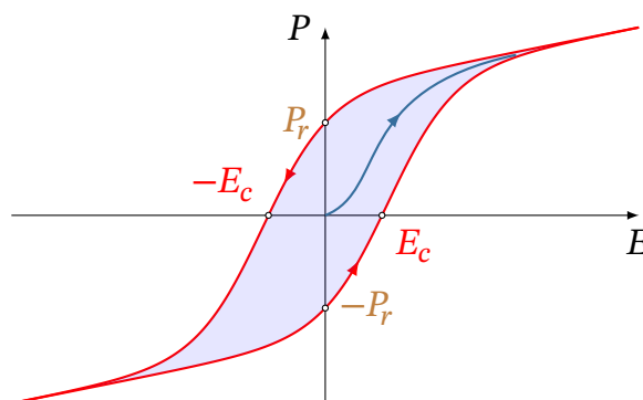
Рис. 5.15. Петля гістерезису сегнетоелектрика: P_r — залишкова поляризація, E_c — коерцитивна сила
