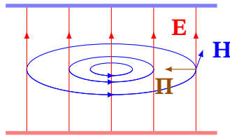
Рис. 11.8. Поля \mathbf{E} , \mathbf{H} і вектор Пойнтінга \mathbf{\Pi} при зарядці плоского конденсатора
