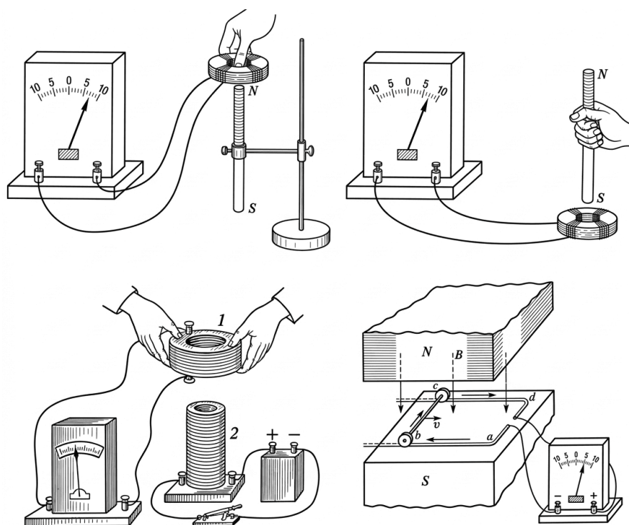
Рис. 10.2. Схема класичних дослідів Фарадея з електромагнітної індукції Знак «мінус» у цьому законі — не формальність, а прояв правила Ленца , з яким ми детальніше познайомимось нижче.
