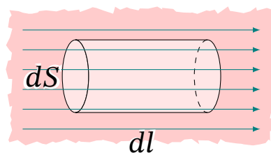
Рис. 7.5. Елементарний циліндр струму до виведення диференціальної форми закону Ома
