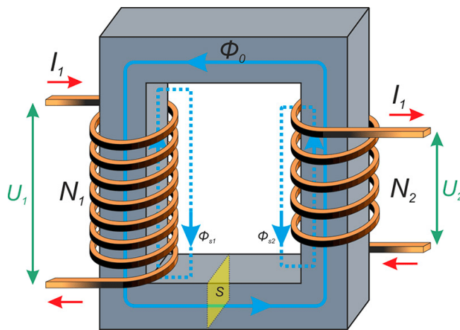
Рис. 10.17. Принципова схема трансформатора
