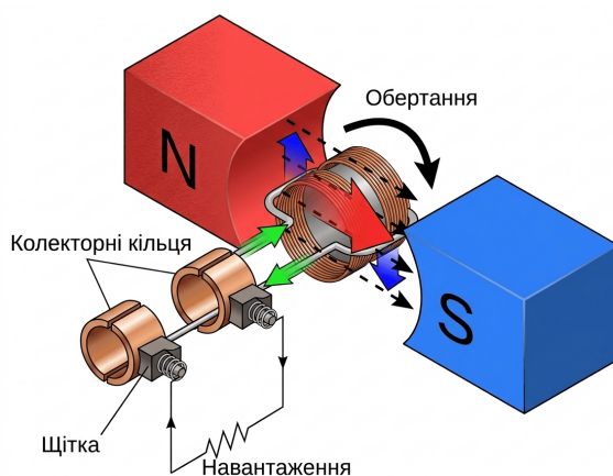
Рис. 10.4. Схема найпростішого генератора змінного струму
