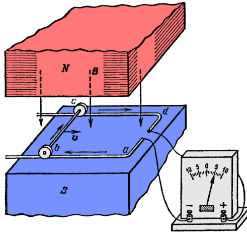
Рис. 10.3. Виникнення ЕРС індукції за рахунок руху перемички bc
