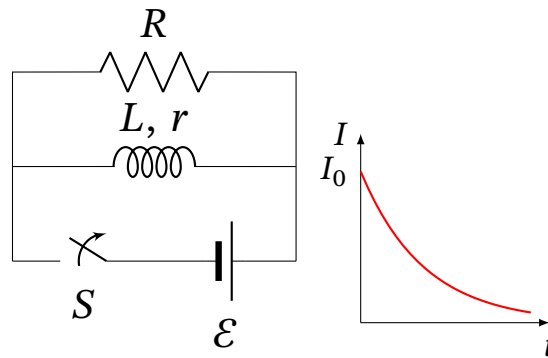
Рис. 10.13. Екстраструм розмикання в колі з індуктивністю
