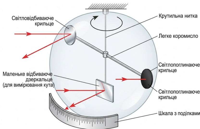
Рис. 13.6. Схема досліду П. М. Лебедева (1899 р.) з вимірювання тиску світла
