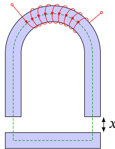
Рис. 10.20. Електромагніт з якорем, відокремленим повітряним зазором x
