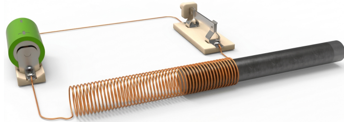
Рис. 10.19. Осердя втягується в котушку зі струмом — приклад пондеромоторної сили в магнітному полі
