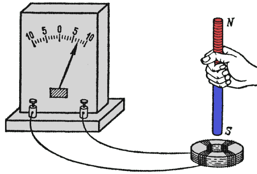
Рис. 10.5. ЕРС індукції в нерухомому контурі за рахунок зміни поля \mathbf{B}
