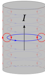
Рис. 11.11. Якісний механізм скін-ефекту: вихрові струми Фуко підсилюють струм на поверхні й послаблюють у центрі провідника
