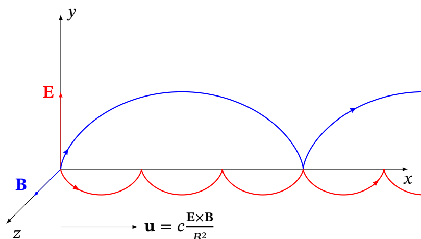
Рис. 12.4. Траєкторія частинки у взаємно перпендикулярних полях \mathbf{B} і \mathbf{E} за умови, що початкова швидкість дорівнює нулю.
