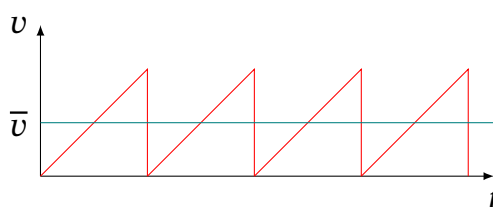
Рис. 7.6. Пілкоподібна залежність швидкості електрона від часу в моделі Друде
