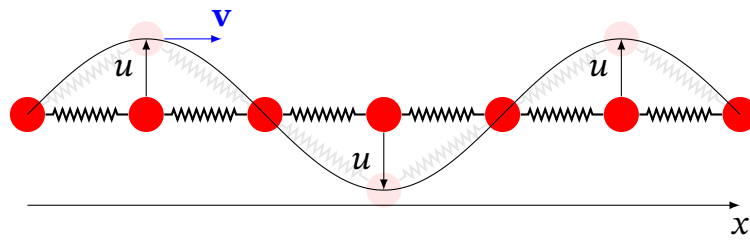
Рис. 13.1. Механічна хвиля в ланцюжку зв'язаних пружинками тягарців — наочна модель для розуміння хвильового процесу
