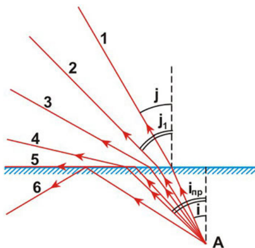
Рис. 13.10. Заломлений промінь наближається до поверхні розділу при зростанні кута падіння
