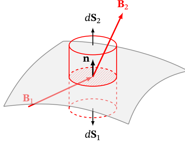
Рис. 9.5. Циліндр Гаусса на межі розділу двох магнетиків
