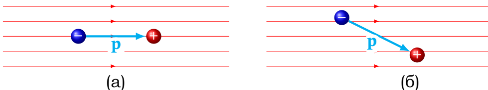
Рис. 3.9. Положення диполя в однорідному електричному полі. Ліворуч (а) — положення стійкої рівноваги з мінімальною енергією. Праворуч (б) — нестійке положення.
