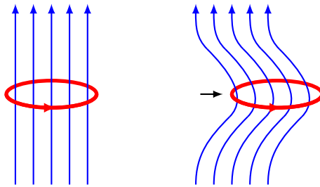
Рис. 10.8. «Вморожування» силових ліній магнітного поля в надпровідний контур
