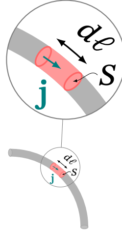
Рис. 8.3. Елемент лінійного струму I d\boldsymbol{\ell} : збільшений фрагмент показує напрям \mathbf{j} уздовж осі провідника перерізу S
