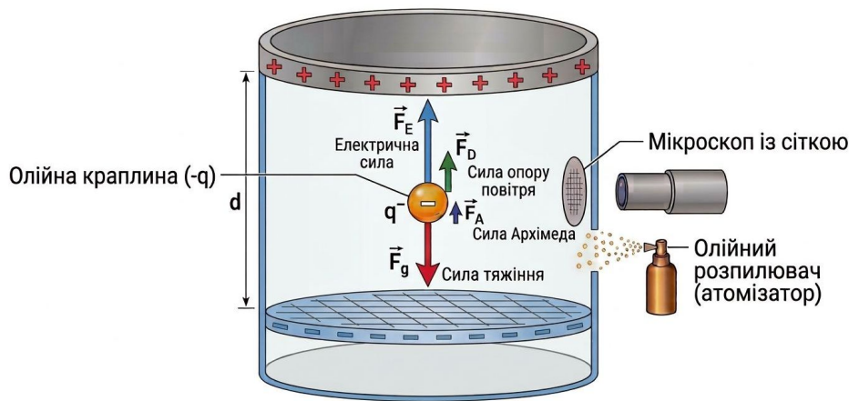
Рис. 12.7. Схема установки Міллікена для вимірювання заряду електрона (сила qE вказана для випадку q < 0 ).
