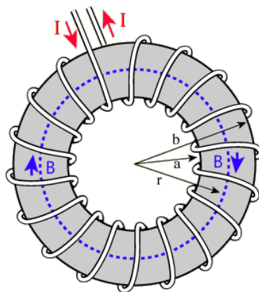
Рис. 10.11. Тороїдальна котушка
