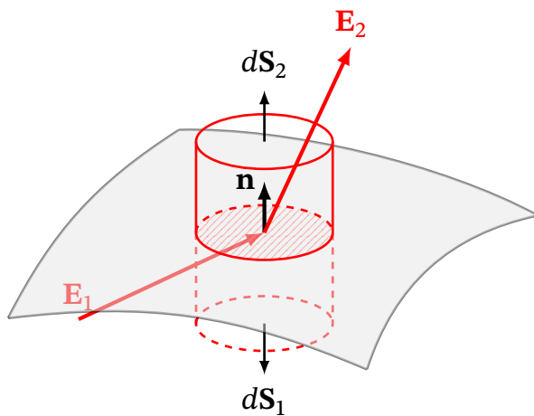
Рис. 2.20. До виведення першої граничної умови
