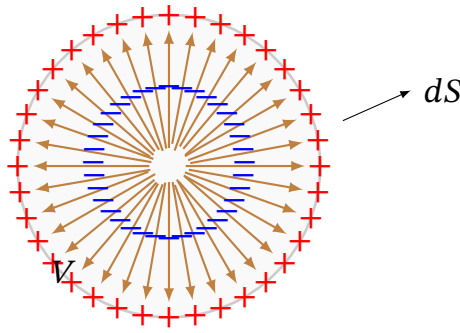
Рис. 5.7. Довільний об'єм неоднорідно поляризованого діелектрика: на поверхні виступають некомпенсовані зв'язані заряди виділеного об'єму:
