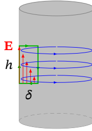
Рис. 11.12. Контур для оцінки циркуляції E поблизу поверхні провідника
