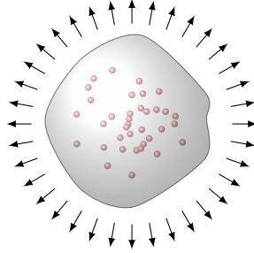
Рис. 11.7. Заряджені частинки в області, обмеженій замкненою поверхнею: енергія електромагнітного поля може втікати й витікати крізь цю поверхню
