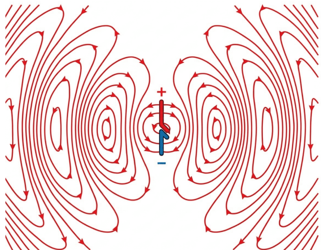
Рис. 14.7. Електричне поле осцилюючого диполя: у ближній зоні поле ніби «причеплене» до диполя, у хвильовій — випромінюється
