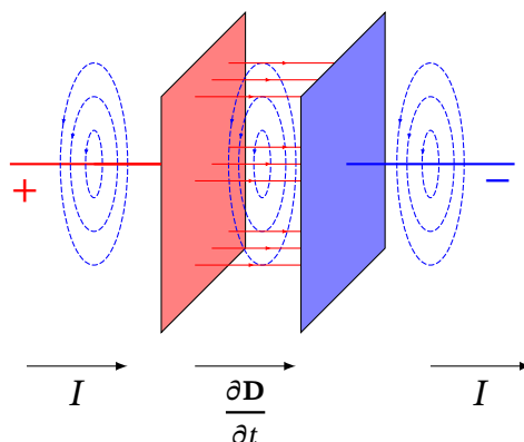
Рис. 11.5. Магнітне поле, створене струмом зміщення всередині конденсатора під час його зарядки
