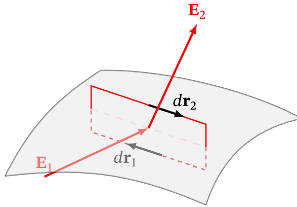
Рис. 5.10. Контур циркуляції на межі розділу двох середовищ для виведення граничної умови на тангенціальну складову \mathbf{E}
