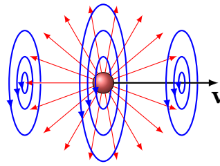
Рис. 8.2. Заряд, що рухається зі швидкістю \mathbf{v} , є джерелом як електричного, так і магнітного поля
