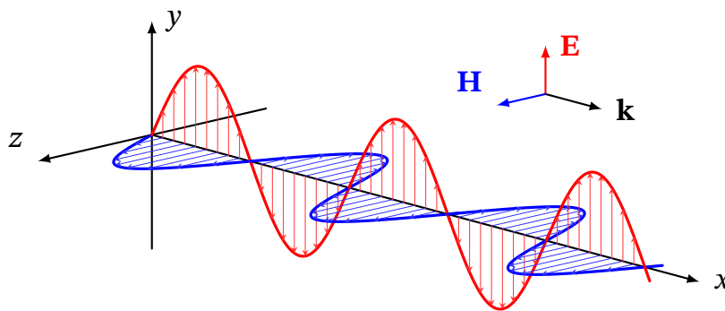
Рис. 13.4. Плоска монохроматична електромагнітна хвиля: взаємно перпендикулярні коливання \mathbf{E} і \mathbf{H} , що поширюються вздовж \mathbf{k}
