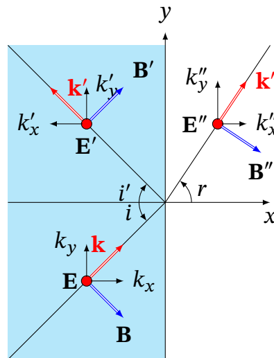
Рис. 13.8. Падаюча, відбита й заломлена s-поляризовані хвилі на межі розділу двох діелектриків
