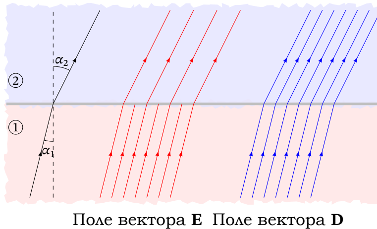
Рис. 5.11. Заломлення силових ліній \mathbf{E} і \mathbf{D} на межі розділу двох діелектриків
