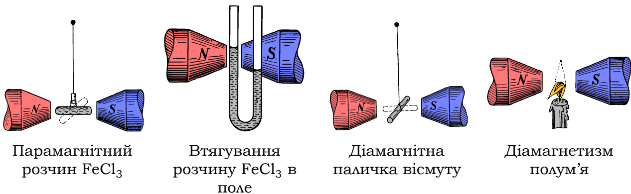
Рис. 10.21. Поведінка пара- й діамагнітних речовин у неоднорідному магнітному полі
