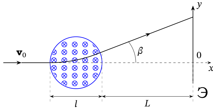
Рис. 12.6. Відхилення зарядженої частинки магнітним полем. М — магніт, Е — екран. Напрямок магнітного поля перпендикулярно площині листа і напрямлено «за лист».
