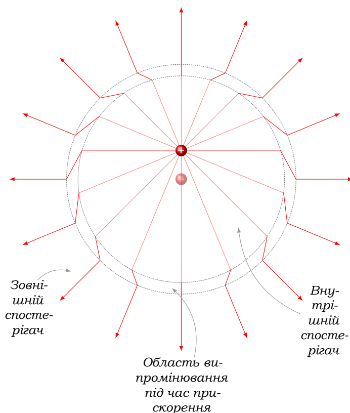
Рис. 14.3. Заломлені («злами») силові лінії поля короткочасно прискореного заряду: межа між «старим» і «новим» полем
