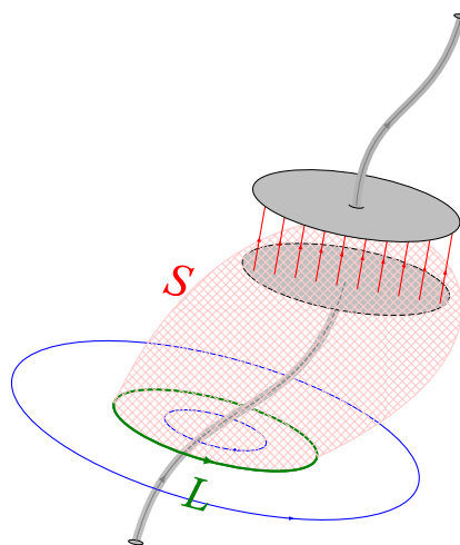
Рис. 11.2. Контур L , натягнута на нього поверхня S та провідник зі струмом, що її пронизує
