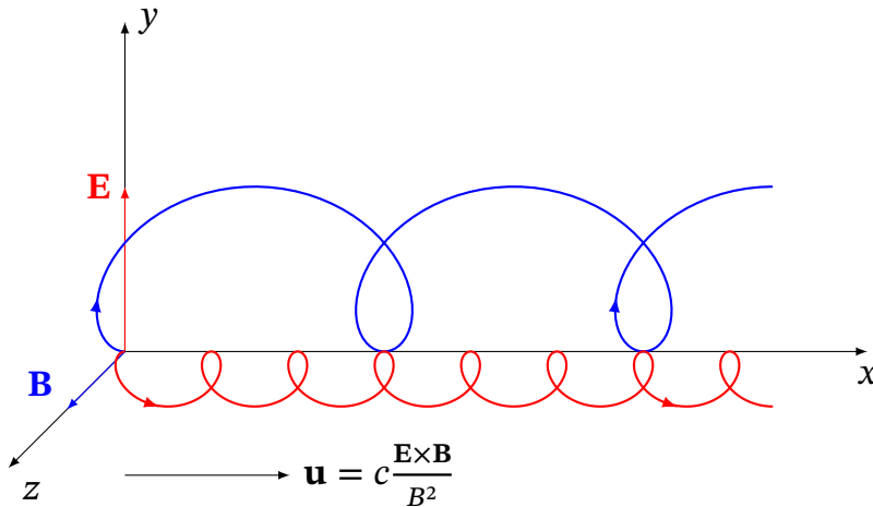
Рис. 12.3. Електричний дрейф додатно (синя крива) та від'ємно (червона крива) заряджених частинок.
