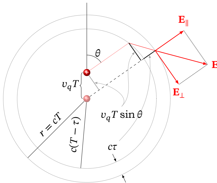
Рис. 14.4. Геометрія зламу силової лінії: розкладання поля на поздовжню E_{\parallel} і поперечну E_{\perp} складові
