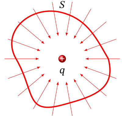
Рис. 2.10. До теореми Ерншоу
