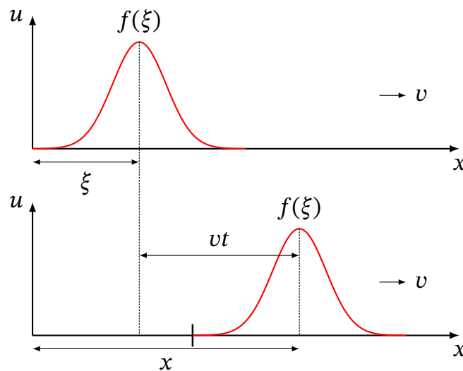
Рис. 13.2. Збурення, що поширюється без зміни форми зі швидкістю v : профіль у момент t — це профіль у момент 0, зсунутий на vt
