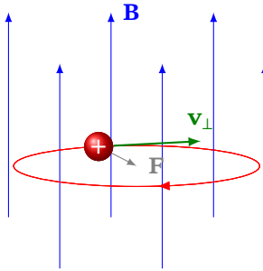
Рис. 8.5. Кругова траєкторія зарядженої частинки в однорідному магнітному полі: сила завжди перпендикулярна до швидкості
