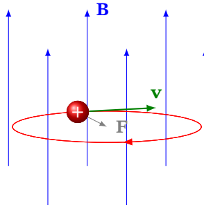
Рис. 12.1. Обертальний рух частинки із зарядом q > 0 навколо напрямку магнітного поля.
