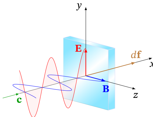
Рис. 13.5. Механізм виникнення тиску електромагнітної хвилі: сила Ампера d\mathbf{f} , що діє на струм, збуджений полем \mathbf{E} , у полі \mathbf{B}
