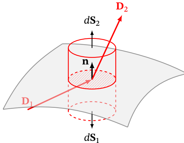
Рис. 5.9. Циліндр Гаусса на межі розділу двох середовищ для виведення граничної умови на нормальну складову D
