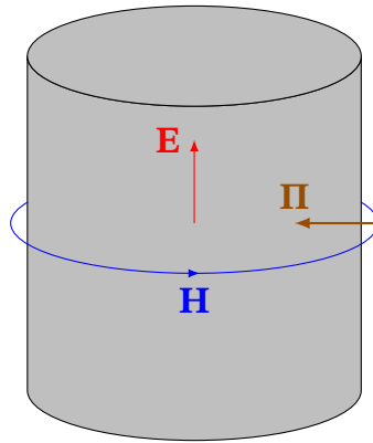
Рис. 11.9. Поля \mathbf{E} , \mathbf{H} і вектор Пойнтінга \mathbf{\Pi} на поверхні довгого провідника зі струмом
