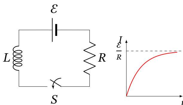
Рис. 10.12. Встановлення струму в колі з індуктивністю після замикання ключа
