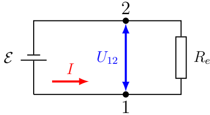
Рис. 3.1. Електричне коло
