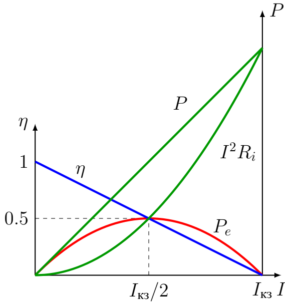
Рис. 3.3. Діаграма режимів роботи джерела електроенергії
