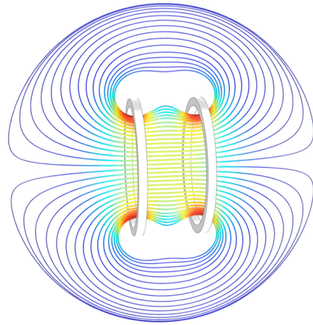
Рис. 4.3. Видяг поля котушок Гельмгольца (взято з https://www.freepng.ru/png-d02278/ )
