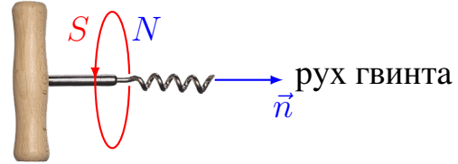
Рис. 4.1. Полюса витка
