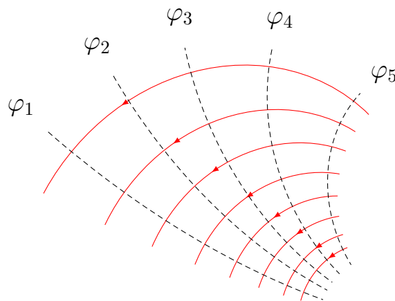
Рис. 2.4. Вектор \vec{E} спрямований у кожній точці по нормалі до еквіпотенціальної поверхні у бік зменшення потенціалу \varphi : \varphi_1 < \varphi_2 < \varphi_3 < \varphi_4 < \varphi_5
