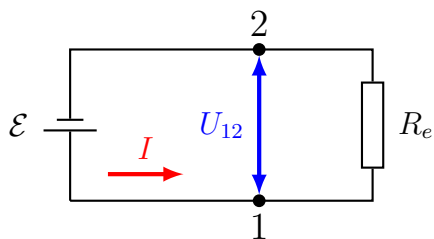
Рис. 3.1. Електричне коло
