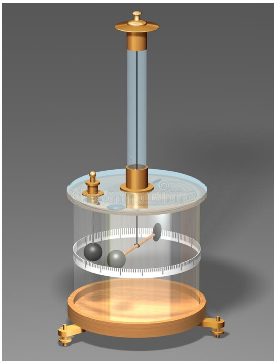
Рис. 1.3. Крутильні терези
