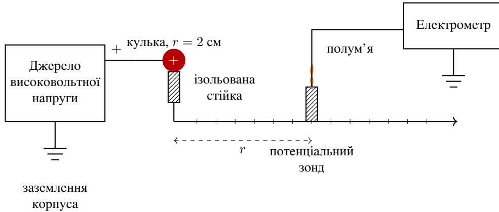
Рис. 2.8. Принципова схема установки: заряджена кулька з'єднана з джерелом високовольтної напруги; потенціальний зонд із пальником переміщують уздовж лінійки на різні відстані r від центра кульки та з'єднують із входом електрометра; корпуси джерела й електрометра заземлені
