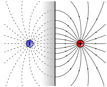
Рис. 1.2. Заряд та його зображення в заземленій металевій пластині
