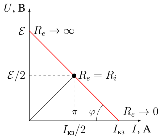
Рис. 3.5. Характеристика джерела із сталим внутрішнім опором R_i .
