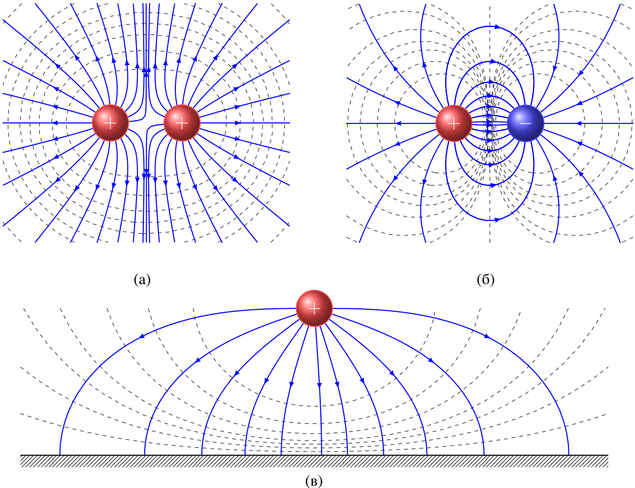
Рис. 2.5. Картини силових ліній (суцільні сині лінії) та еквіпотенціальних поверхонь (штрихові сині лінії) для різних конфігурацій полів: а) двох однойменних зарядів; б) двох різнойменних зарядів; в) заряду над заземленою провідною площиною
