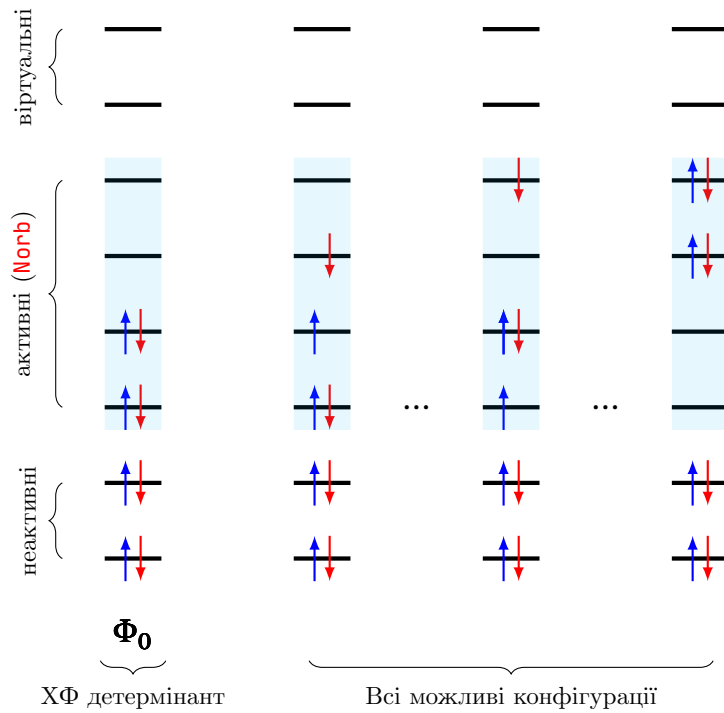
Рис. 5.3. Схема методу CASSCF: поділ орбіталей на остовні, активні та віртуальні, а також побудова повного СІ в активному просторі.
