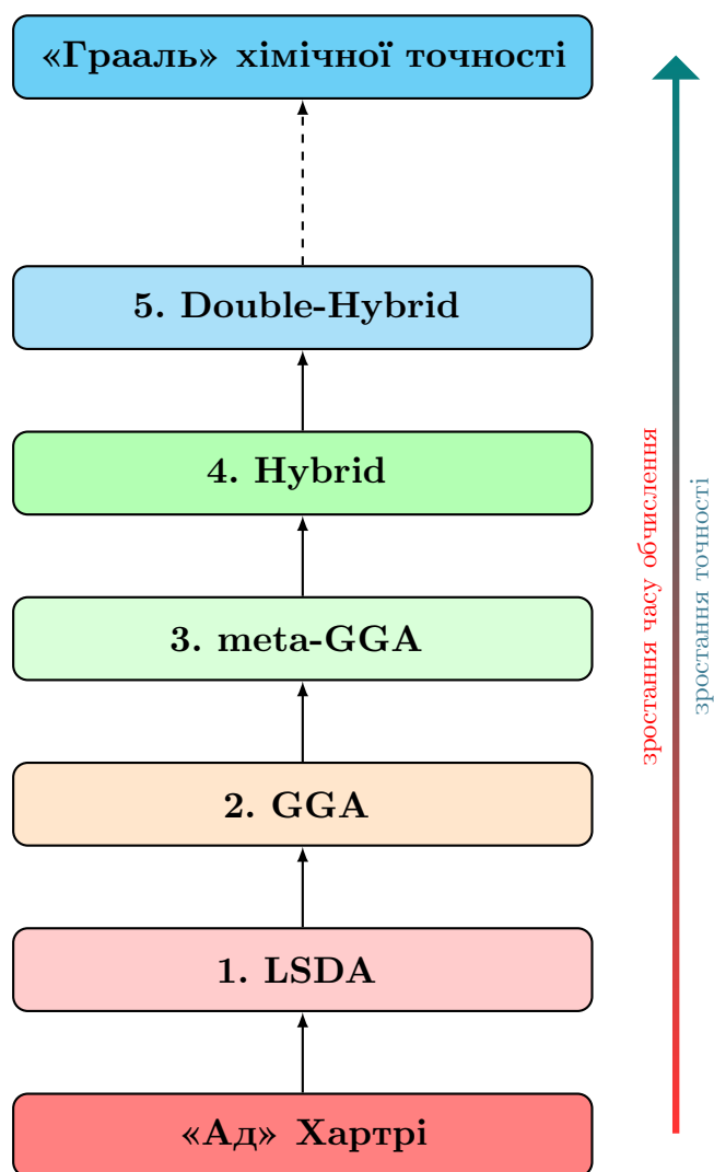
Рис. 1. Драмина Якова (Jacob's ladder) — класифікація обмінно-кореляційних функціоналів DFT.
