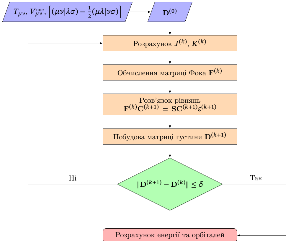
Рис. 3.1. Блок-схема SFC-процедури.
