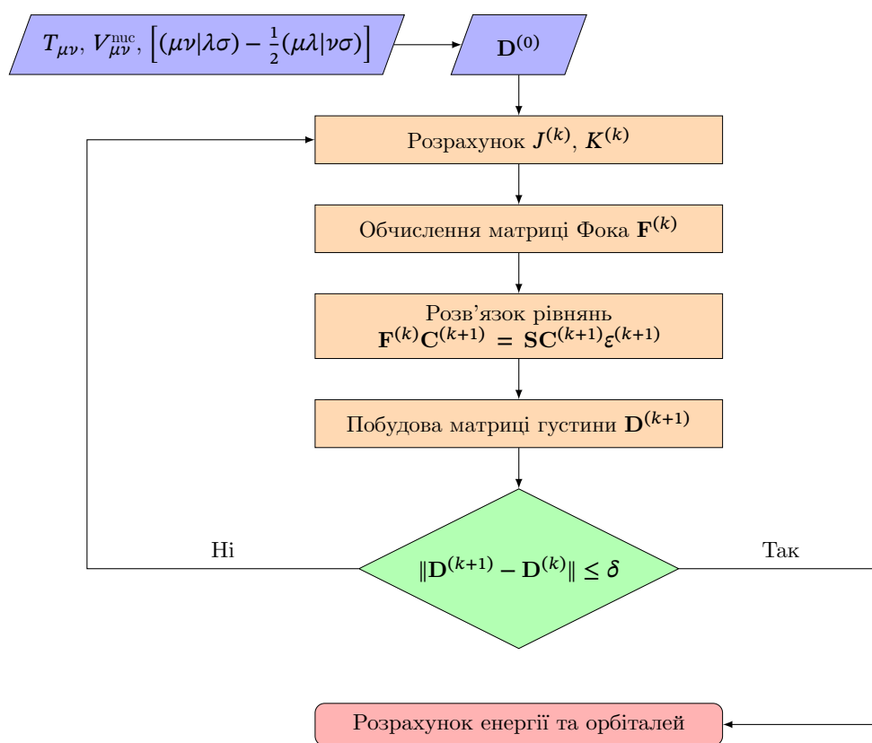
Рис. 3.1. Блок-схема SFC-процедури.
