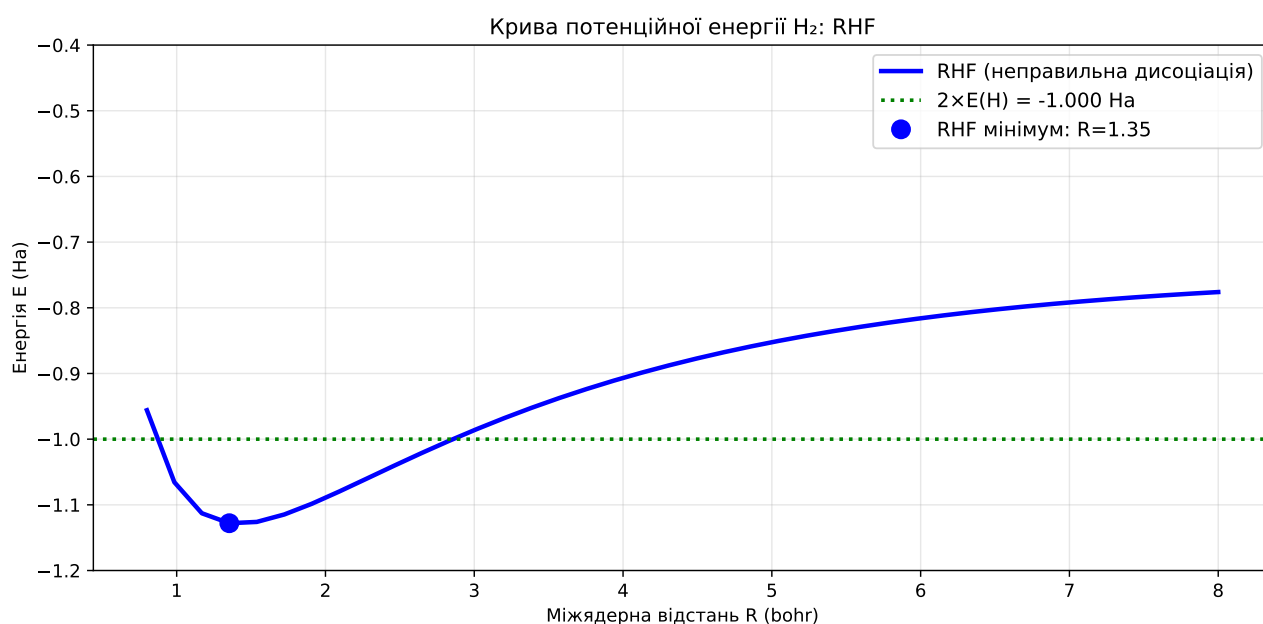
Рис. 4.2. Поверхня потенційної енергії молекули H_2 методом RHF. Однак RHF дає (рис. 4.2):
