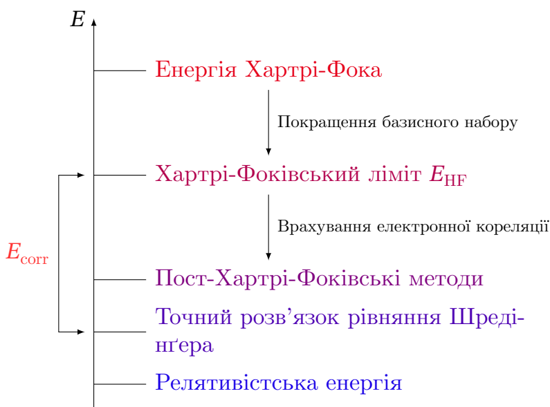
Рис. 5.1. Енергетична діаграма, що ілюструє внесок електронної кореляції ( E_{\text{corr}} ) у наближенні до точного розв'язку рівняння Шредінгера. Хартрі-Фоківський ліміт досягається при повному базисі, а пост-Хартрі-Фоківські методи враховують кореляцію електронів.
