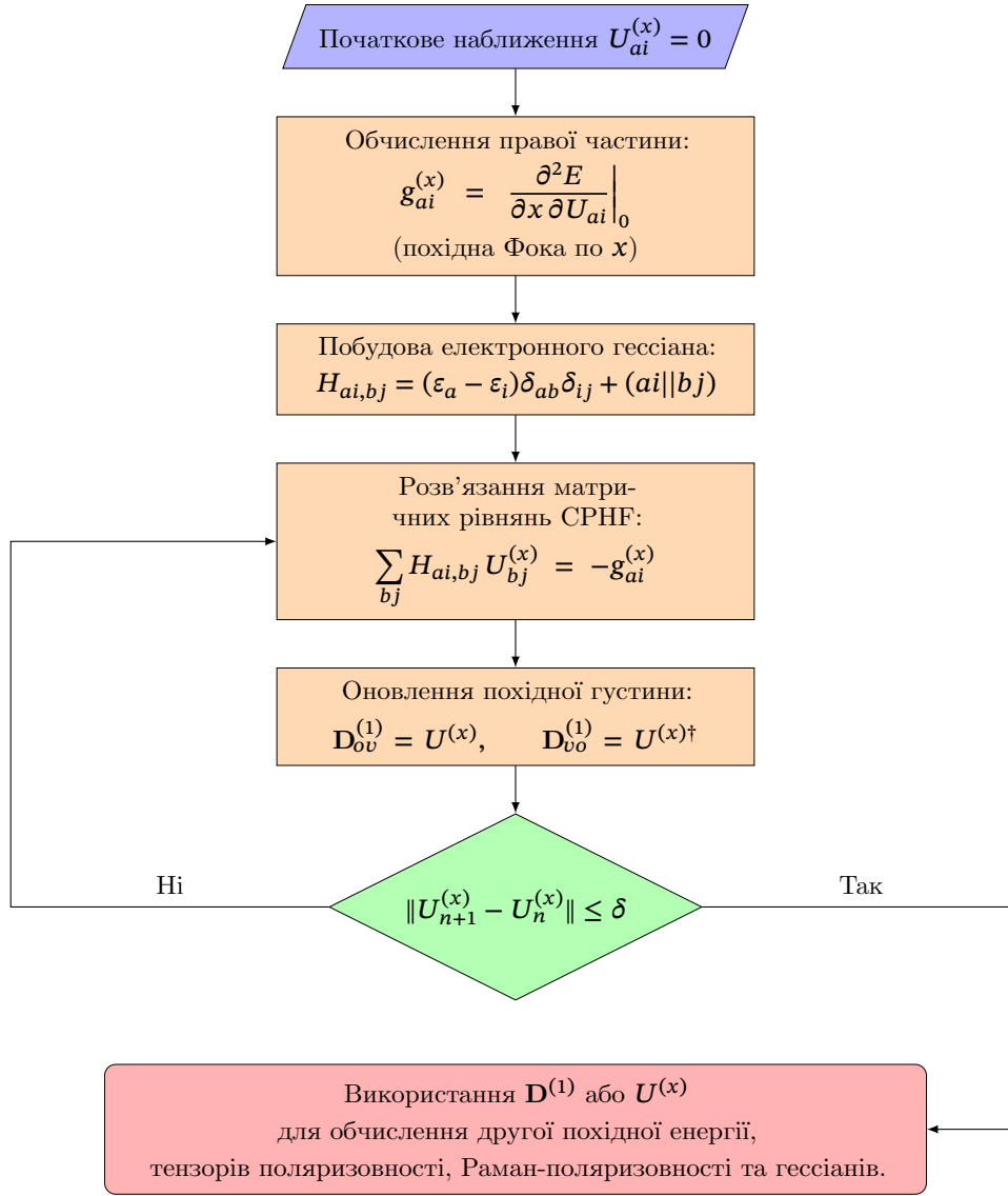
Рис. 1.1. Процедура розв'язку рівнянь СРHF.
