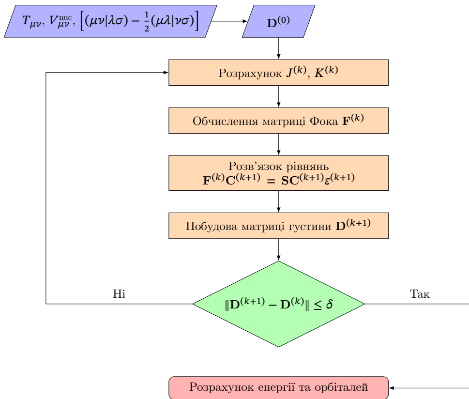
Рис. 3.1. Блок-схема SFC-процедури.
