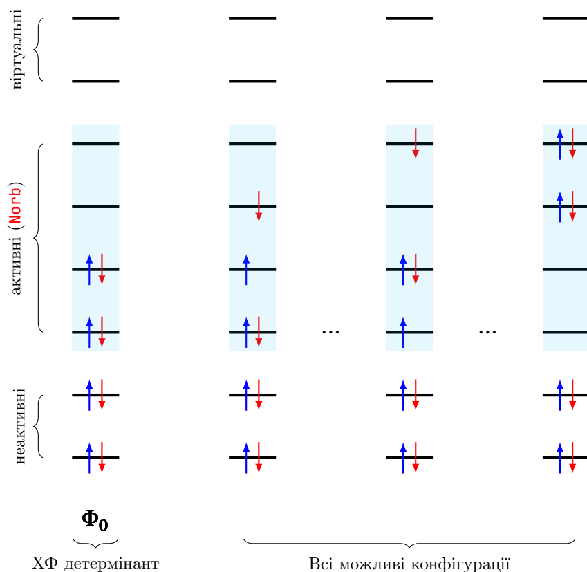
Рис. 5.3. Схема методу CASSCF: поділ орбіталей на основні, активні та віртуальні, а також побудова повного СІ в активному просторі.
