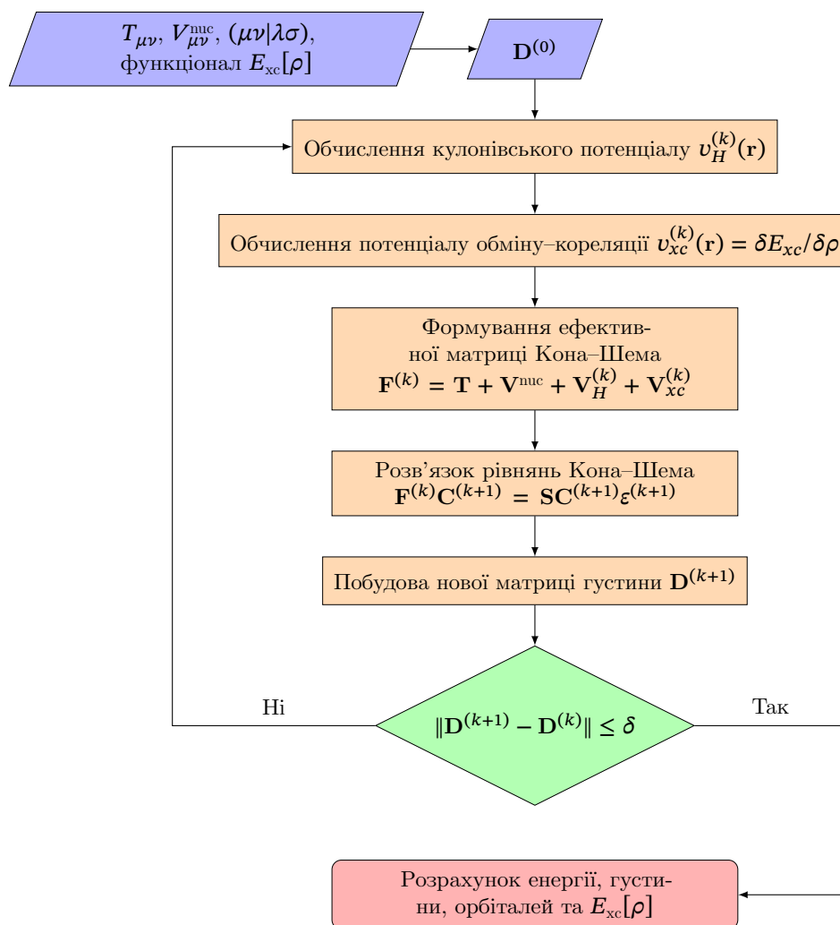
Рис. 6.1. Самозгоджений цикл Кона-Шема. На відміну від HF, тут замість матриць J і K будуються потенціали v_H та v_{xc} , які визначають ефективну матрицю Фока. і повторюють обчислення до досягнення самозгодженості. Це означає, що потенціал v_{\text{eff}}(\mathbf{r}) залежить від густини \rho(\mathbf{r}) , а сама густина — від орбіталей, знайдених у цьому ж потенціалі. Таким чином, розв'язання рівнянь Кона-Шема є ітераційним процесом (див. рис. 6.1).
