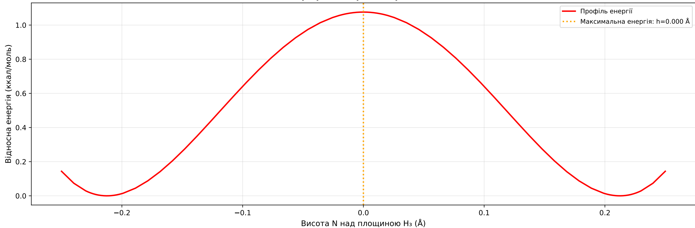
Профіль енергії інверсії NH 3
