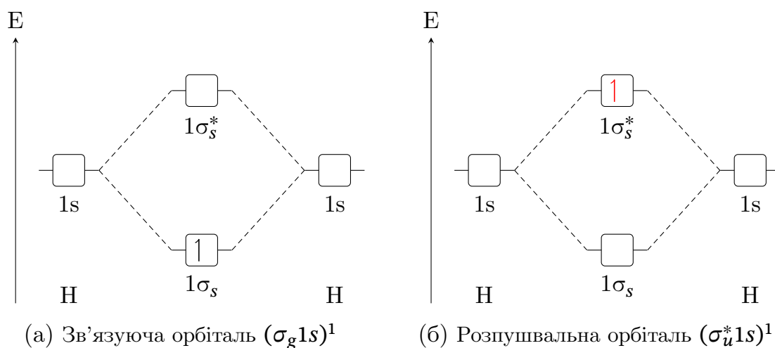
Рис. 4.2. Енергетична діаграма
