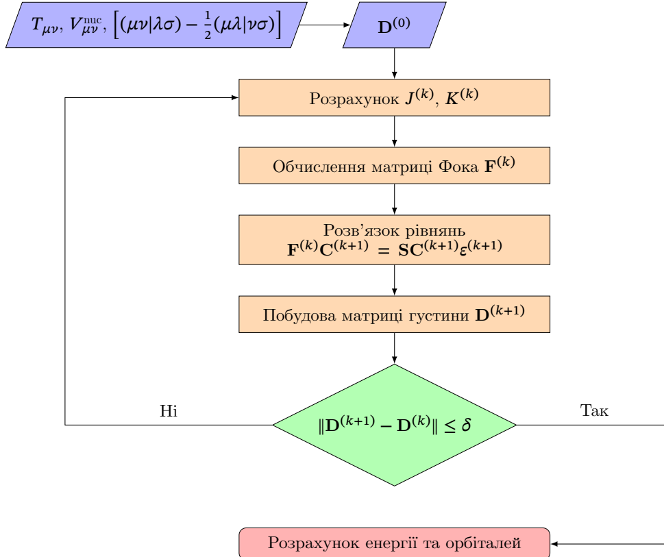
Рис. 3.1. Блок-схема SFC-процедури.
