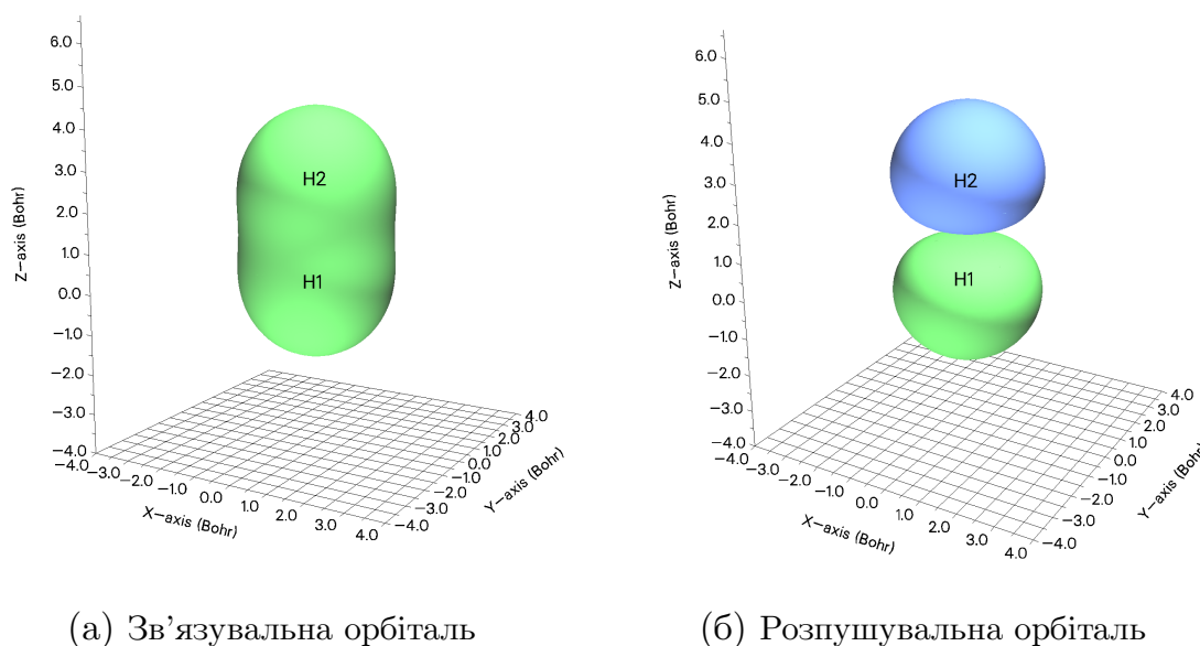
Рис. 4.4. Просторовий вигляд орбіталей
