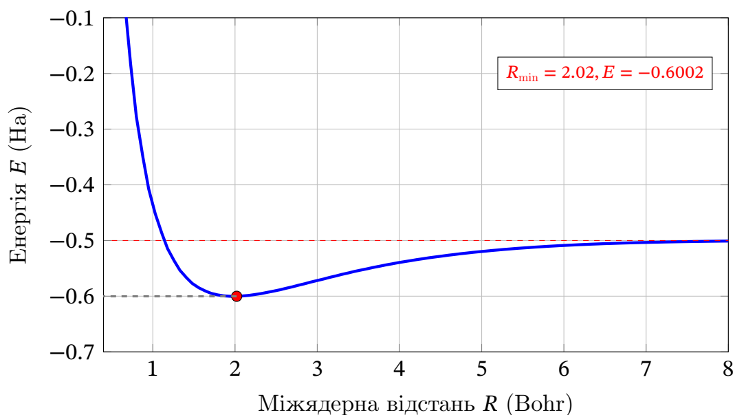
Рис. 4.2. Крива потенційної енергії (PES) для \text{H}_2^+ .
