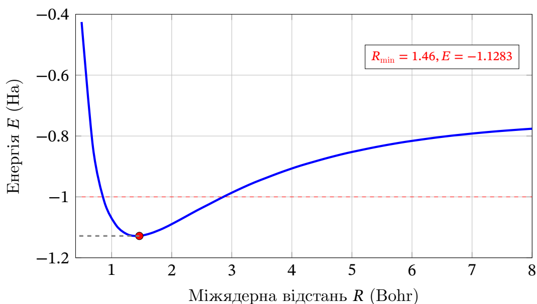
Рис. 4.3. Поверхня потенційної енергії молекули \text{H}_2 методом RHF.
