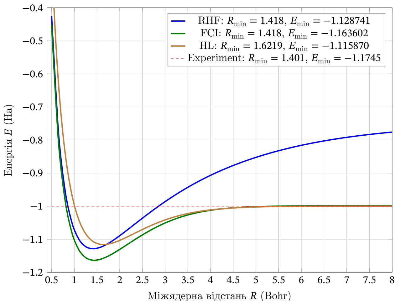
Рис. 4.4. Порівняння потенціальних енергетичних кривих молекули H_2 , отриманих методами RHF та FCI у базисному наборі cc-pVDZ . Для ілюстрації ковалентного також наведено криву, обчислену за теорією Гайтлера–Лондона.
