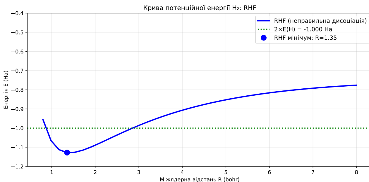
Рис. 2.2. Поверхня потенційна енергії молекули H_2 методом RHF. При великих R це означає:
