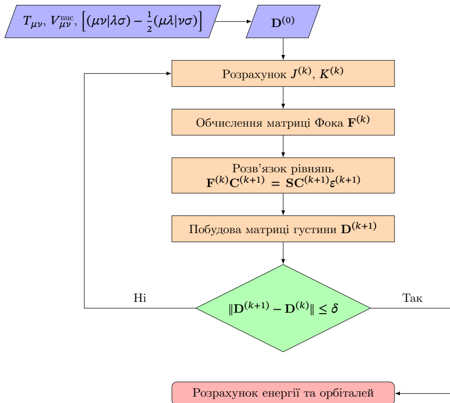
Рис. 1.1. Блок-схема SFC-процедури.
