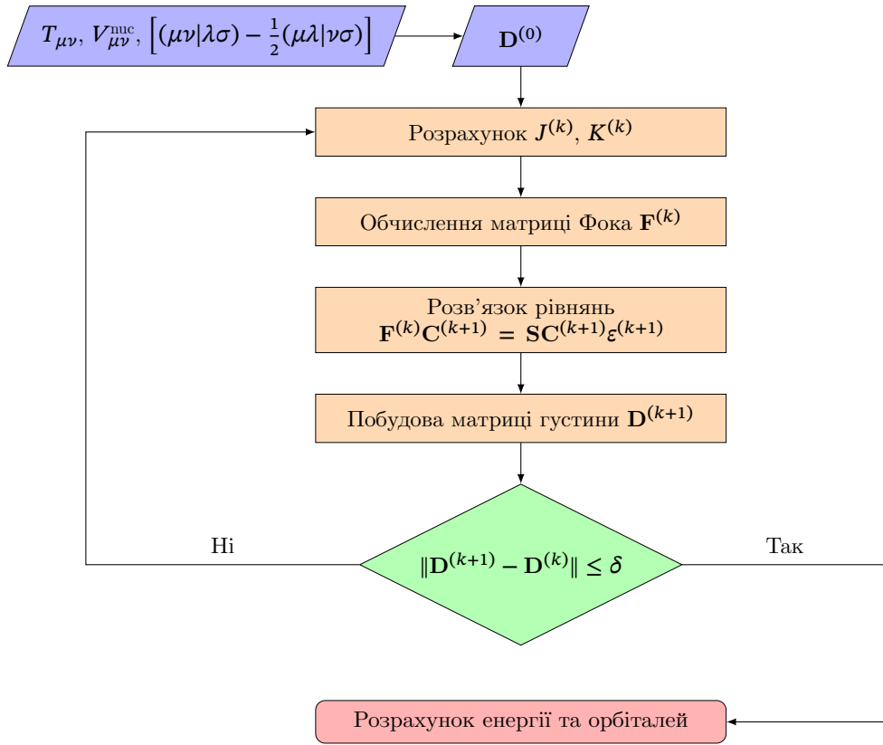
Рис. 3.1. Блок-схема SFC-процедури.
