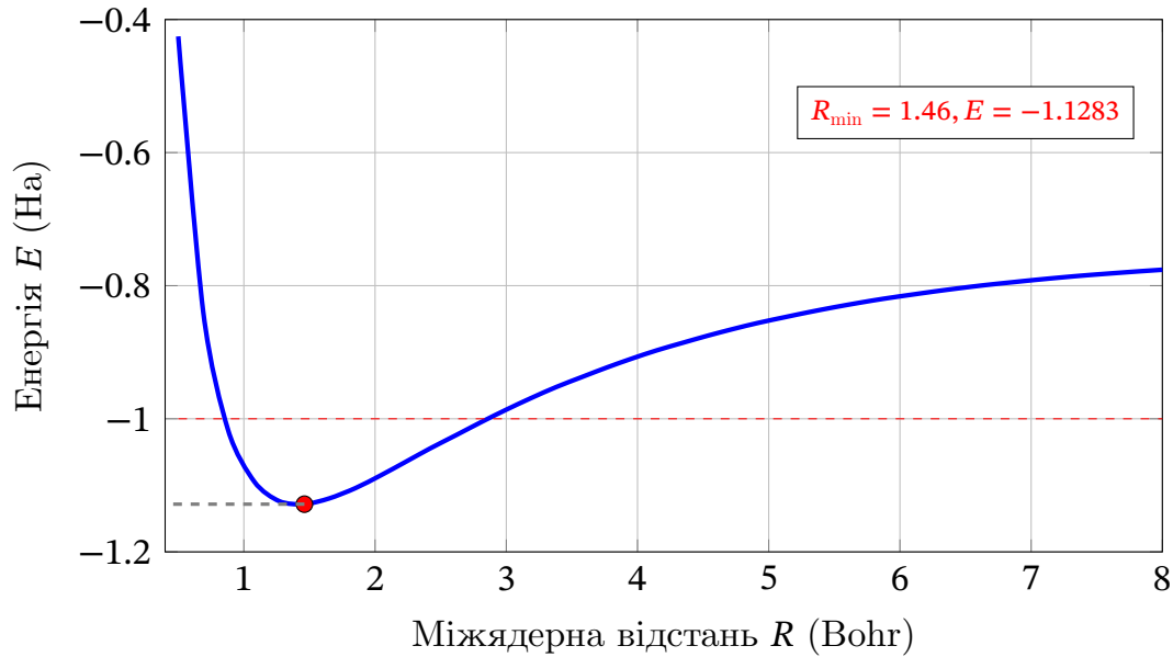
Рис. 4.7. Поверхня потенційної енергії молекули H_2 методом RHF.
