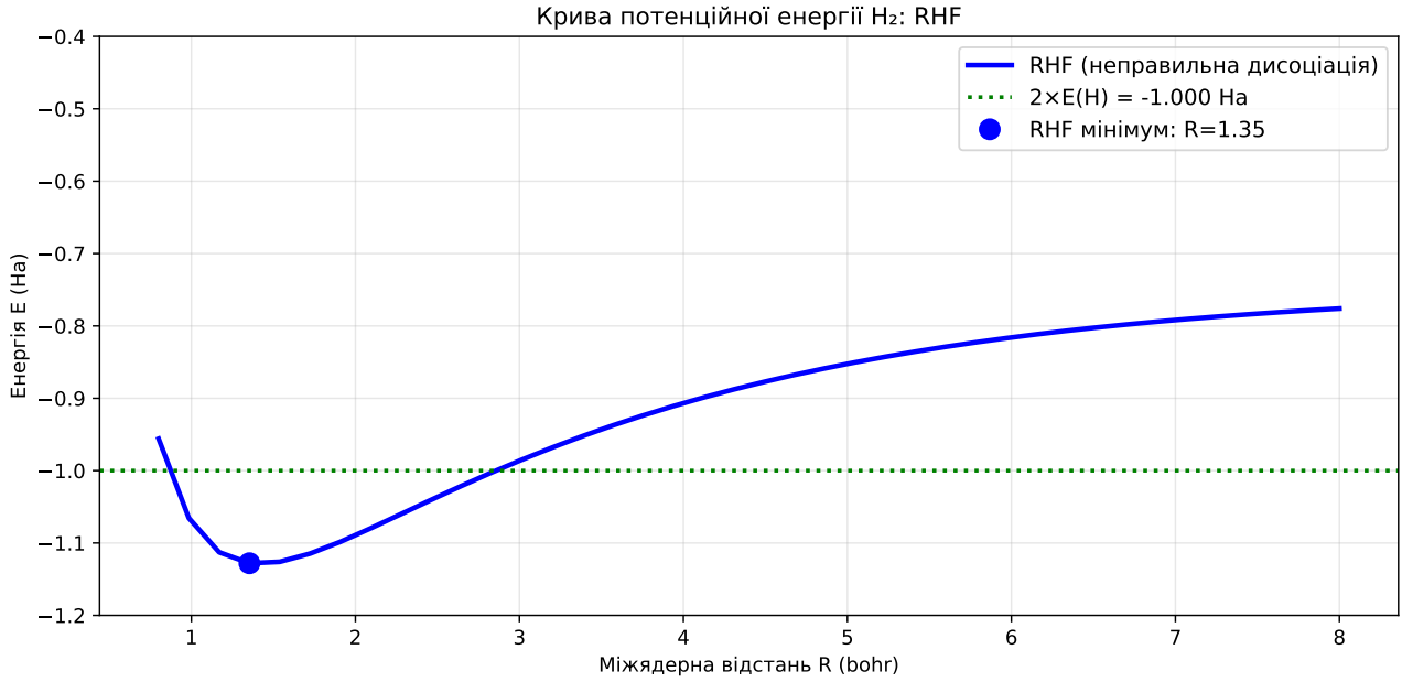
Рис. 4.3. Поверхня потенційної енергії молекули H_2 методом RHF. фізичної поведінки: енергія не прямує до суми енергій двох ізольованих атомів H.
