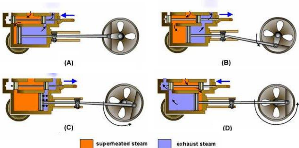
Рис. 2.14. Робота двотактної парової машини.
