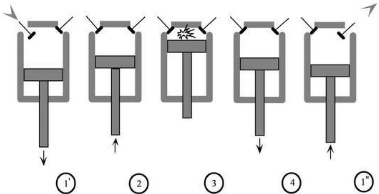
Рис. 2.17. Поршень і клапани в чотиритактному двигуні внутрішнього згорання
