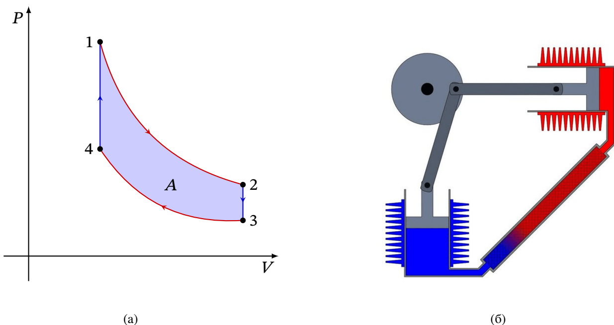
Рис. 2.19. Цикл (а) та Двигун (б) Стірлінга
