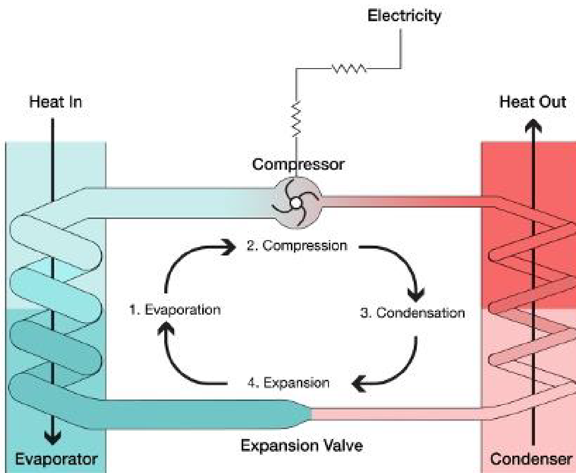
Рис. 2.9. Схема роботи теплового насоса
