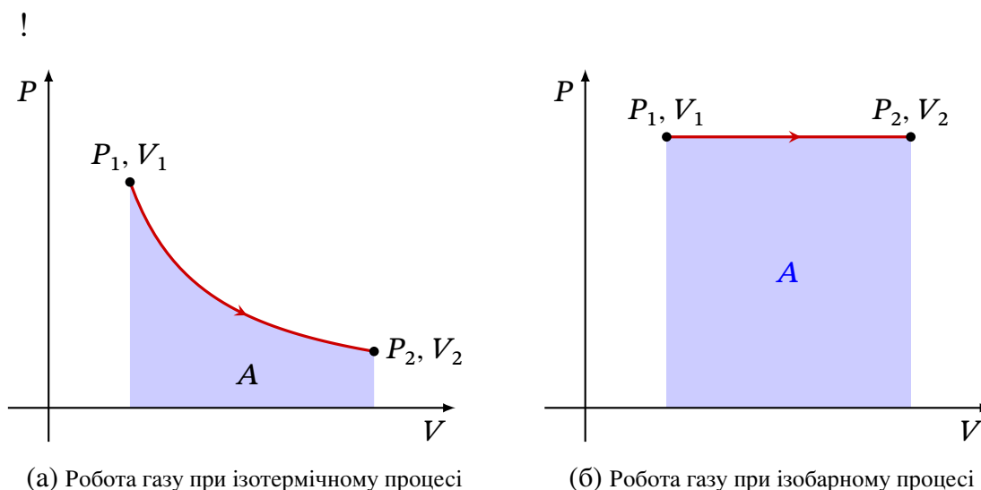
Рис. 1.4. Робота в газових процесах є площею під кривими
