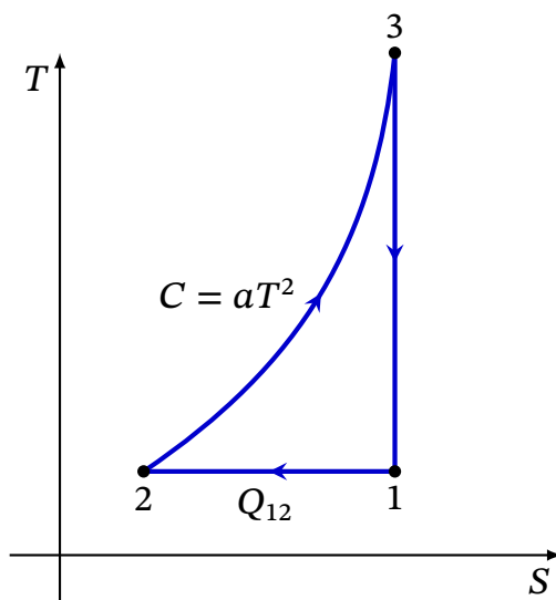
Рис. 3.6. Приклад обрахунку К.К.Д. циклу із використанням T - S діаграми.
