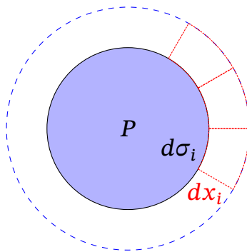
Рис. 1.13. Визначення елементарної роботи для гідро та газодинамічних систем
