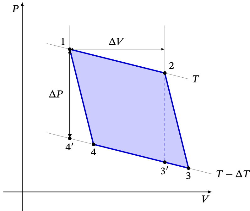
Рис. 3.4. Нескінченно малий цикл Карно на індикаторній діаграмі в довільній фізичній системі. де \Delta V може бути обрано малим, щоб диференціали можна було замінити приростом, а \left(\frac{\partial U}{\partial V}\right)_T і P вважати незмінними. З іншого боку робота в циклі, з точністю до малих вищого порядку, дорівнює площі паралелограма 123'4'
