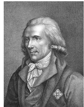
Граф Румфорд (1753 – 1814)
