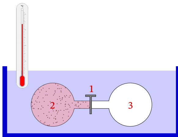
Рис. 2.4. Дослід Гей-Люсака по розширенню газу в вакуум. Після відкриття перегородки 1, газ із посудини ліворуч заповнює вакуумовану посудину праворуч, але температура навколишнього середовища не змінюється.
