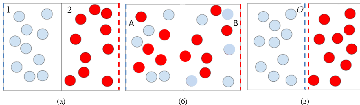
Рис. 3.12. До ілюстрації парадоксу Гібса: (а) два гази розділені теплопровідною перегородкою, (б) гази після змішування, (в) гази після розділення переміщенню до середини двохнапівпроникливих окремо для кожного з газів перегородок
