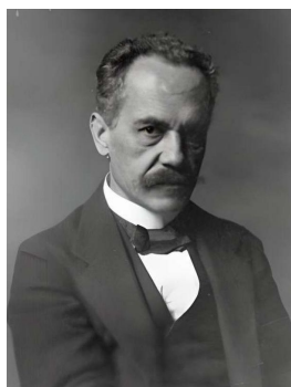
Арнольд Зоммерфельд (1868 – 1951)
