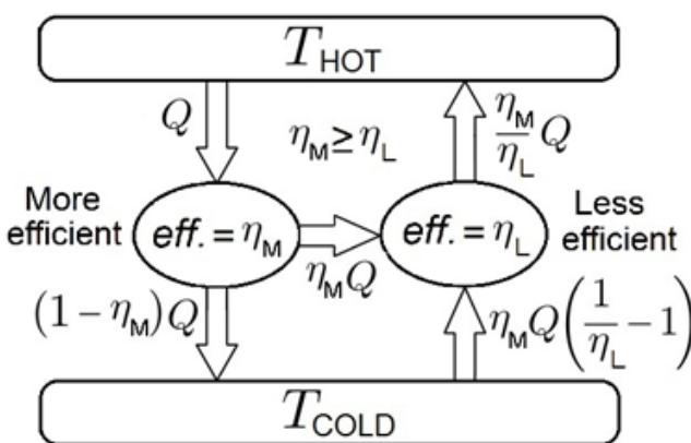
Рис. 1.1. Доведення першої теореми Карно
