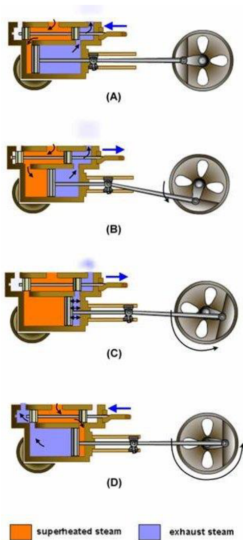
Рис. 1.2. Робота двотактної парової машини.
