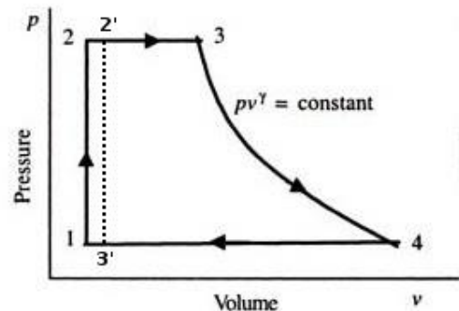
Рис. 1.1. Цикл Ранкіна роботи парової машини на діаграмі P, V .
