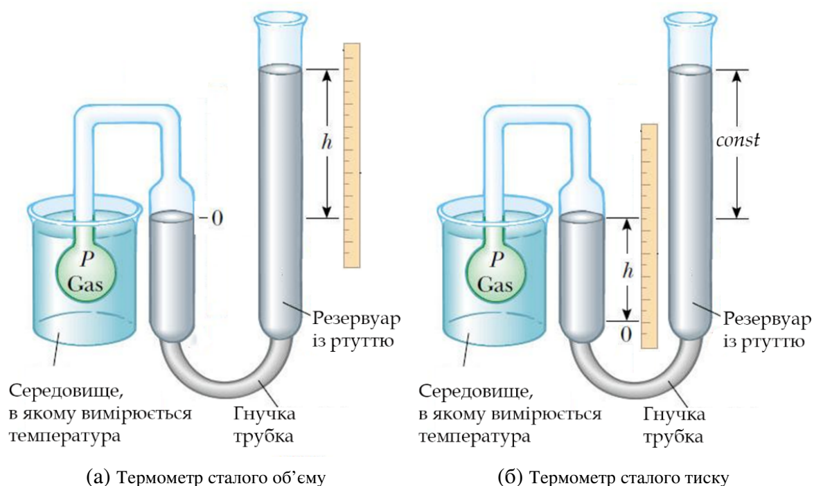
Рис. 1.7. Термометри сталого об'єму та тиску конструктивно принципово не відрізняються.
