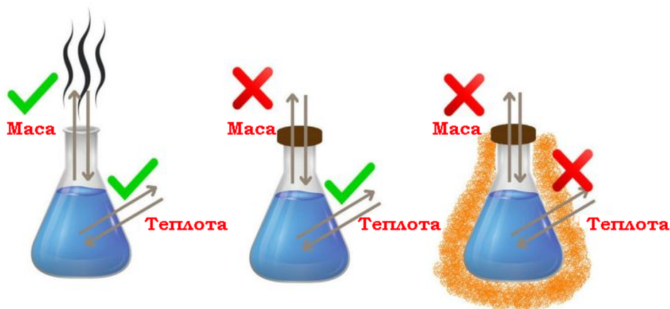
Рис. 1.2. Приклад відкритої, закритої та ізолюваної системи (зліва направо)
