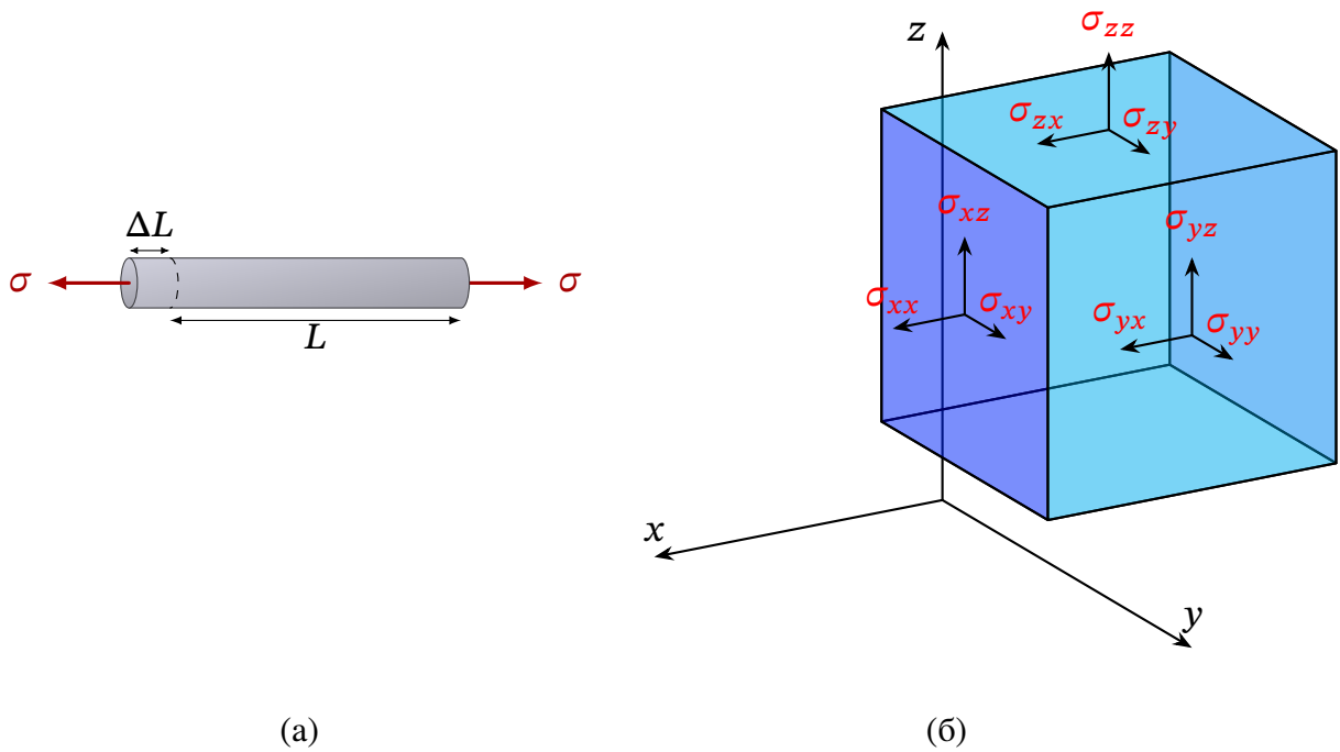
Рис. 1.12. До визначення елементарної роботи, що виконується над (а) гумовим жгутом та (б) твердим тілом
