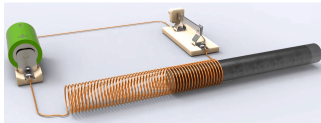
Рис. 1.13. До визначення елементарної роботи, що магнітним полем при намагнічуванні речовини
