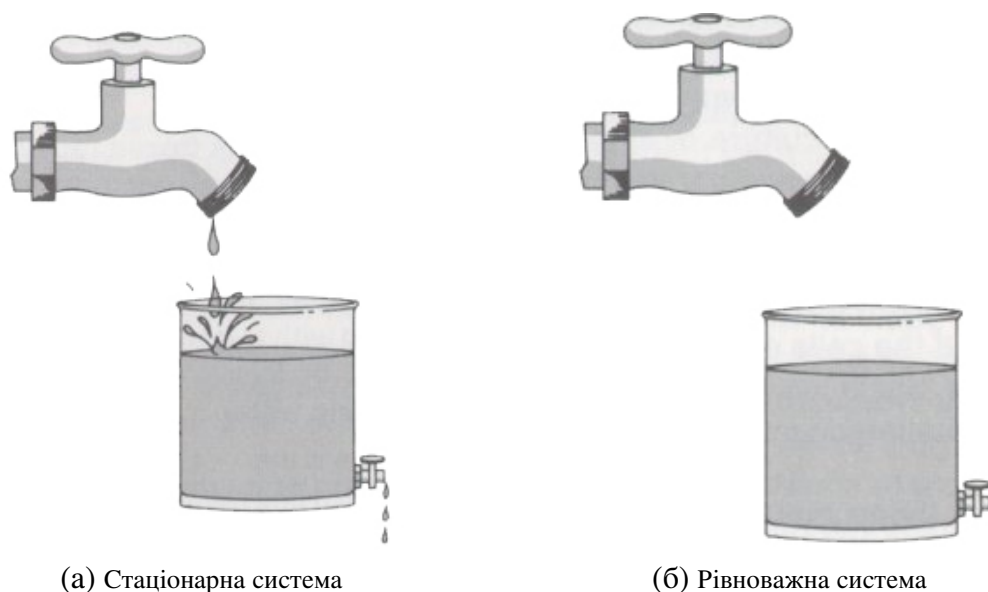
Рис. 1.3. Приклад стаціонарного (вода капає стаціонарним макроскопічним потоком) та рівноважного станів системи (немає макроскопічного потоку)
