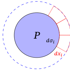
Рис. 1.10. Визначення елементарної роботи для гідро та газодинамічних систем
