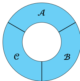
Рис. 1.4. Ілюстрація закону транзитивності теплової рівноваги
