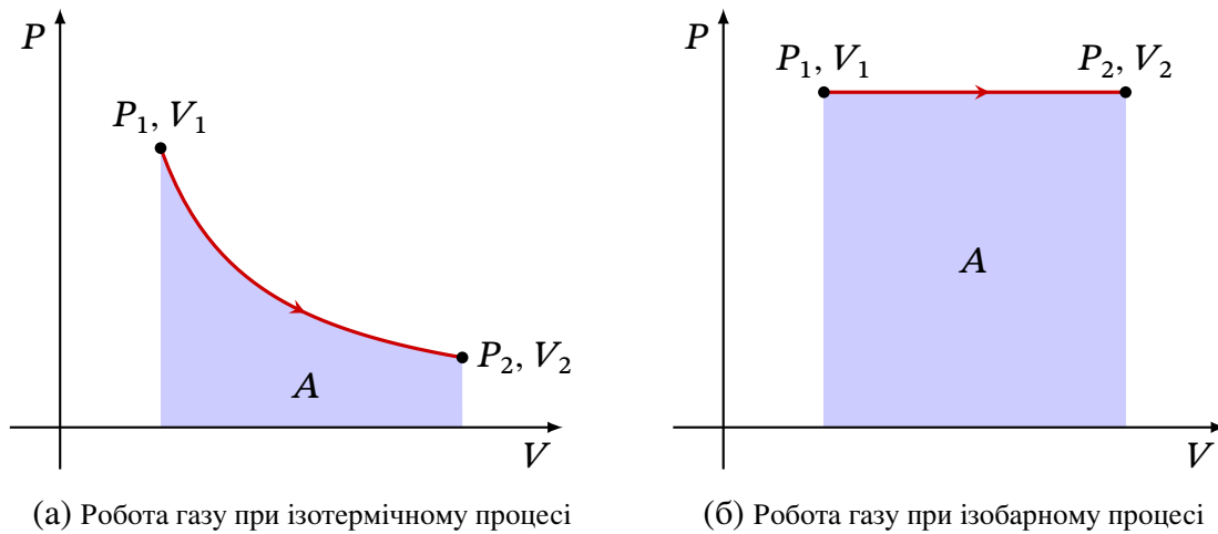
Рис. 1.11. Робота в газових процесах є площею під кривими
