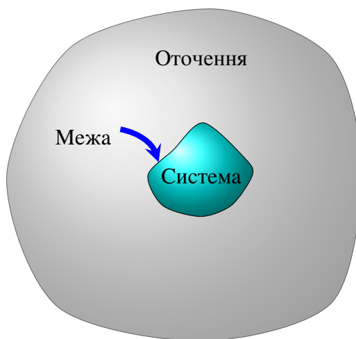
Рис. 1.1. Термодинамічна система і її оточення (термостат)
