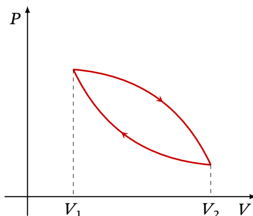
Рис. 1.9. Циклічний процес
