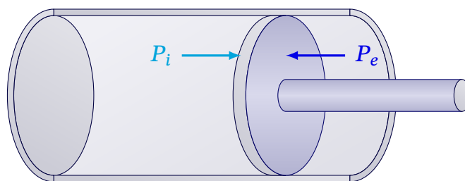
Рис. 1.8. Приведення в рух поршня вимагає незначного перебільшення зовнішнього тиску над тиском газу під поршнем
